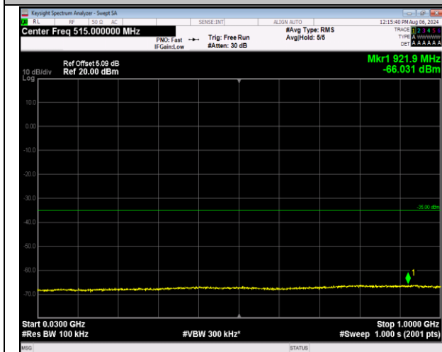
7-7-10MHz-20MHz-QPSK-QPSK-20805-20949-1RB#0-0 RB#0-30~1000MHz-PASS
