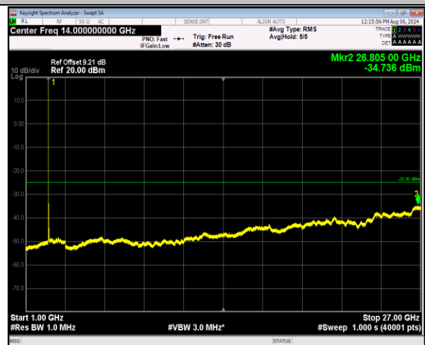
7-7-10MHz-20MHz-QPSK-QPSK-20805-20949-1RB#0-0RB #0-1000~27000MHz-PASS
