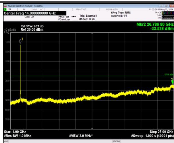
41-41-20MHz-10MHz-64QAM-64QAM-40571-40715-100RB #0-50RB#0-1000~27000MHz-PASS
