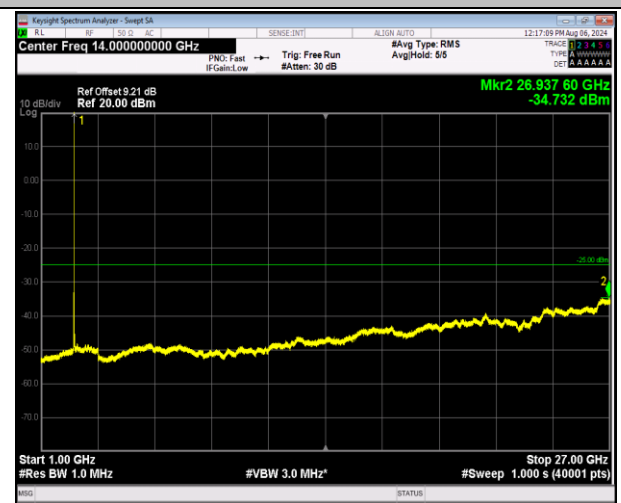
7-7-10MHz-20MHz-QPSK-QPSK-20805-20949-1RB#49-0R B#0-1000~27000MHz-PASS
