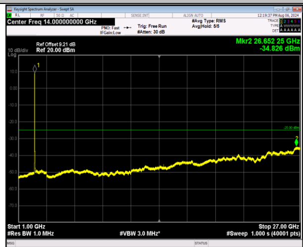
7-7-10MHz-20MHz-QPSK-QPSK-20805-20949-50RB#0-10 ORB#0-1000~27000MHz-PASS
