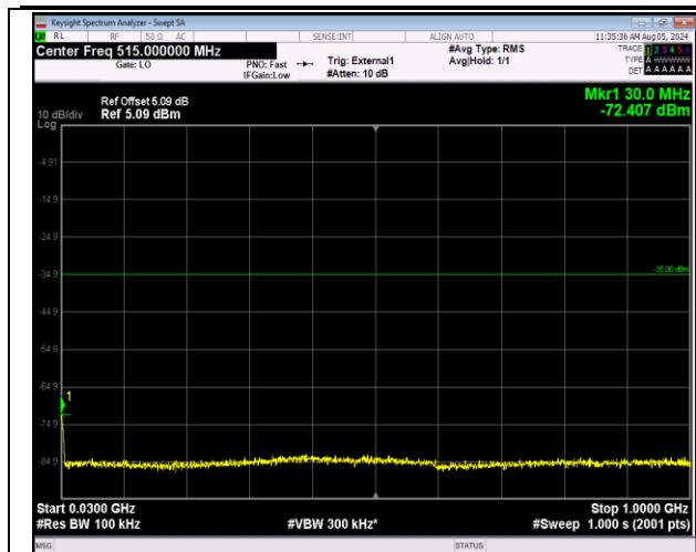
41-41-20MHz-10MHz-64QAM-64QAM-40571-40715-100 RB#0-50RB#0-30~1000MHz-PASS
