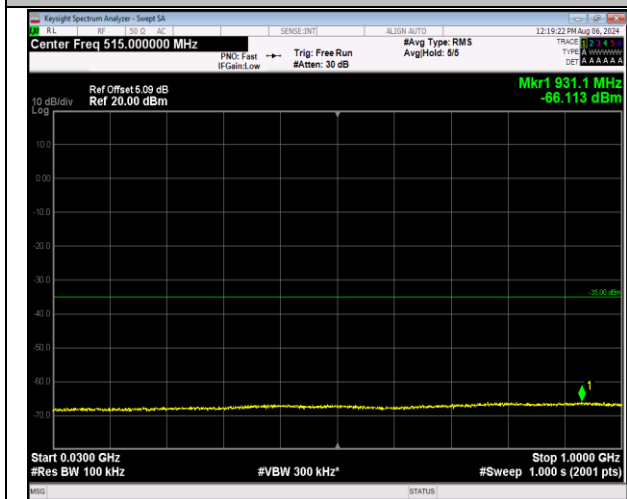
7-7-10MHz-20MHz-QPSK-QPSK-20805-20949-50RB#0-0 100RB#0-30~1000MHz-PASS
