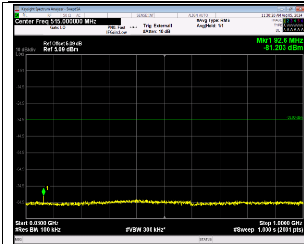
41-41-20MHz-10MHz-64QAM-64QAM-39750-39894-1RB #99-0RB#0-30~1000MHz-PASS
