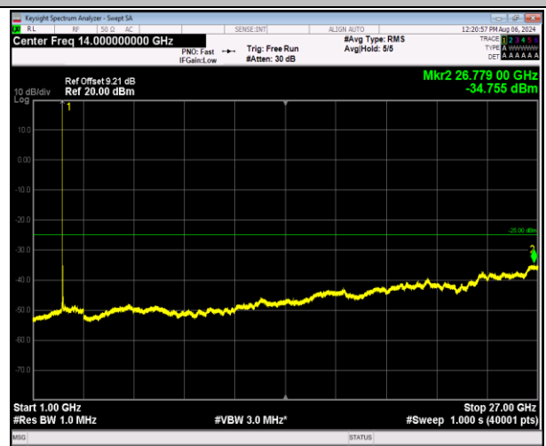
7-7-10MHz-20MHz-QPSK-QPSK-21006-21150-1RB#0-0RB #0-1000~27000MHz-PASS
