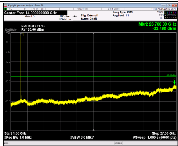
41-41-20MHz-10MHz-64QAM-64QAM-40571-40715-1RB#0 -ORB#0-1000~27000MHz-PASS
