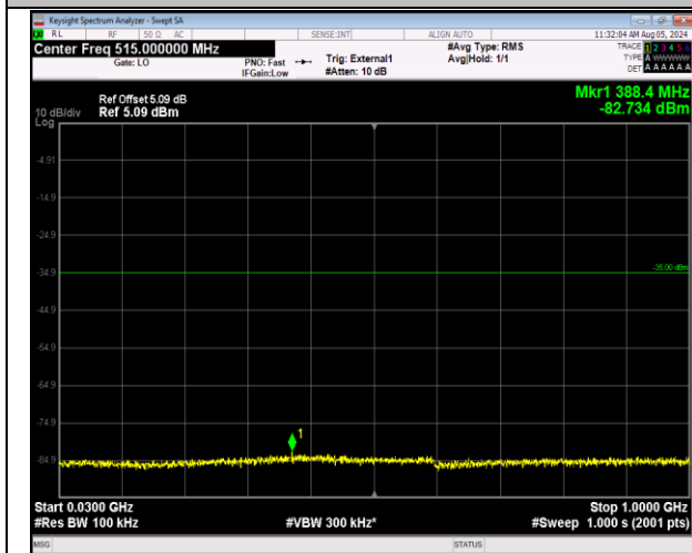
41-41-20MHz-10MHz-64QAM-64QAM-39750-39894-100 RB#0-50RB#0-30~1000MHz-PASS
