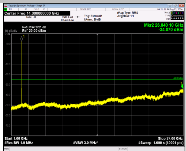
41-41-5MHz-20MHz-64QAM-64QAM-40528-40645-1RB#0- 1RB#99-1000~27000MHz-PASS
