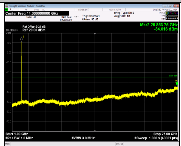
41-41-5MHz-20MHz-64QAM-64QAM-39683-39800-1RB#0- 1RB#99-1000~27000MHz-PASS
