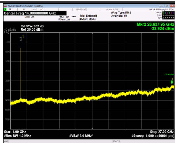
41-41-5MHz-20MHz-64QAM-64QAM-41373-41490-1RB#0- 1RB#99-1000~27000MHz-PASS
