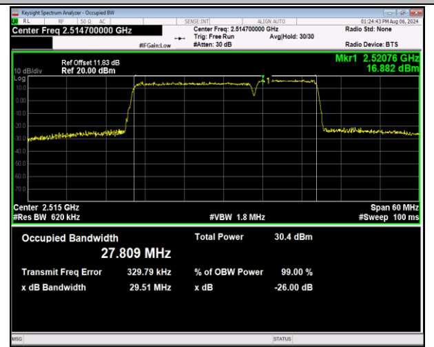
7-7-20MHz-10MHz-QPSK-QPSK-20850-20994-100RB#0- 50RB#0-PASS
