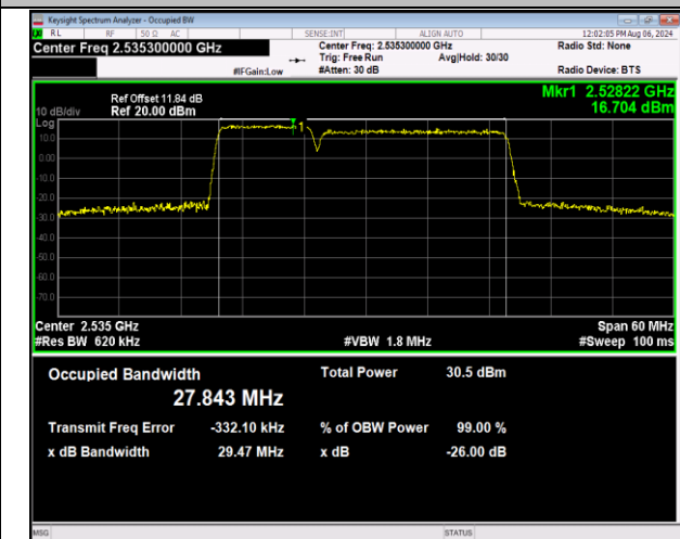
7-7-10MHz-20MHz-QPSK-QPSK-21006-21150-50RB#0-1 00RB#0-PASS
