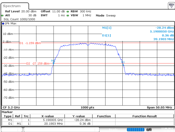
a_5200MHz_Chain 0
