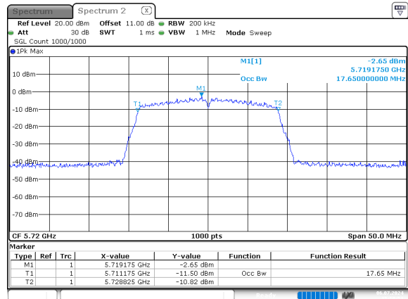
n20_5720MHz_Chain 0
