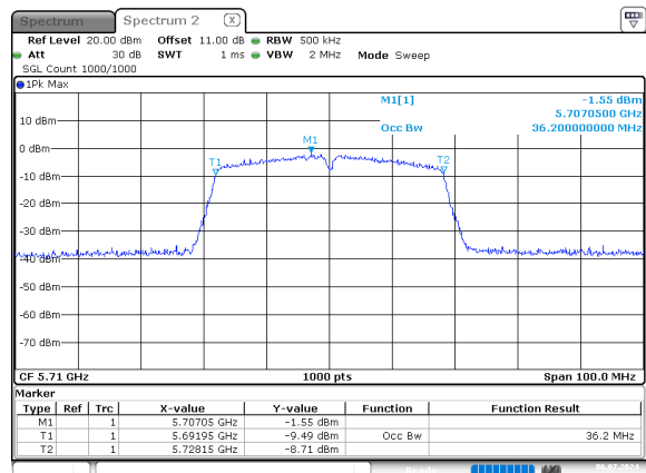
n40_5710MHz_Chain 0
