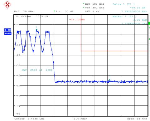
DH1_Hopping_Upper
