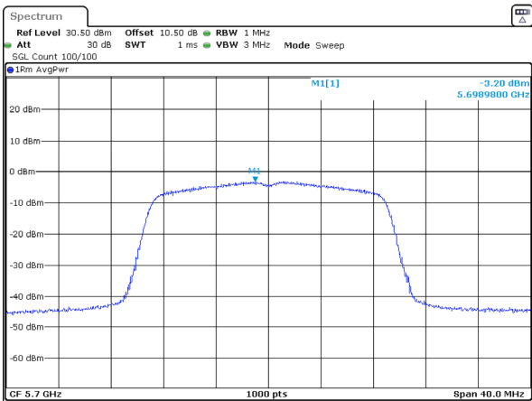
802.11ac20_5700MHz
