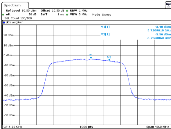
802.11ac20_5720MHz
