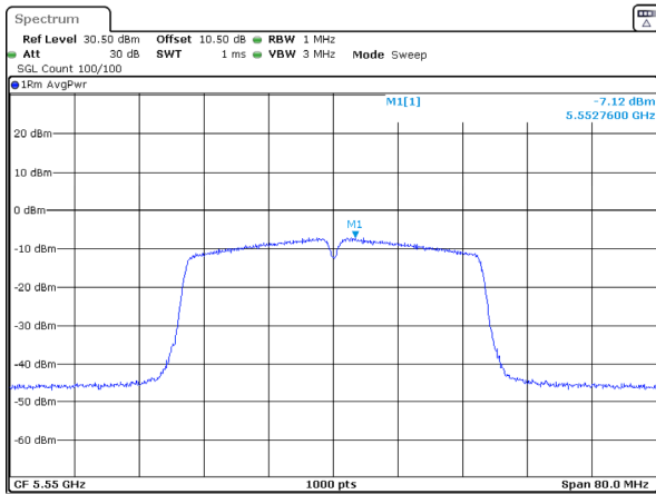
802.11ac40_5550MHz
