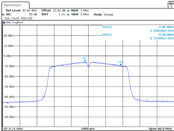
802.11ac40_5710MHz
