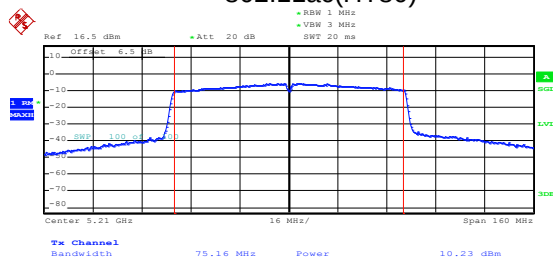
802.11ac(HT80)
