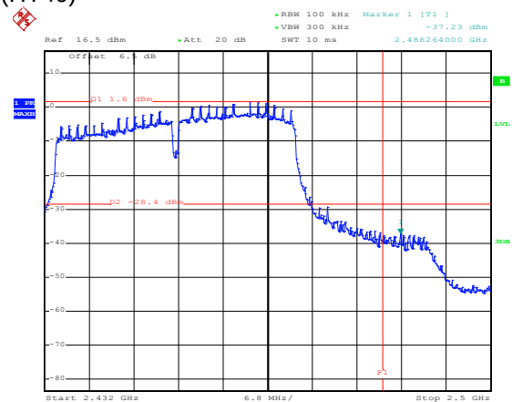
802.11n(HT40)
