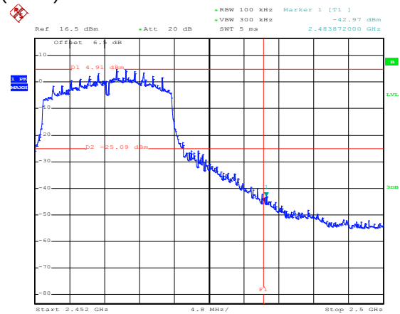
802.11n(HT20)
