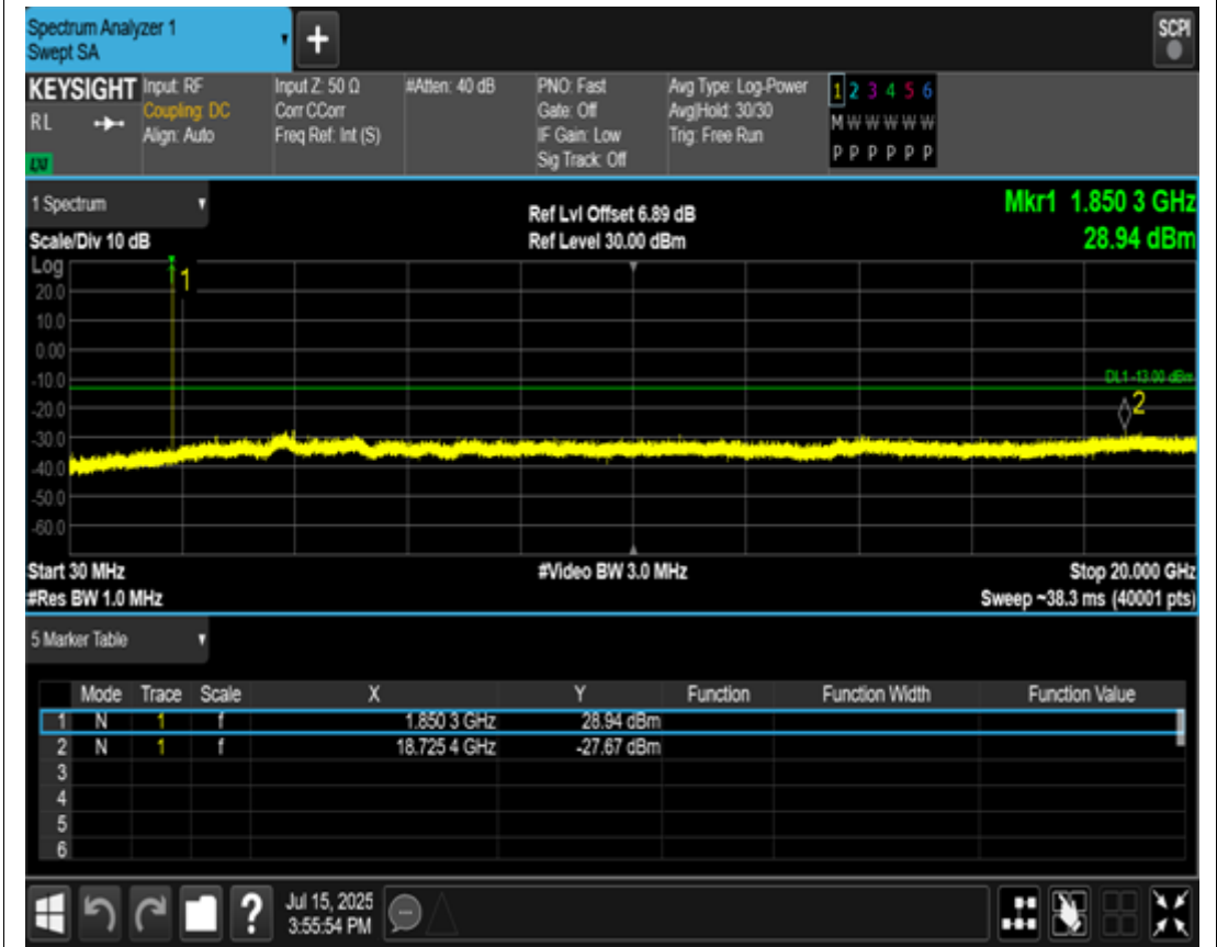
EGPRS1900 Channel=512
