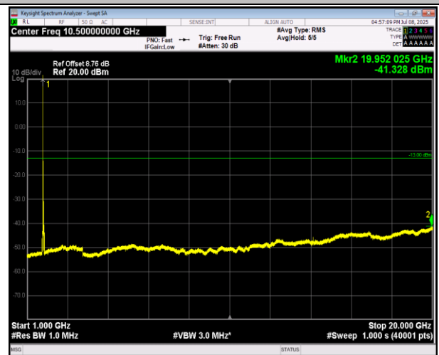
66-66-20MHz-20MHz-QPSK-QPSK-132374-132572-1RB#0-1RB#99-1000~20000MHz-PASS
