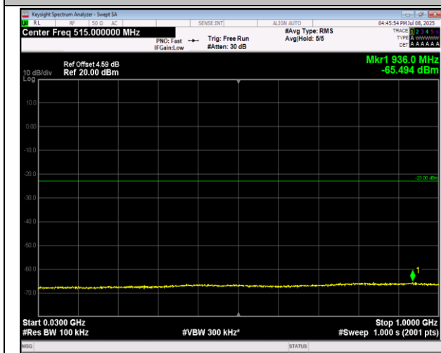
66-66-20MHz-20MHz-QPSK-QPSK-132072-132270-1RB #0-1RB#99-30~1000MHz-PASS
