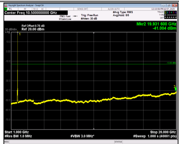
66-66-20MHz-5MHz-QPSK-QPSK-132397-132514-100RB# 0-25RB#0-1000~20000MHz-PASS
