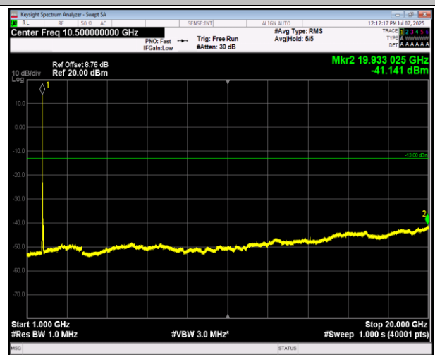
66-66-20MHz-5MHz-QPSK-QPSK-132397-132514-1RB#99 -0RB#0-1000~20000MHz-PASS
