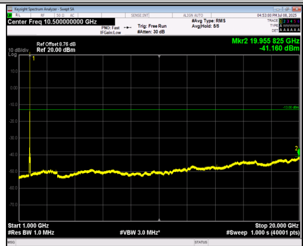
66-66-20MHz-20MHz-QPSK-QPSK-132323-132521-100RB #0-100RB#0-1000~20000MHz-PASS
