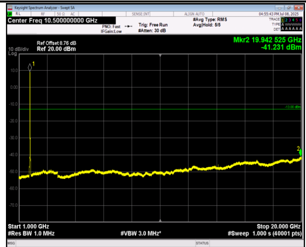
66-66-20MHz-20MHz-16QAM-16QAM-132323-132521-1R B#0-ORB#0-1000~20000MHz-PASS
