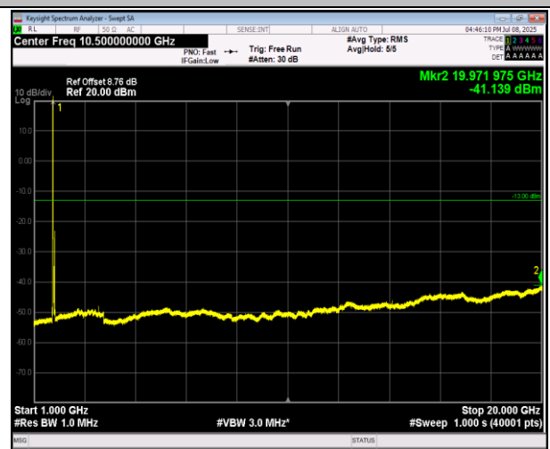
66-66-20MHz-20MHz-QPSK-QPSK-132072-132270-1RB#0 -1RB#99-1000~20000MHz-PASS
