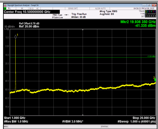
66-66-20MHz-20MHz-QPSK-QPSK-132374-132572-1RB#0-0RB#0-1000~20000MHz-PASS
