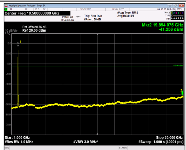
66-66-20MHz-20MHz-QPSK-QPSK-132323-132521-1RB#0 -ORB#0-1000~20000MHz-PASS
