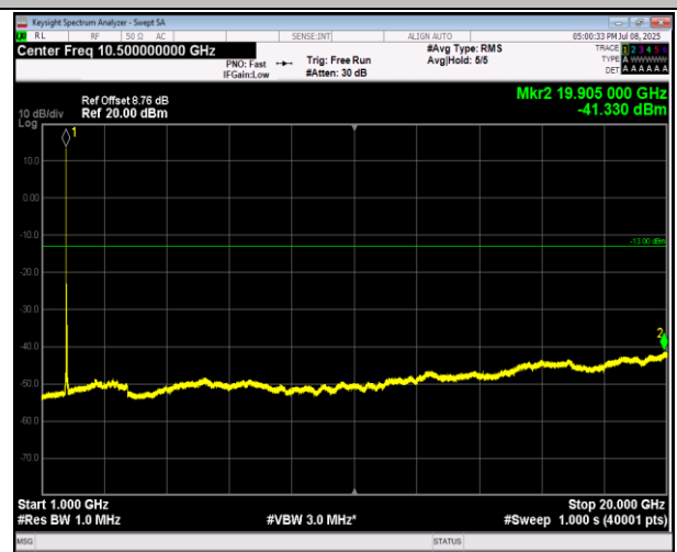
66-66-20MHz-20MHz-16QAM-16QAM-132374-132572-1R B#99-0RB#0-1000~20000MHz-PASS
