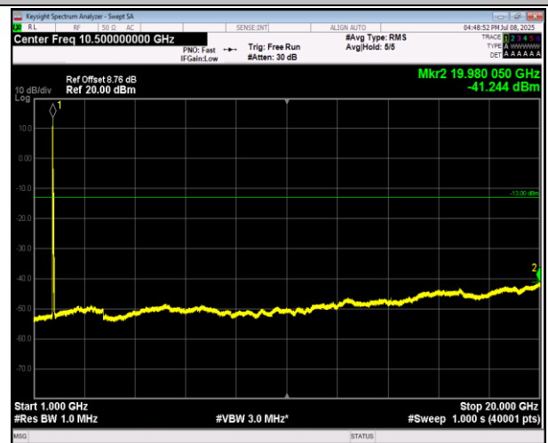
66-66-20MHz-20MHz-QPSK-QPSK-132072-132270-1RB#9 9-ORB#0-1000~20000MHz-PASS
