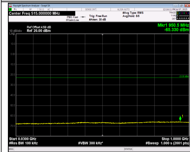
66-66-20MHz-5MHz-QPSK-QPSK-132522-132639-100R B#0-25RB#0-30~1000MHz-PASS
