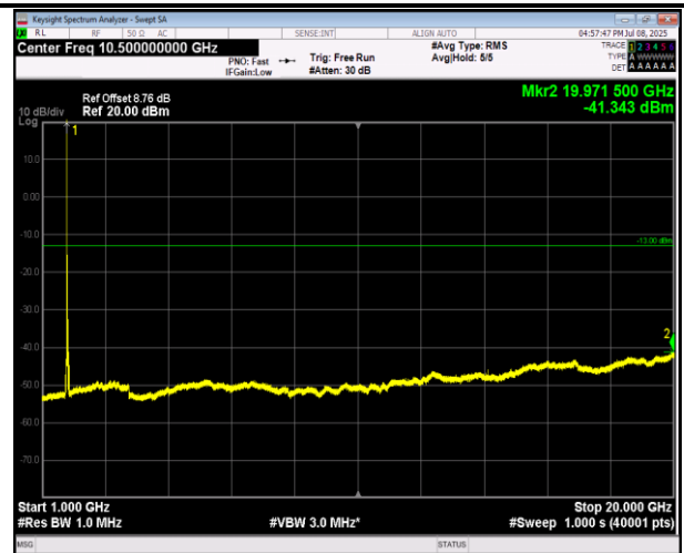
66-66-20MHz-20MHz-16QAM-16QAM-132374-132572-1R B#0-1RB#99-1000~20000MHz-PASS
