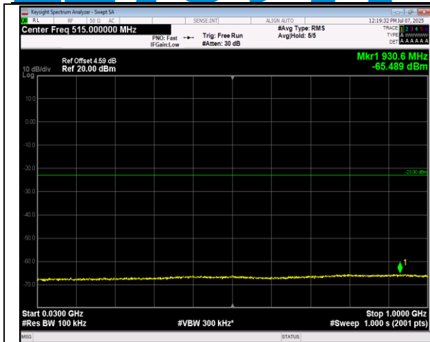
66-66-20MHz-20MHz-QPSK-QPSK-132072-132270-1RB #0-ORB#0-30~1000MHz-PASS
