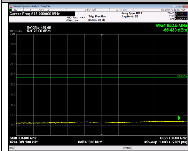
66-66-20MHz-20MHz-16QAM-16QAM-132323-132521-1 RB#0-1RB#99-30~1000MHz-PASS
