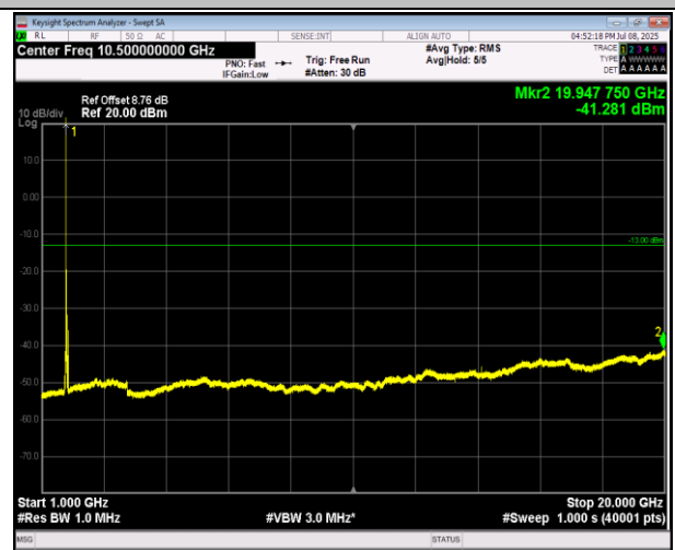
66-66-20MHz-20MHz-16QAM-16QAM-132323-132521-1R B#0-1RB#99-1000~20000MHz-PASS
