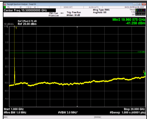
66-66-20MHz-20MHz-QPSK-QPSK-132323-132521-1RB#0 -1RB#99-1000~20000MHz-PASS
