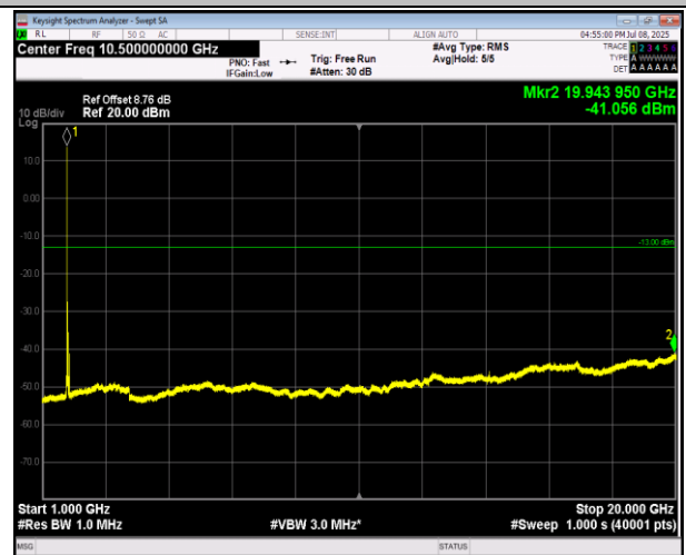
66-66-20MHz-20MHz-16QAM-16QAM-132323-132521-1R B#99-ORB#0-1000~20000MHz-PASS
