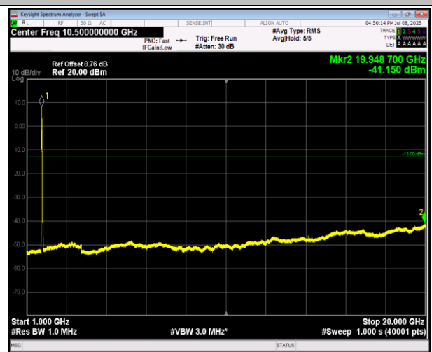
66-66-20MHz-20MHz-16QAM-16QAM-132072-132270-1R B#0-0RB#0-1000~20000MHz-PASS
