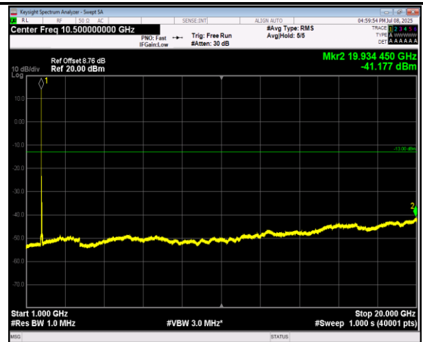
66-66-20MHz-20MHz-QPSK-QPSK-132374-132572-1RB#9 9-ORB#0-1000~20000MHz-PASS
