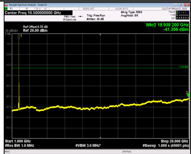
66-66-20MHz-5MHz-QPSK-QPSK-132522-132639-1RB#99 -ORB#0-1000~20000MHz-PASS
