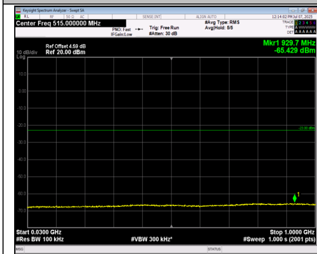
66-66-20MHz-5MHz-QPSK-QPSK-132522-132639-1RB# 0-0RB#0-30~1000MHz-PASS
