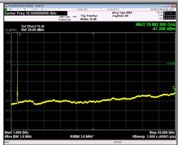
66-66-20MHz-20MHz-QPSK-QPSK-132374-132572-100RB #0-100RB#0-1000~20000MHz-PASS
