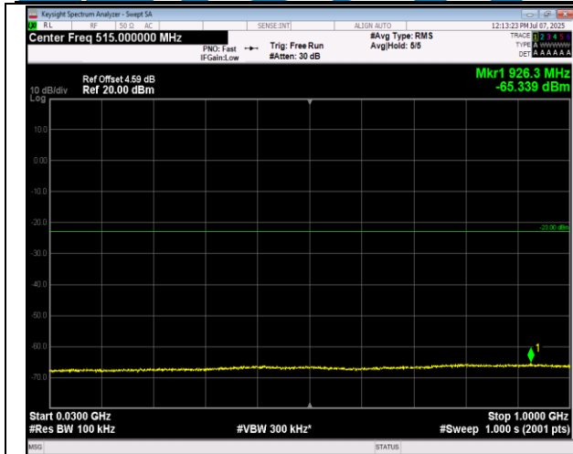
66-66-20MHz-5MHz-16QAM-16QAM-132397-132514-1R B#0-ORB#0-30~1000MHz-PASS
