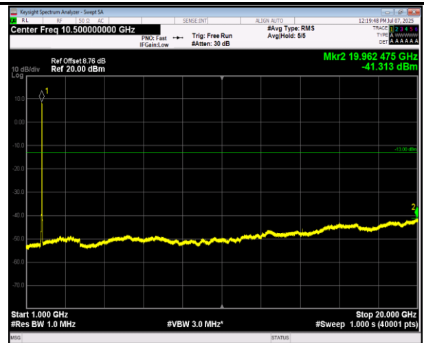
66-66-20MHz-20MHz-QPSK-QPSK-132072-132270-1RB#0 -ORB#0-1000~20000MHz-PASS
