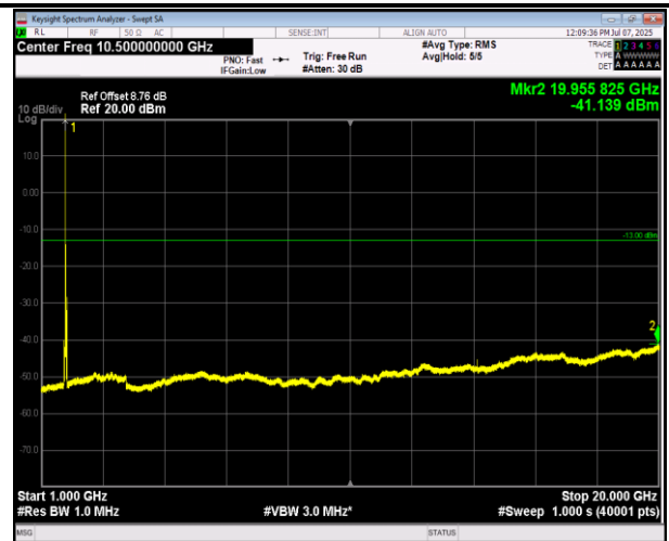
66-66-20MHz-5MHz-QPSK-QPSK-132397-132514-1RB#0- 1RB#24-1000~20000MHz-PASS
