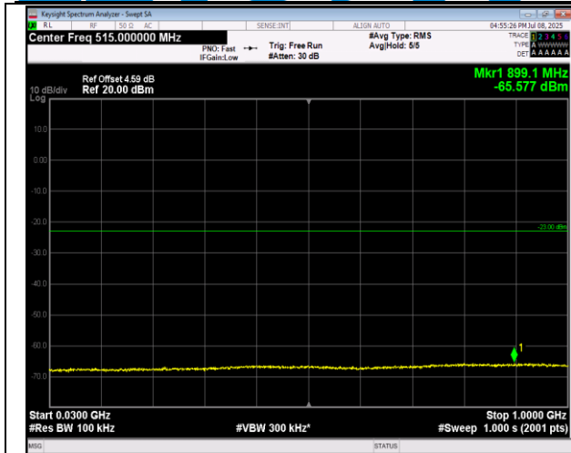
66-66-20MHz-20MHz-16QAM-16QAM-132323-132521-1 RB#0-ORB#0-30~1000MHz-PASS
