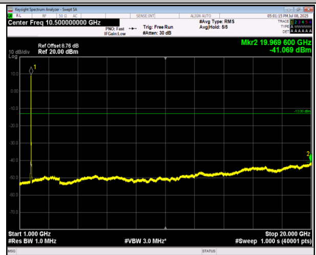
66-66-20MHz-20MHz-16QAM-16QAM-132374-132572-1R B#0-ORB#0-1000~20000MHz-PASS
