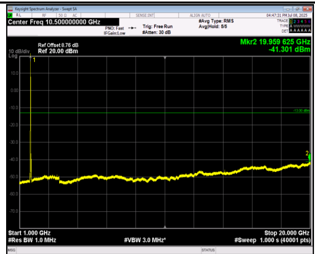
66-66-20MHz-20MHz-QPSK-QPSK-132072-132270-100RB #0-100RB#0-1000~20000MHz-PASS
