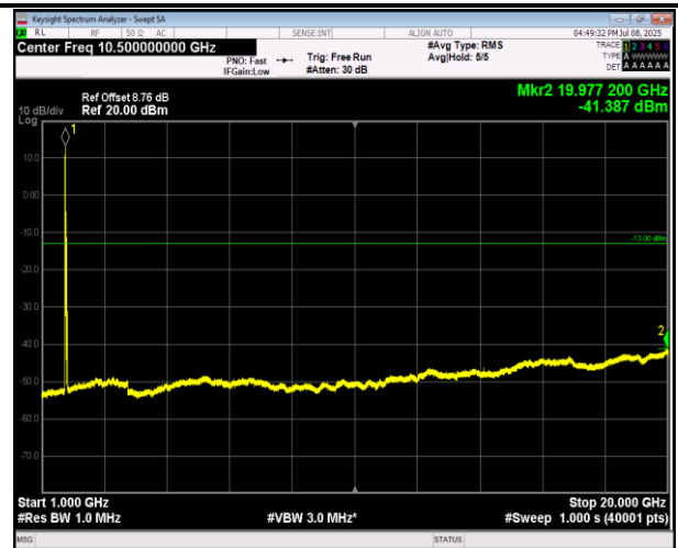
66-66-20MHz-20MHz-16QAM-16QAM-132072-132270-1R B#99-ORB#0-1000~20000MHz-PASS
