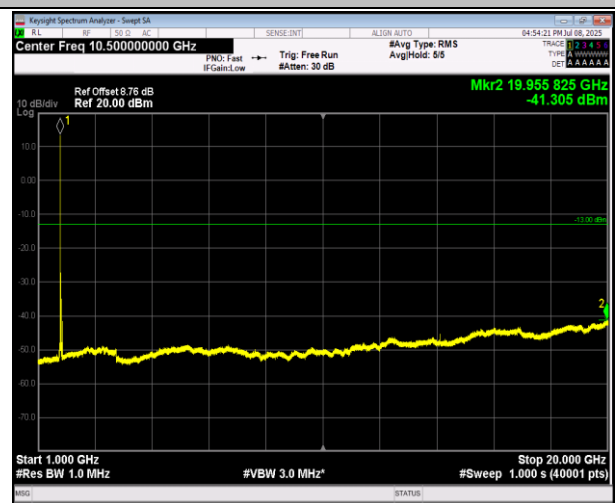
66-66-20MHz-20MHz-QPSK-QPSK-132323-132521-1RB#9 9-0RB#0-1000~20000MHz-PASS
