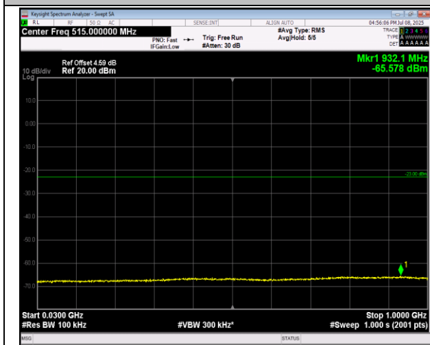
66-66-20MHz-20MHz-QPSK-QPSK-132374-132572-1RB#0-0RB#0-30~1000MHz-PASS
