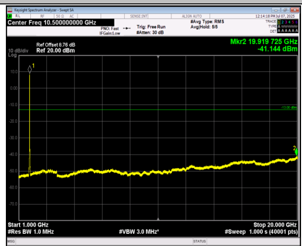
66-66-20MHz-5MHz-QPSK-QPSK-132522-132639-1RB#0- 0RB#0-1000~20000MHz-PASS
