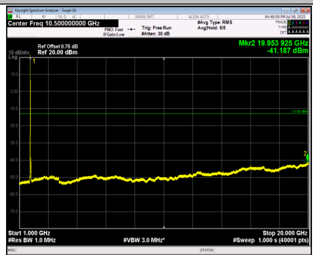
66-66-20MHz-20MHz-16QAM-16QAM-132072-132270-100 RB#0-100RB#0-1000~20000MHz-PASS
