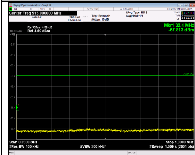
41(2555-2655)-41(2555-2655)-20MHz-5MHz-16QAM-16 QAM-40715-40832-1RB#99-0RB#0-30~1000MHz-PASS
