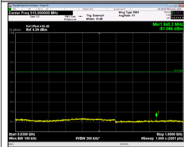
41(2555-2655)-41(2555-2655)-20MHz-5MHz-QPSK-QPS K-40340-40457-1RB#0-1RB#24-30~1000MHz-PASS
