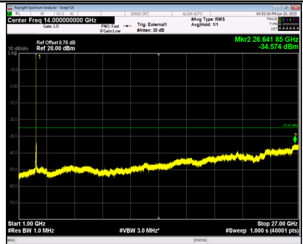
41(2555-2655)-41(2555-2655)-15MHz-20MHz-QPSK-QPS K-40644-40815-1RB#0-1RB#99-1000~27000MHz-PASS
