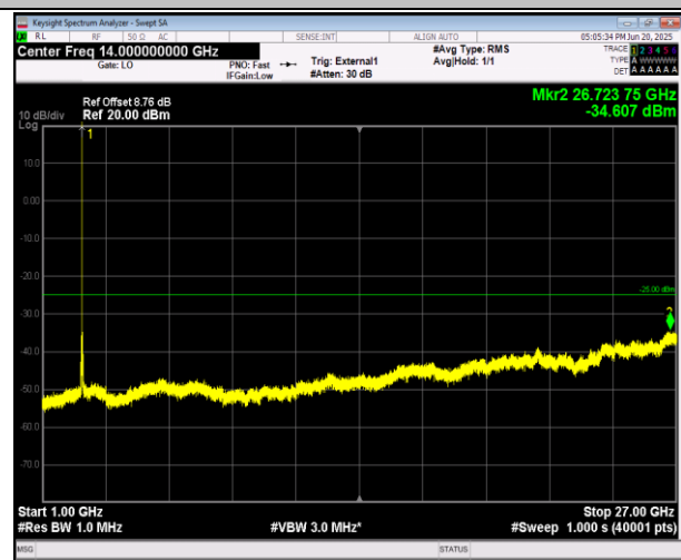
41(2555-2655)-41(2555-2655)-15MHz-20MHz-QPSK-QPS K-40969-41140-75RB#0-100RB#0-1000~27000MHz-PASS
