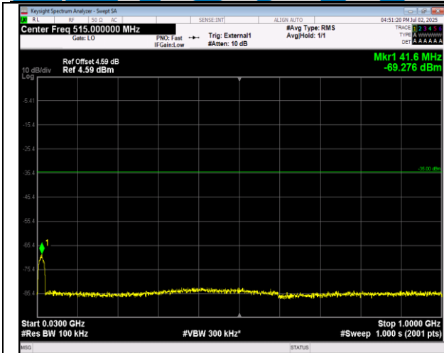
41(2555-2655)-41(2555-2655)-20MHz-5MHz-16QAM-16 QAM-40715-40832-1RB#0-0RB#0-30~1000MHz-PASS
