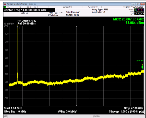
41(2555-2655)-41(2555-2655)-15MHz-20MHz-QPSK-QPS K-40644-40815-75RB#0-100RB#0-1000~27000MHz-PASS
