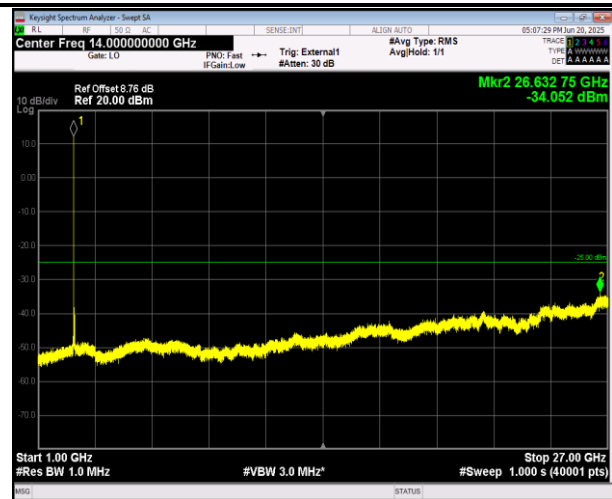
41(2555-2655)-41(2555-2655)-15MHz-20MHz-QPSK-QPS K-40969-41140-1RB#74-ORB#0-1000~27000MHz-PASS
