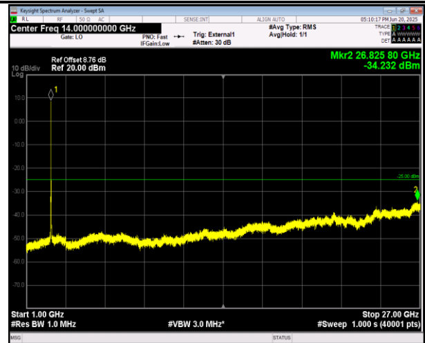
41(2555-2655)-41(2555-2655)-20MHz-5MHz-QPSK-QPSK- 40340-40457-1RB#0-ORB#0-1000~27000MHz-PASS
