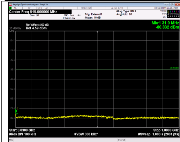
41(2555-2655)-41(2555-2655)-15MHz-20MHz-QPSK-QP SK-40644-40815-1RB#0-1RB#99-30~1000MHz-PASS
