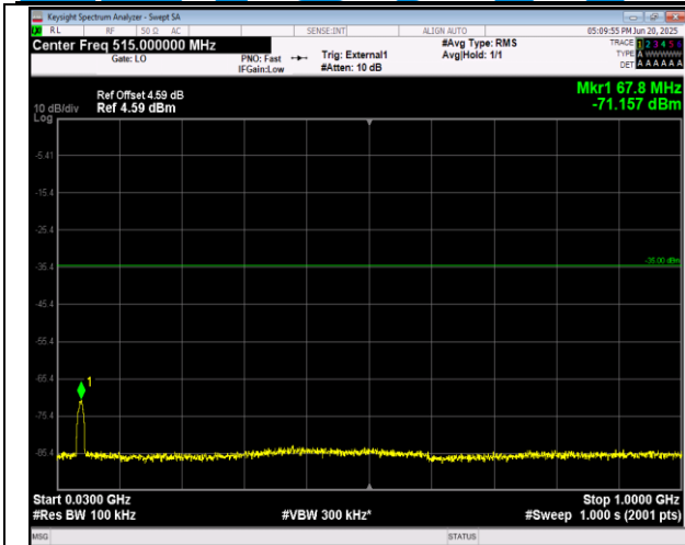
41(2555-2655)-41(2555-2655)-20MHz-5MHz-QPSK-QPS K-40340-40457-1RB#0-ORB#0-30~1000MHz-PASS
