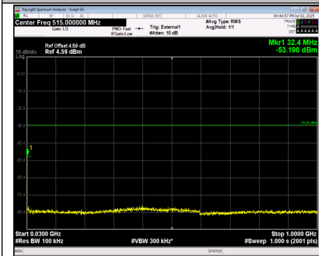
41(2555-2655)-41(2555-2655)-20MHz-5MHz-16QAM-16 QAM-40715-40832-1RB#0-1RB#24-30~1000MHz-PASS
