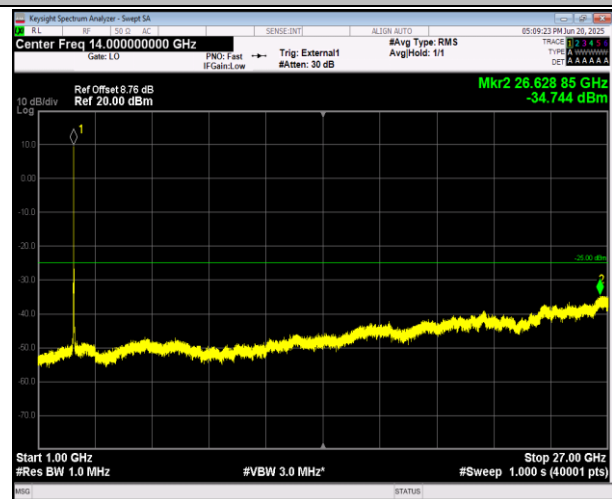
41(2555-2655)-41(2555-2655)-15MHz-20MHz-16QAM-16 AM-40969-41140-1RB#0-ORB#0-1000~27000MHz-PASS
