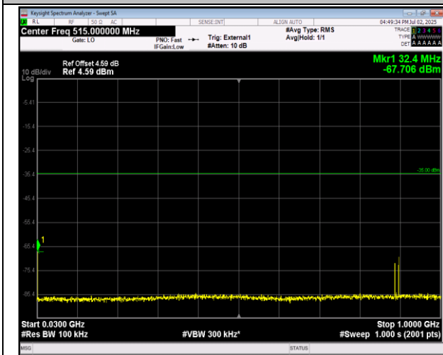
41(2555-2655)-41(2555-2655)-20MHz-5MHz-QPSK-QPS K-40715-40832-1RB#99-0RB#0-30~1000MHz-PASS
