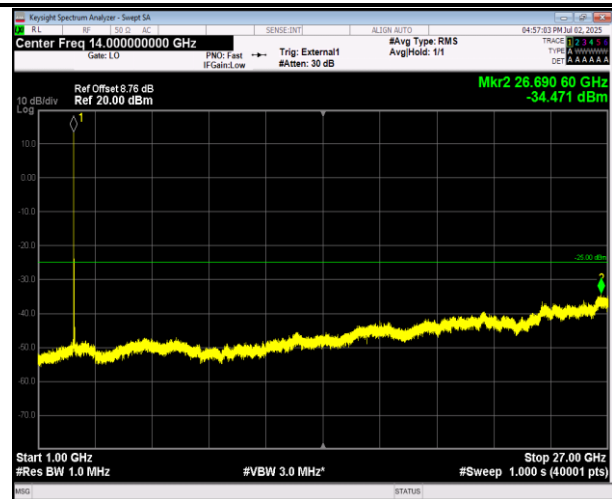
41(2555-2655)-41(2555-2655)-20MHz-5MHz-QPSK-QPSK- 41090-41207-1RB#99-0RB#0-1000~27000MHz-PASS
