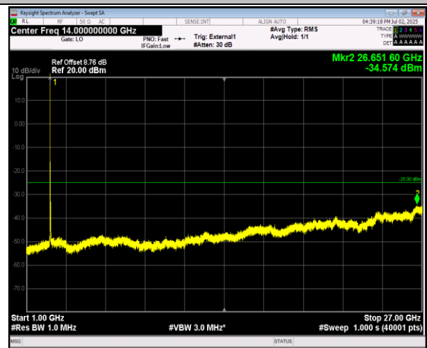
41(2555-2655)-41(2555-2655)-20MHz-5MHz-QPSK-QPSK- 40340-40457-1RB#0-1RB#24-1000~27000MHz-PASS
