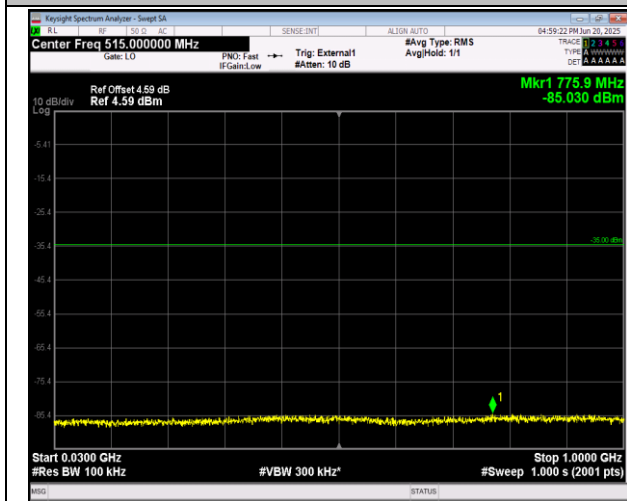
41(2555-2655)-41(2555-2655)-15MHz-20MHz-QPSK-QP SK-40644-40815-1RB#74-0RB#0-30~1000MHz-PASS
