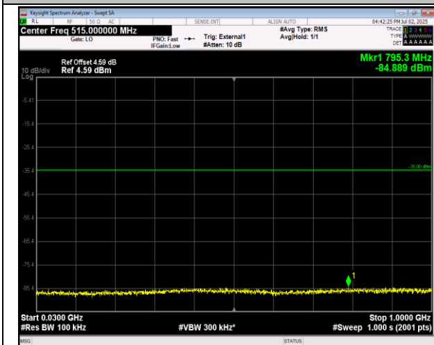
41(2555-2655)-41(2555-2655)-20MHz-5MHz-QPSK-QPS K-40340-40457-1RB#99-ORB#0-30~1000MHz-PASS
