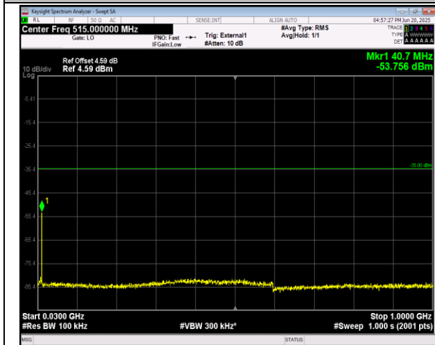
41(2555-2655)-41(2555-2655)-15MHz-20MHz-QPSK-QP SK-40644-40815-75RB#0-100RB#0-30~1000MHz-PASS
