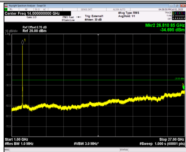
41(2555-2655)-41(2555-2655)-20MHz-5MHz-16QAM-16QA M-41090-41207-1RB#0-0RB#0-1000~27000MHz-PASS
