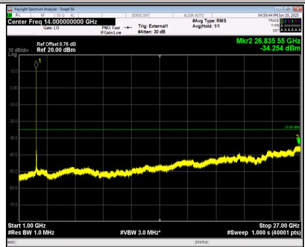
41(2555-2655)-41(2555-2655)-15MHz-20MHz-QPSK-QPS K-40644-40815-1RB#74-0RB#0-1000~27000MHz-PASS
