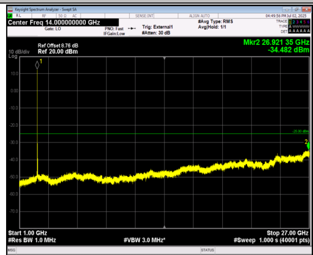
41(2555-2655)-41(2555-2655)-20MHz-5MHz-QPSK-QPSK- 40715-40832-1RB#99-0RB#0-1000~27000MHz-PASS
