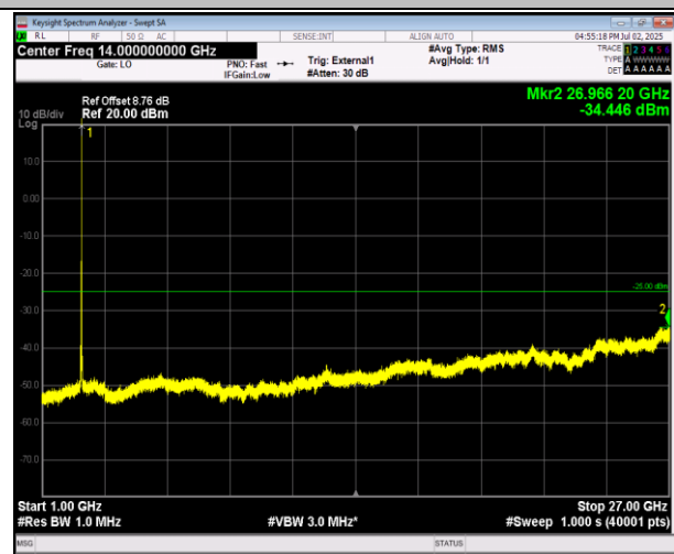
41(2555-2655)-41(2555-2655)-20MHz-5MHz-QPSK-QPSK- 41090-41207-100RB#0-25RB#0-1000~27000MHz-PASS
