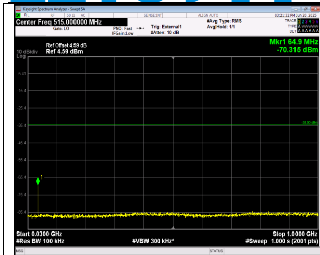
41(2555-2655)-41(2555-2655)-15MHz-15MHz-QPSK-QP SK-41015-41165-1RB#74-ORB#0-30~1000MHz-PASS
