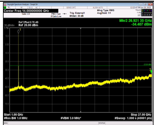
41(2555-2655)-41(2555-2655)-15MHz-10MHz-QPSK-QPS K-41067-41187-1RB#74-ORB#0-1000~27000MHz-PASS
