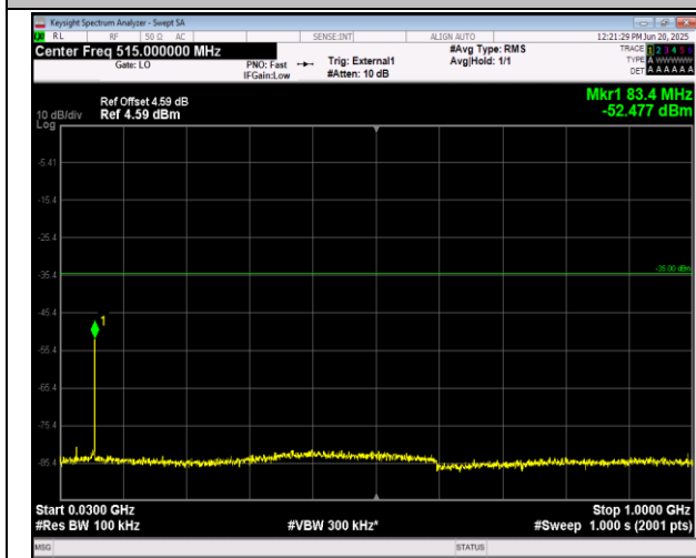
41(2555-2655)-41(2555-2655)-15MHz-10MHz-QPSK-QP SK-41067-41187-75RB#0-50RB#0-30~1000MHz-PASS
