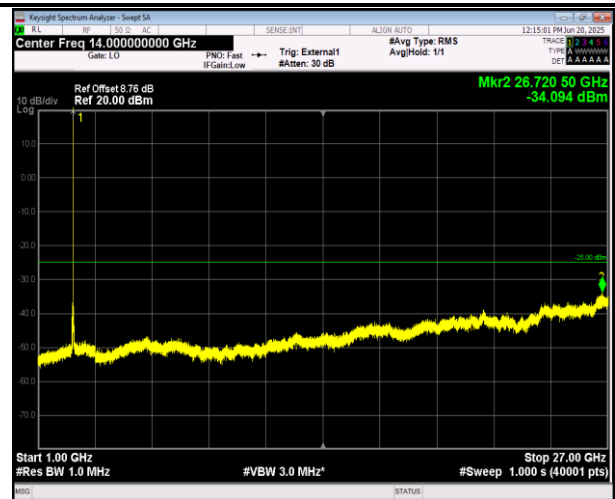
41(2555-2655)-41(2555-2655)-15MHz-10MHz-16QAM-16 QAM-40691-40811-75RB#0-50RB#0-1000~27000MHz-PASS
