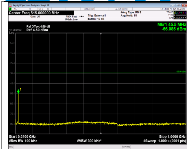
41(2555-2655)-41(2555-2655)-15MHz-10MHz-16QAM-16 QAM-40691-40811-75RB#0-50RB#0-30~1000MHz-PASS
