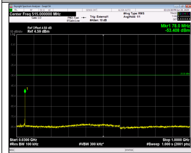
41(2555-2655)-41(2555-2655)-15MHz-15MHz-QPSK-QP SK-41015-41165-75RB#0-75RB#0-30~1000MHz-PASS
