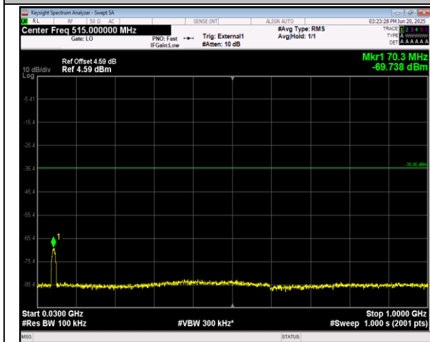
41(2555-2655)-41(2555-2655)-15MHz-15MHz-16QAM-16 QAM-41015-41165-1RB#0-ORB#0-30~1000MHz-PASS
