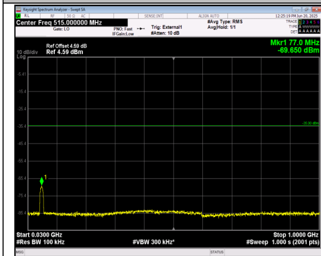
41(2555-2655)-41(2555-2655)-15MHz-10MHz-16QAM-16 QAM-41067-41187-1RB#0-ORB#0-30~1000MHz-PASS
