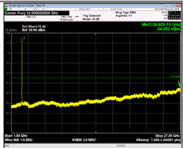
41(2555-2655)-41(2555-2655)-15MHz-15MHz-16QAM-16Q AM-41015-41165-1RB#0-ORB#0-1000~27000MHz-PASS
