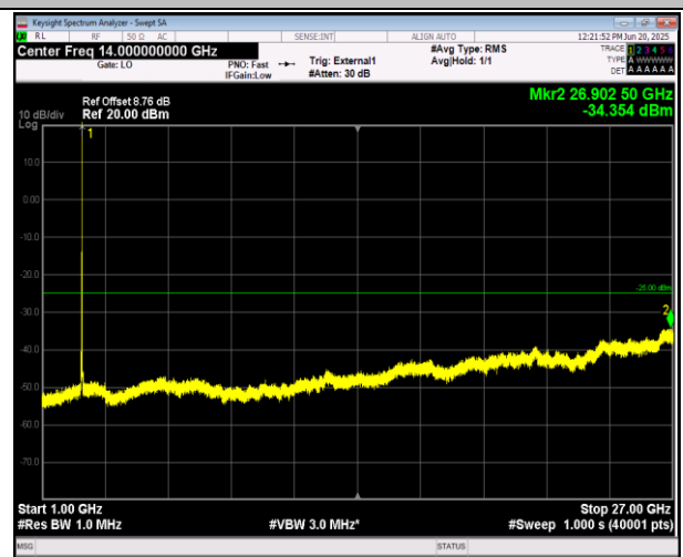
41(2555-2655)-41(2555-2655)-15MHz-10MHz-QPSK-QPS K-41067-41187-75RB#0-50RB#0-1000~27000MHz-PASS
