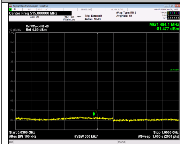
41(2555-2655)-41(2555-2655)-15MHz-20MHz-QPSK-QP SK-40318-40489-1RB#0-1RB#99-30~1000MHz-PASS
