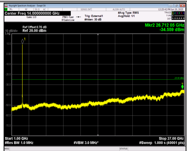
41(2555-2655)-41(2555-2655)-15MHz-10MHz-16QAM-16 AM-41067-41187-1RB#0-ORB#0-1000~27000MHz-PASS
