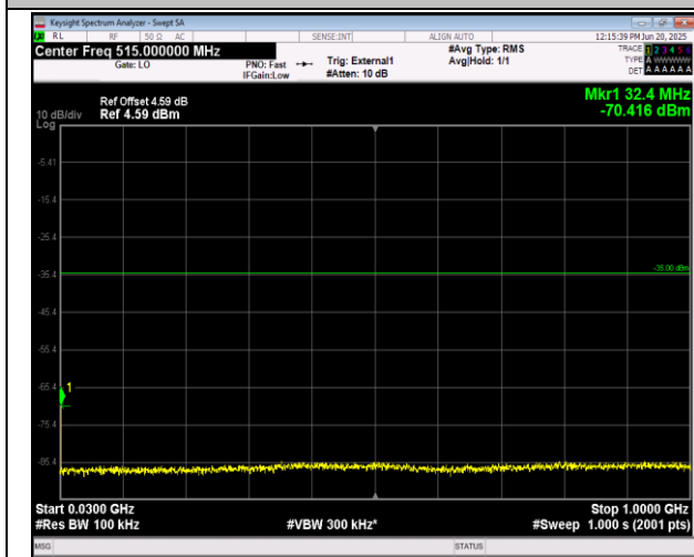
41(2555-2655)-41(2555-2655)-15MHz-10MHz-QPSK-QP SK-40691-40811-1RB#74-0RB#0-30~1000MHz-PASS
