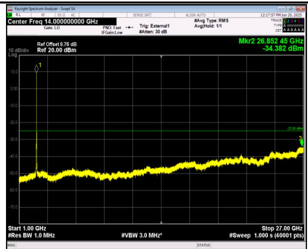
41(2555-2655)-41(2555-2655)-15MHz-10MHz-16QAM-16Q AM-40691-40811-1RB#0-ORB#0-1000~27000MHz-PASS
