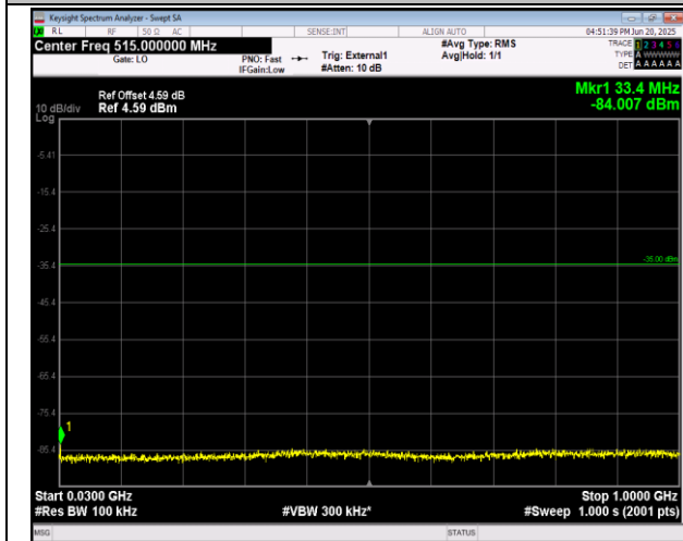
41(2555-2655)-41(2555-2655)-15MHz-20MHz-QPSK-QP SK-40318-40489-1RB#74-ORB#0-30~1000MHz-PASS
