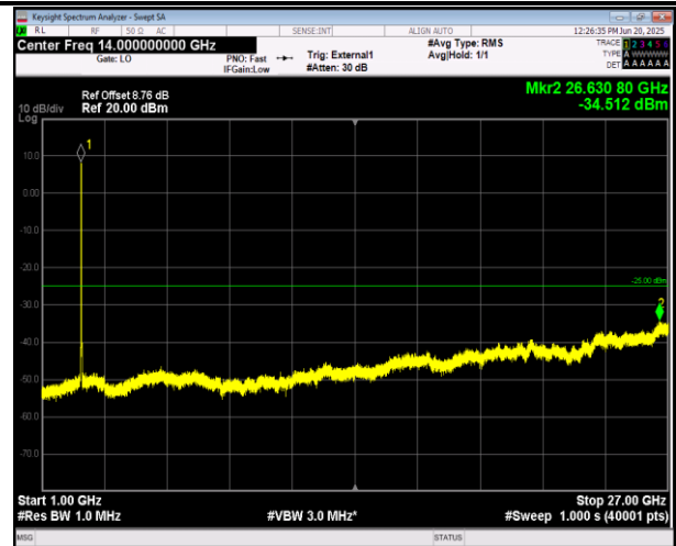
41(2555-2655)-41(2555-2655)-15MHz-15MHz-QPSK-QPS K-40315-40465-1RB#0-ORB#0-1000~27000MHz-PASS
