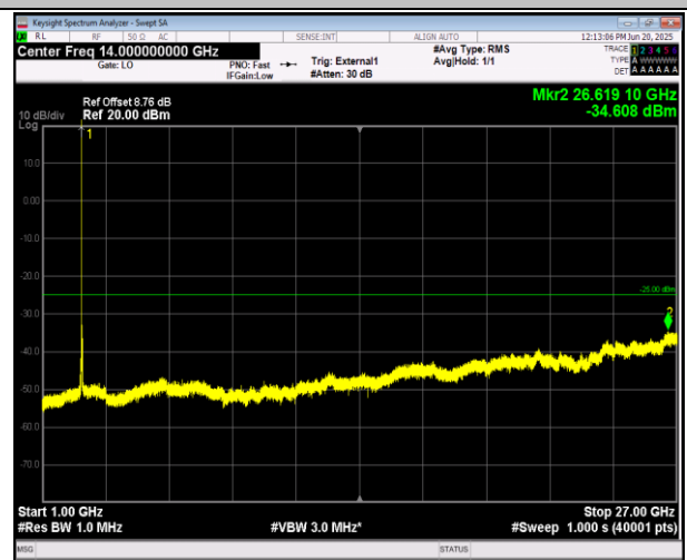
41(2555-2655)-41(2555-2655)-15MHz-10MHz-16QAM-16Q AM-40691-40811-1RB#0-1RB#49-1000~27000MHz-PASS
