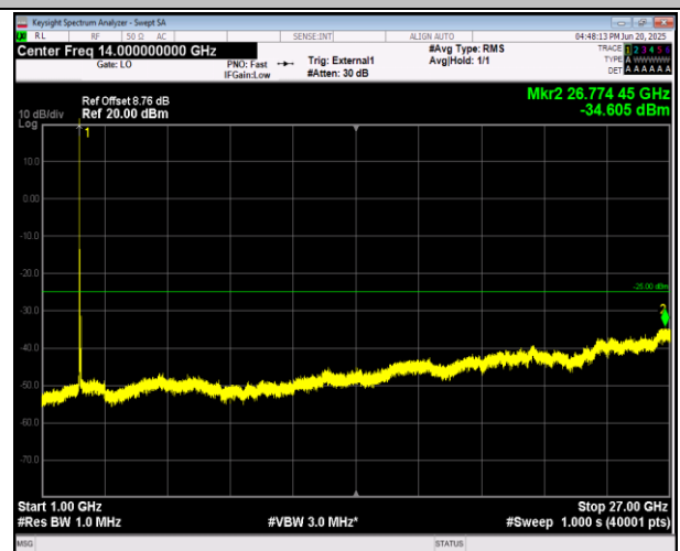
41(2555-2655)-41(2555-2655)-15MHz-20MHz-QPSK-QPS K-40318-40489-1RB#0-1RB#99-1000~27000MHz-PASS
