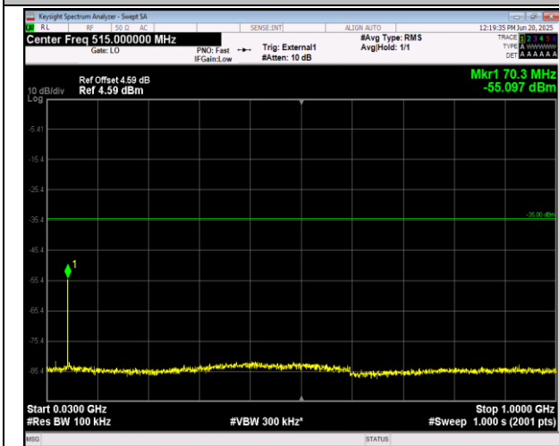
41(2555-2655)-41(2555-2655)-15MHz-10MHz-QPSK-QP SK-41067-41187-1RB#0-1RB#49-30~1000MHz-PASS
