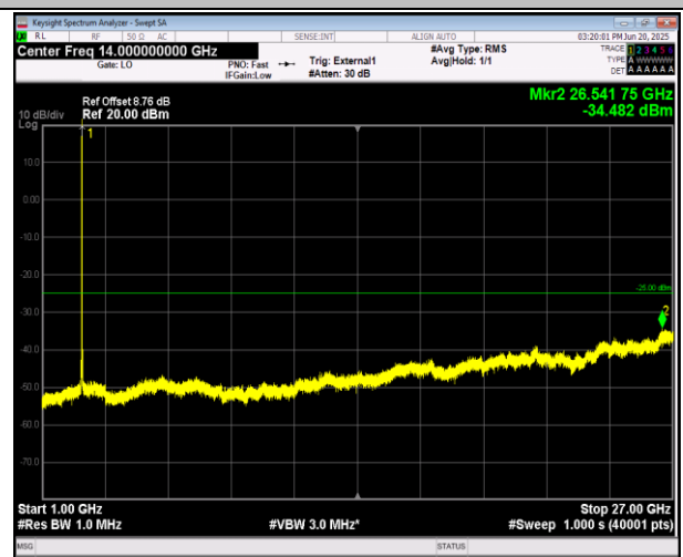
41(2555-2655)-41(2555-2655)-15MHz-15MHz-QPSK-QPS K-41015-41165-75RB#0-75RB#0-1000~27000MHz-PASS
