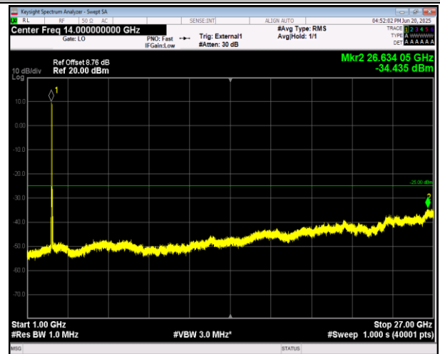
41(2555-2655)-41(2555-2655)-15MHz-20MHz-QPSK-QPS K-40318-40489-1RB#74-ORB#0-1000~27000MHz-PASS
