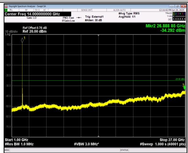
41(2555-2655)-41(2555-2655)-15MHz-10MHz-QPSK-QPS K-40691-40811-1RB#74-0RB#0-1000~27000MHz-PASS
