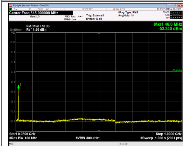
41(2555-2655)-41(2555-2655)-15MHz-10MHz-QPSK-QP SK-40691-40811-75RB#0-50RB#0-30~1000MHz-PASS
