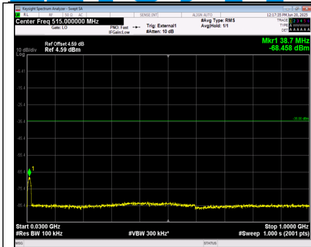
41(2555-2655)-41(2555-2655)-15MHz-10MHz-16QAM-16 QAM-40691-40811-1RB#0-ORB#0-30~1000MHz-PASS
