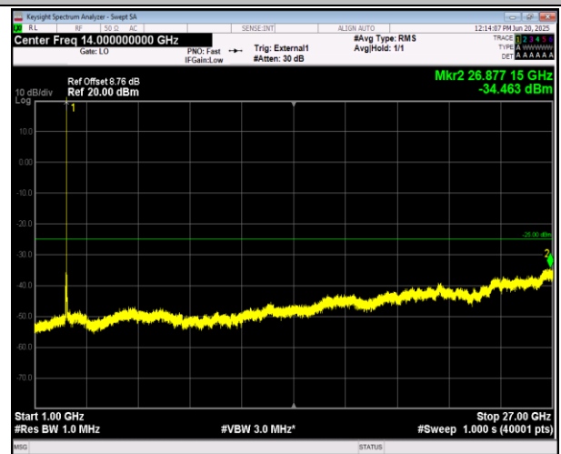
41(2555-2655)-41(2555-2655)-15MHz-10MHz-QPSK-QPS K-40691-40811-75RB#0-50RB#0-1000~27000MHz-PASS
