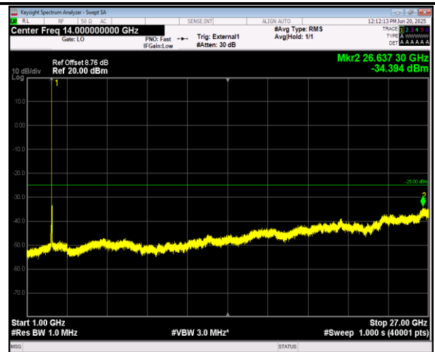
41(2555-2655)-41(2555-2655)-15MHz-10MHz-QPSK-QPS K-40691-40811-1RB#0-1RB#49-1000~27000MHz-PASS
