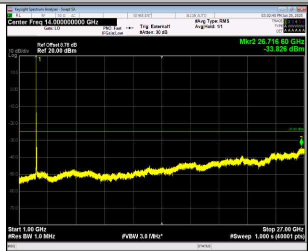
41(2555-2655)-41(2555-2655)-15MHz-15MHz-QPSK-QPS K-40315-40465-1RB#0-1RB#74-1000~27000MHz-PASS
