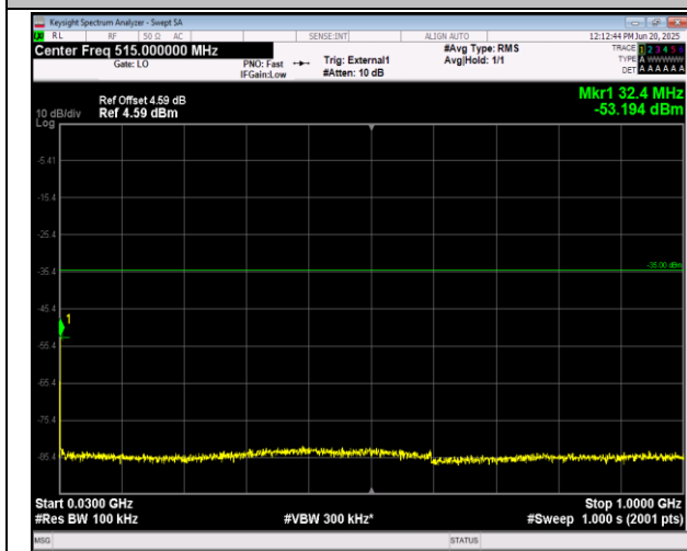
41(2555-2655)-41(2555-2655)-15MHz-10MHz-16QAM-16 QAM-40691-40811-1RB#0-1RB#49-30~1000MHz-PASS
