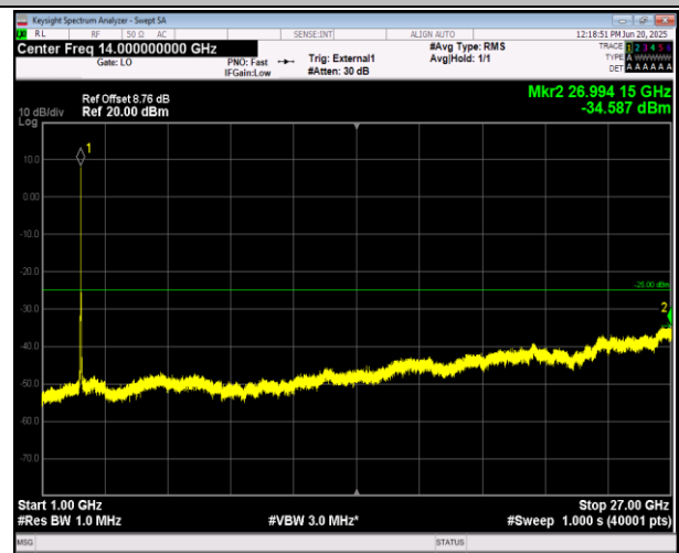
41(2555-2655)-41(2555-2655)-15MHz-10MHz-QPSK-QPS K-41067-41187-1RB#0-0RB#0-1000~27000MHz-PASS
