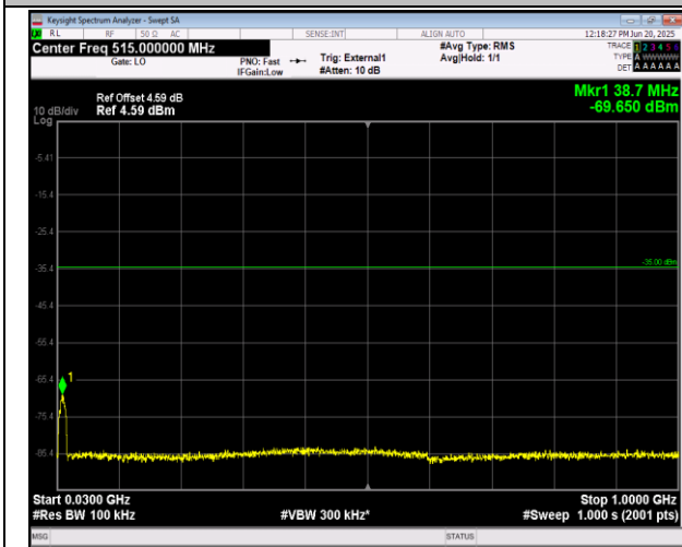
41(2555-2655)-41(2555-2655)-15MHz-10MHz-QPSK-QP SK-41067-41187-1RB#0-0RB#0-30~1000MHz-PASS
