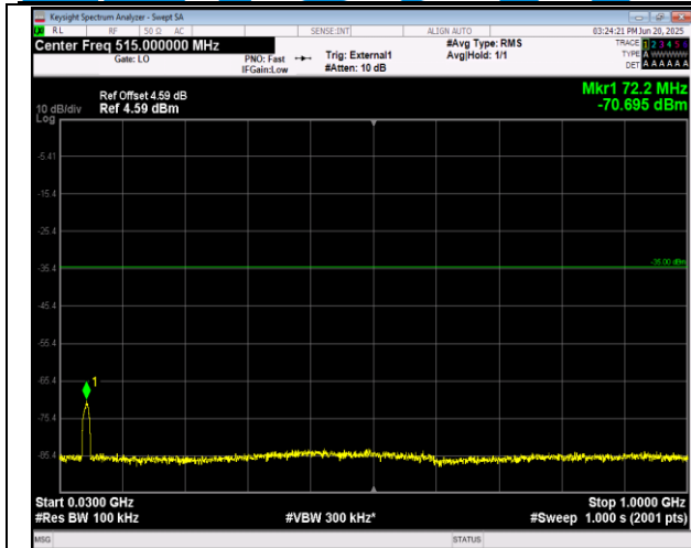
41(2555-2655)-41(2555-2655)-15MHz-20MHz-QPSK-QP SK-40318-40489-1RB#0-ORB#0-30~1000MHz-PASS
