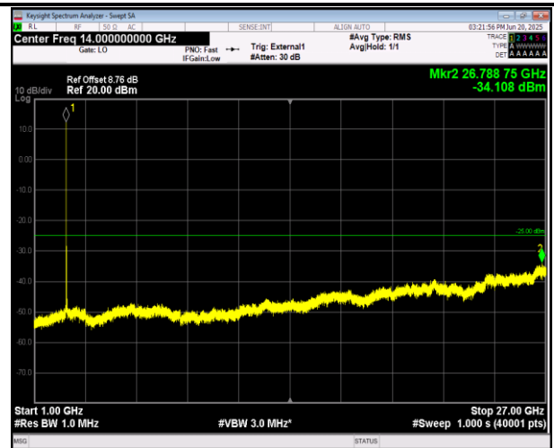
41(2555-2655)-41(2555-2655)-15MHz-15MHz-QPSK-QPS K-41015-41165-1RB#74-ORB#0-1000~27000MHz-PASS
