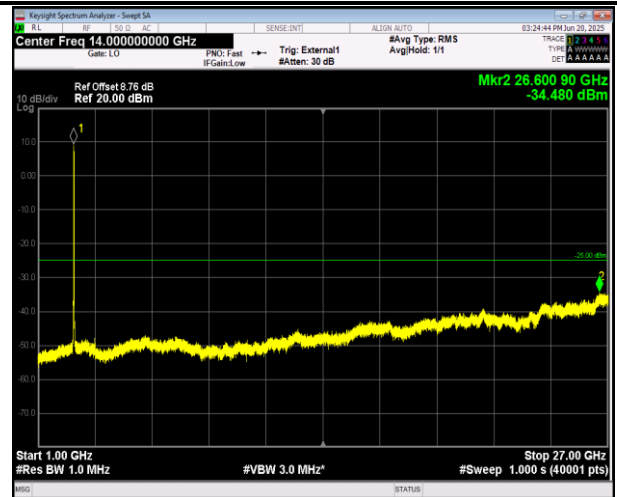
41(2555-2655)-41(2555-2655)-15MHz-20MHz-QPSK-QPS K-40318-40489-1RB#0-ORB#0-1000~27000MHz-PASS
