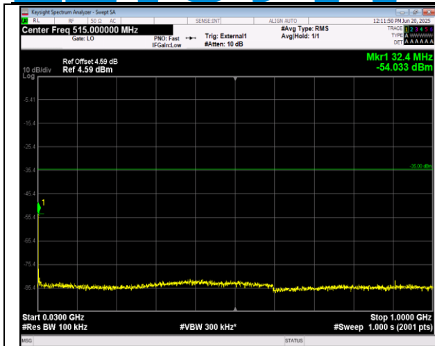
41(2555-2655)-41(2555-2655)-15MHz-10MHz-QPSK-QP SK-40691-40811-1RB#0-1RB#49-30~1000MHz-PASS
