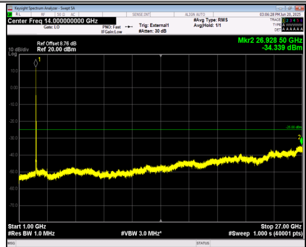
41(2555-2655)-41(2555-2655)-15MHz-15MHz-QPSK-QPS K-40315-40465-1RB#74-ORB#0-1000~27000MHz-PASS
