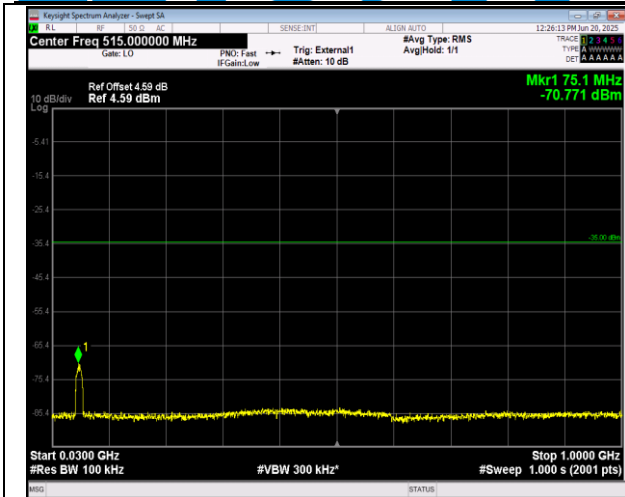
41(2555-2655)-41(2555-2655)-15MHz-15MHz-QPSK-QP SK-40315-40465-1RB#0-ORB#0-30~1000MHz-PASS
