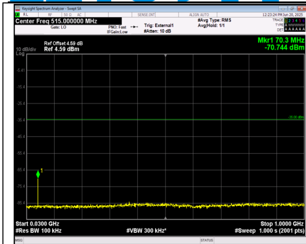
41(2555-2655)-41(2555-2655)-15MHz-10MHz-QPSK-QP SK-41067-41187-1RB#74-ORB#0-30~1000MHz-PASS
