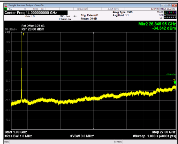
41(2555-2655)-41(2555-2655)-15MHz-10MHz-QPSK-QPS K-41067-41187-1RB#0-1RB#49-1000~27000MHz-PASS
