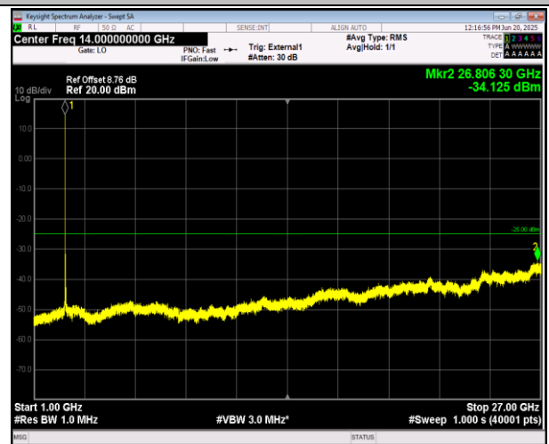
41(2555-2655)-41(2555-2655)-15MHz-10MHz-16QAM-16Q AM-40691-40811-1RB#74-ORB#0-1000~27000MHz-PASS
