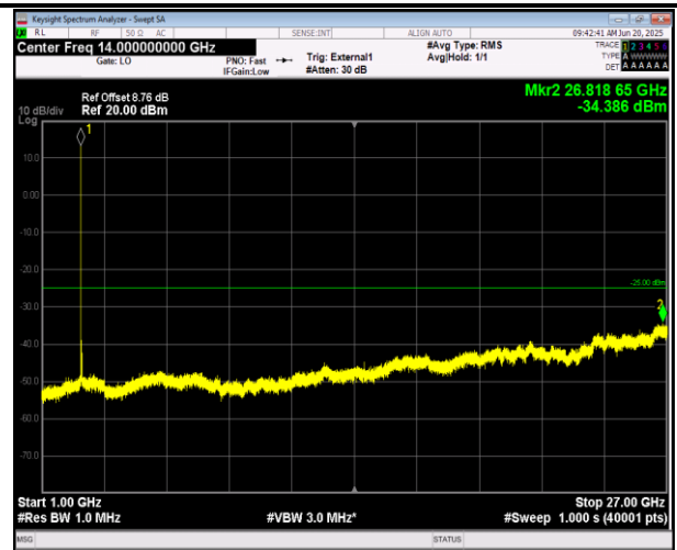
41(2555-2655)-41(2555-2655)-10MHz-20MHz-QPSK-QPS K-40996-41140-1RB#49-ORB#0-1000~27000MHz-PASS
