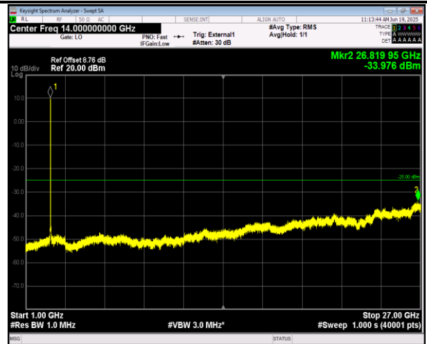
41(2555-2655)-41(2555-2655)-10MHz-20MHz-QPSK-QPS K-40295-40439-1RB#0-ORB#0-1000~27000MHz-PASS
