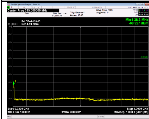
41(2555-2655)-41(2555-2655)-10MHz-15MHz-QPSK-QP SK-41045-41165-1RB#0-0RB#0-30~1000MHz-PASS
