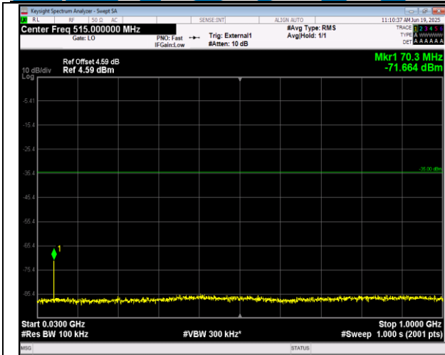
41(2555-2655)-41(2555-2655)-10MHz-15MHz-QPSK-QP SK-41045-41165-1RB#49-ORB#0-30~1000MHz-PASS
