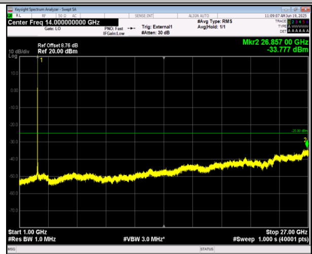
41(2555-2655)-41(2555-2655)-10MHz-15MHz-QPSK-QPS K-41045-41165-50RB#0-75RB#0-1000~27000MHz-PASS
