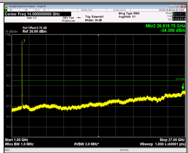
41(2555-2655)-41(2555-2655)-10MHz-20MHz-16QAM-16Q AM-40295-40439-1RB#0-0RB#0-1000~27000MHz-PASS
