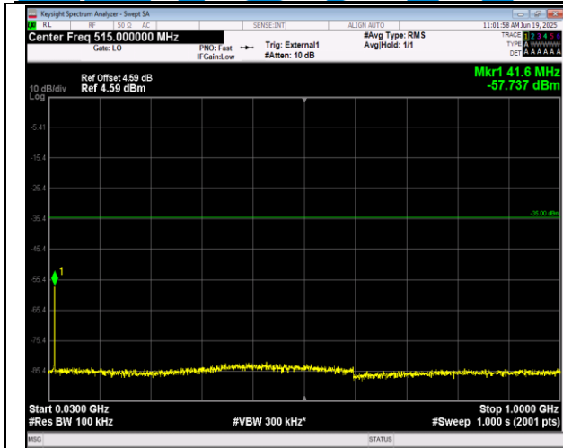
41(2555-2655)-41(2555-2655)-10MHz-15MHz-16QAM-16 QAM-40669-40789-50RB#0-75RB#0-30~1000MHz-PASS
