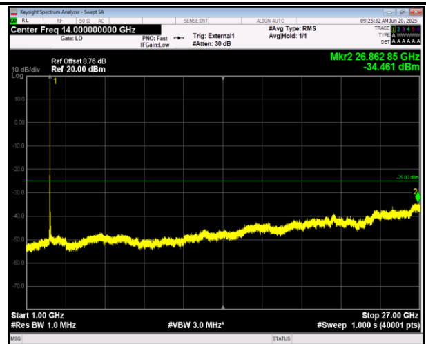
41(2555-2655)-41(2555-2655)-10MHz-20MHz-QPSK-QPS K-40295-40439-50RB#0-100RB#0-1000~27000MHz-PASS
