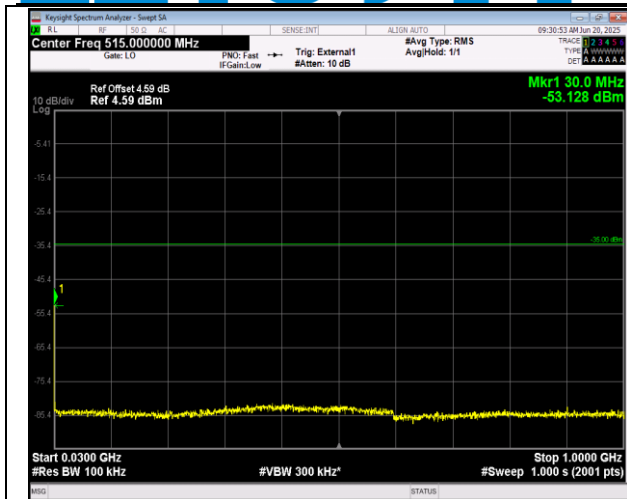
41(2555-2655)-41(2555-2655)-10MHz-20MHz-QPSK-QP SK-40646-40790-1RB#0-1RB#99-30~1000MHz-PASS
