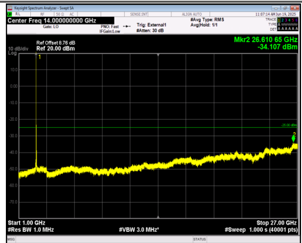
41(2555-2655)-41(2555-2655)-10MHz-15MHz-QPSK-QPS K-41045-41165-1RB#0-1RB#74-1000~27000MHz-PASS
