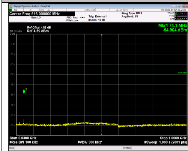
41(2555-2655)-41(2555-2655)-10MHz-20MHz-QPSK-QP SK-40996-41140-50RB#0-100RB#0-30~1000MHz-PASS
