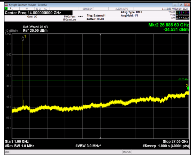
41(2555-2655)-41(2555-2655)-10MHz-15MHz-QPSK-QPS K-41045-41165-1RB#49-ORB#0-1000~27000MHz-PASS
