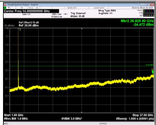
41(2555-2655)-41(2555-2655)-10MHz-20MHz-16QAM-16Q AM-40295-40439-1RB#0-1RB#99-1000~27000MHz-PASS
