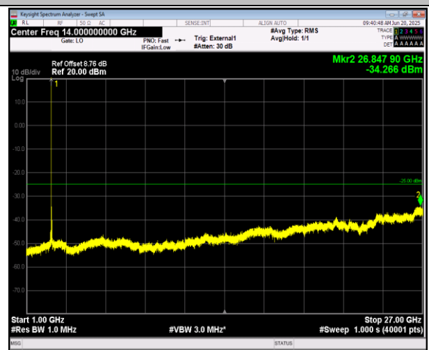
41(2555-2655)-41(2555-2655)-10MHz-20MHz-QPSK-QPS K-40996-41140-50RB#0-100RB#0-1000~27000MHz-PASS
