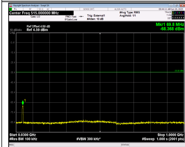
41(2555-2655)-41(2555-2655)-10MHz-20MHz-16QAM-16 QAM-40996-41140-1RB#0-ORB#0-30~1000MHz-PASS
