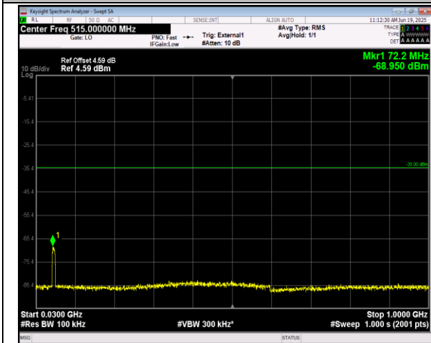
41(2555-2655)-41(2555-2655)-10MHz-15MHz-16QAM-16 QAM-41045-41165-1RB#0-ORB#0-30~1000MHz-PASS
