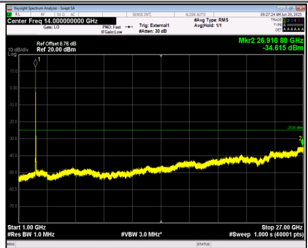
41(2555-2655)-41(2555-2655)-10MHz-20MHz-QPSK-QPS K-40295-40439-1RB#49-ORB#0-1000~27000MHz-PASS
