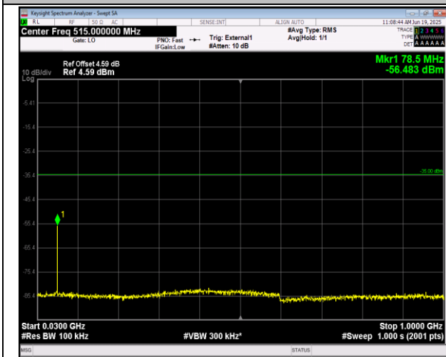
41(2555-2655)-41(2555-2655)-10MHz-15MHz-QPSK-QP SK-41045-41165-50RB#0-75RB#0-30~1000MHz-PASS
