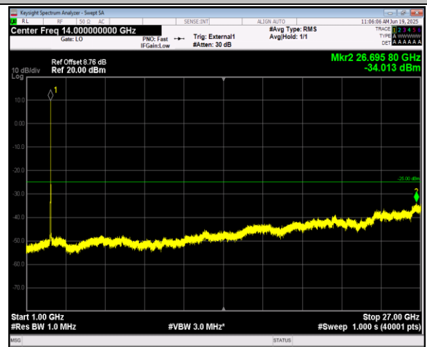
41(2555-2655)-41(2555-2655)-10MHz-15MHz-QPSK-QPS K-41045-41165-1RB#0-0RB#0-1000~27000MHz-PASS
