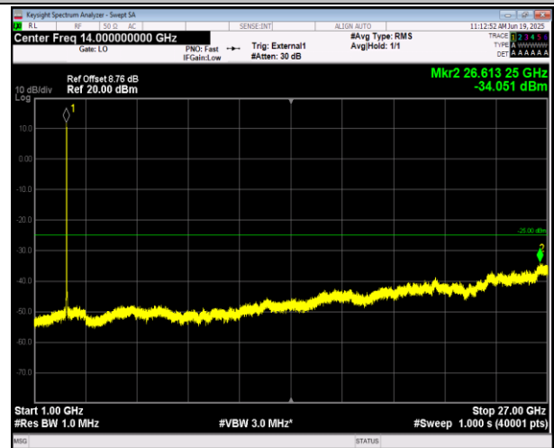
41(2555-2655)-41(2555-2655)-10MHz-15MHz-16QAM-16Q AM-41045-41165-1RB#0-ORB#0-1000~27000MHz-PASS
