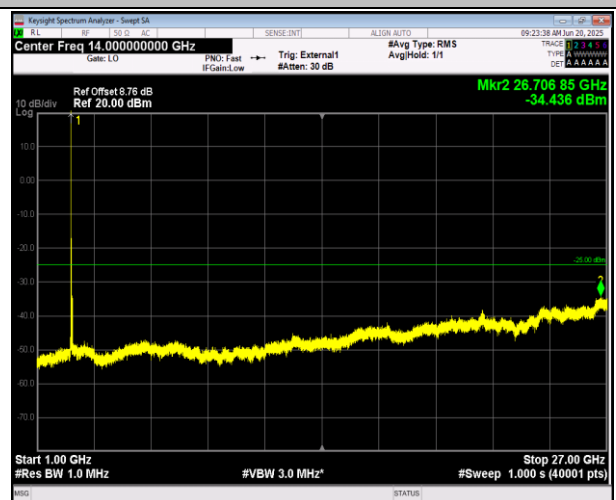
41(2555-2655)-41(2555-2655)-10MHz-20MHz-QPSK-QPS K-40295-40439-1RB#0-1RB#99-1000~27000MHz-PASS
