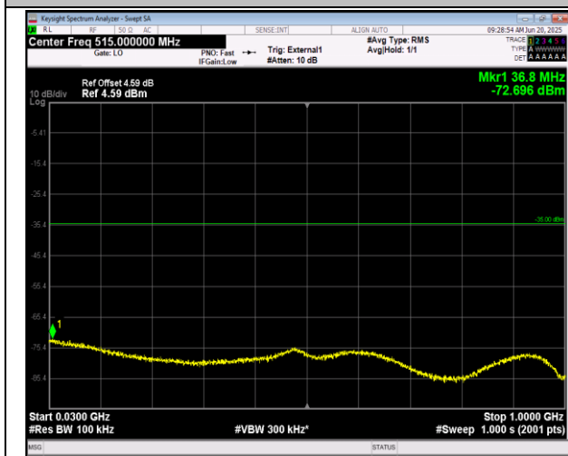
41(2555-2655)-41(2555-2655)-10MHz-20MHz-16QAM-16 QAM-40295-40439-1RB#0-0RB#0-30~1000MHz-PASS
