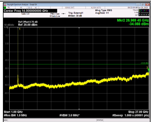
41(2555-2655)-41(2555-2655)-10MHz-20MHz-QPSK-QPS K-40646-40790-50RB#0-100RB#0-1000~27000MHz-PASS
