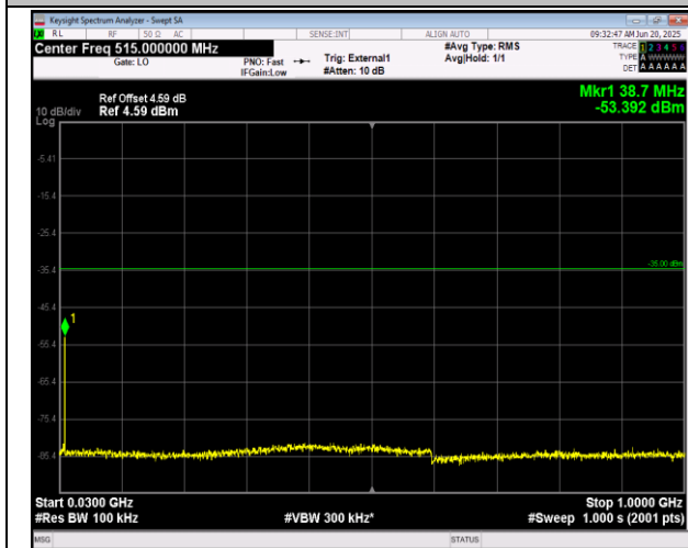
41(2555-2655)-41(2555-2655)-10MHz-20MHz-QPSK-QP SK-40646-40790-50RB#0-100RB#0-30~1000MHz-PASS
