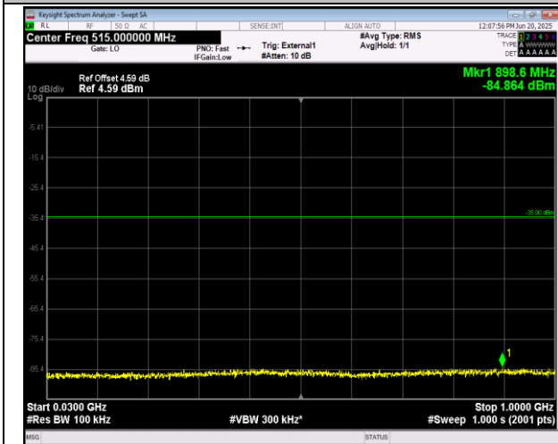
41(2555-2655)-41(2555-2655)-15MHz-10MHz-QPSK-QP SK-40315-40435-1RB#74-ORB#0-30~1000MHz-PASS
