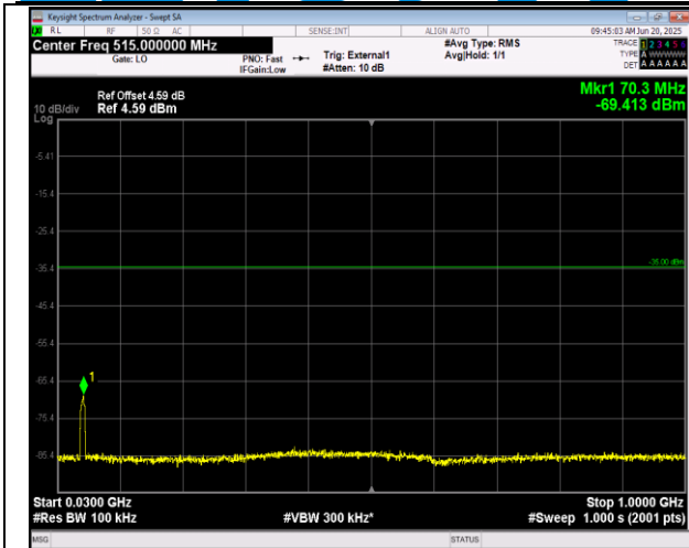
41(2555-2655)-41(2555-2655)-15MHz-10MHz-QPSK-QP SK-40315-40435-1RB#0-ORB#0-30~1000MHz-PASS
