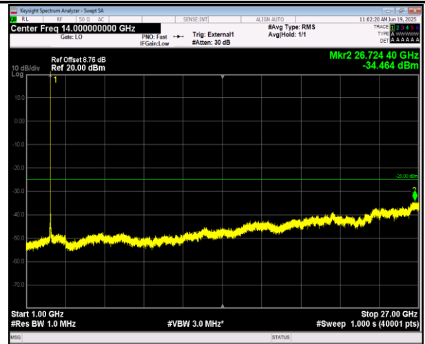
41(2555-2655)-41(2555-2655)-10MHz-15MHz-16QAM-16Q AM-40669-40789-50RB#0-75RB#0-1000~27000MHz-PASS
