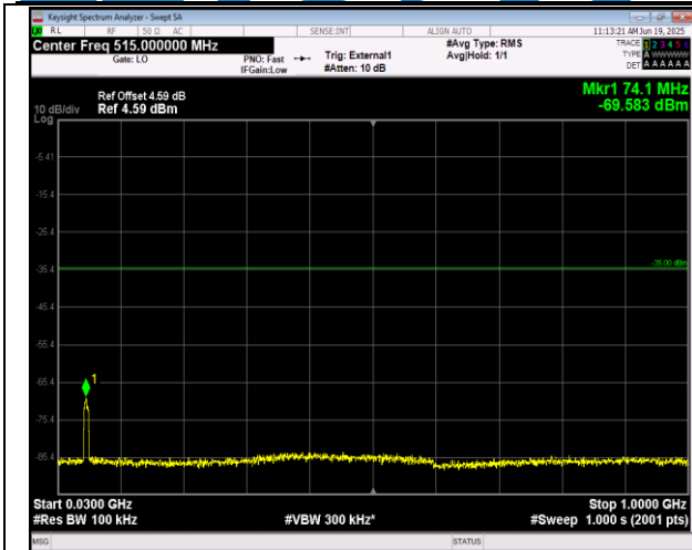
41(2555-2655)-41(2555-2655)-10MHz-20MHz-QPSK-QP SK-40295-40439-1RB#0-ORB#0-30~1000MHz-PASS
