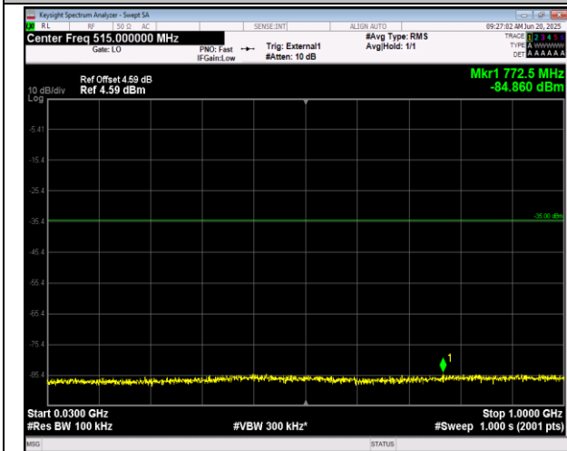
41(2555-2655)-41(2555-2655)-10MHz-20MHz-QPSK-QP SK-40295-40439-1RB#49-ORB#0-30~1000MHz-PASS
