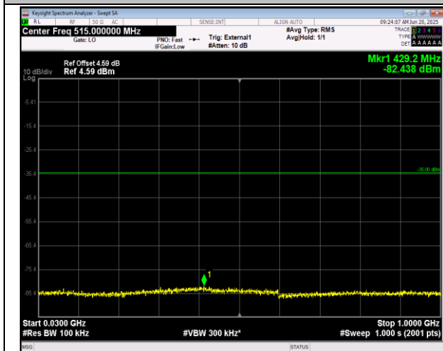
41(2555-2655)-41(2555-2655)-10MHz-20MHz-16QAM-16 QAM-40295-40439-1RB#0-1RB#99-30~1000MHz-PASS
