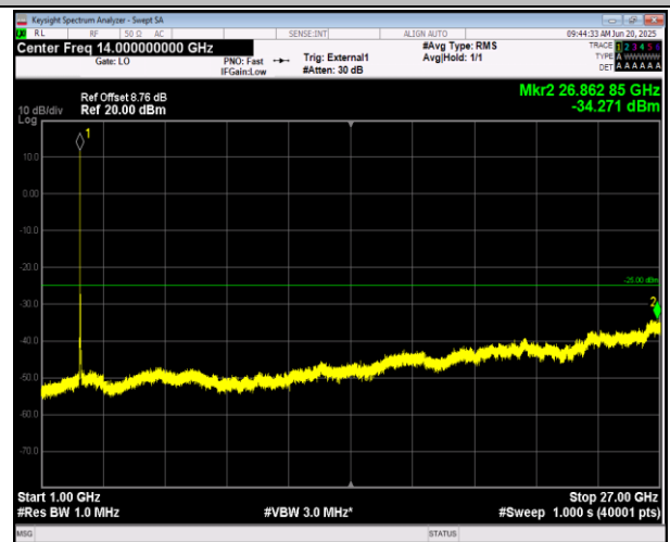
41(2555-2655)-41(2555-2655)-10MHz-20MHz-16QAM-16 AM-40996-41140-1RB#0-ORB#0-1000~27000MHz-PASS
