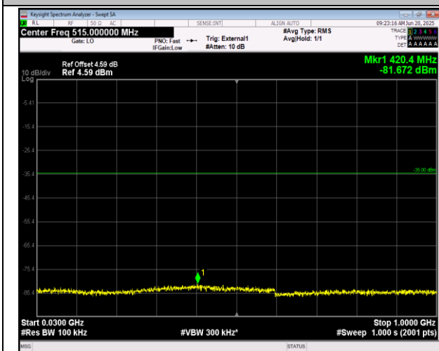
41(2555-2655)-41(2555-2655)-10MHz-20MHz-QPSK-QP SK-40295-40439-1RB#0-1RB#99-30~1000MHz-PASS
