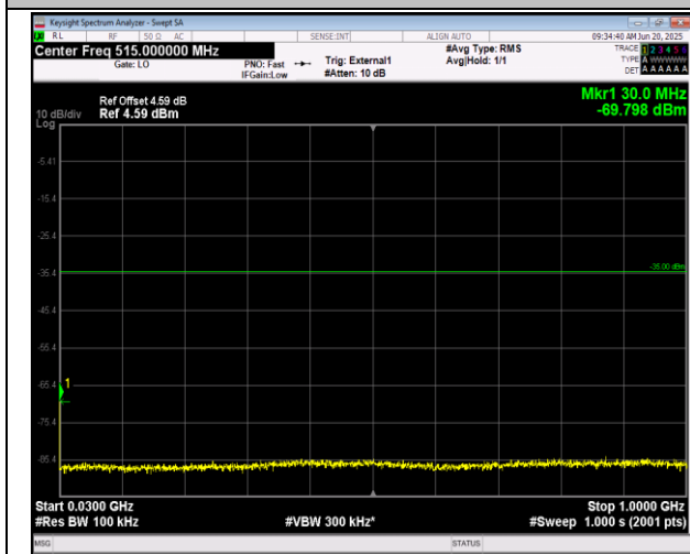
41(2555-2655)-41(2555-2655)-10MHz-20MHz-QPSK-QP SK-40646-40790-1RB#49-0RB#0-30~1000MHz-PASS
