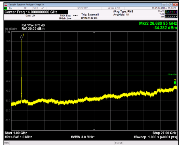
41(2555-2655)-41(2555-2655)-15MHz-10MHz-QPSK-QPS K-40315-40435-1RB#0-ORB#0-1000~27000MHz-PASS
