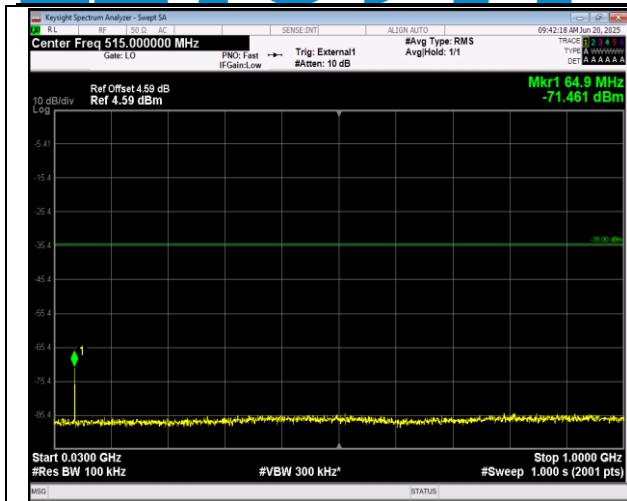
41(2555-2655)-41(2555-2655)-10MHz-20MHz-QPSK-QP SK-40996-41140-1RB#49-ORB#0-30~1000MHz-PASS
