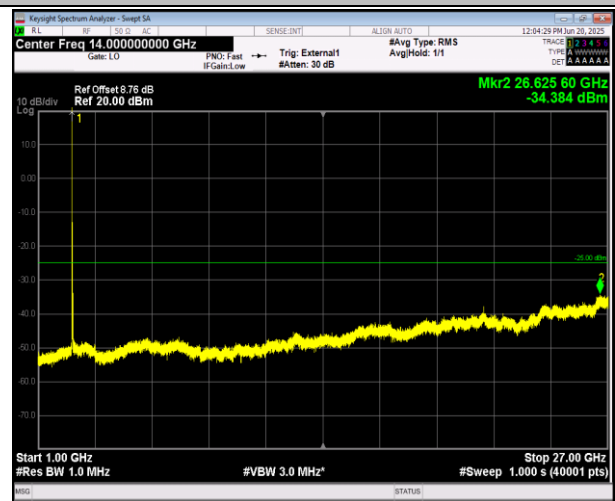
41(2555-2655)-41(2555-2655)-15MHz-10MHz-QPSK-QPS K-40315-40435-1RB#0-1RB#49-1000~27000MHz-PASS
