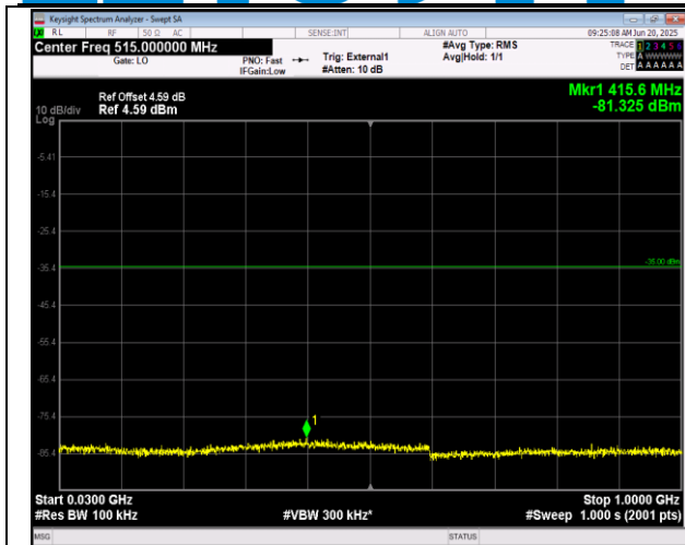
41(2555-2655)-41(2555-2655)-10MHz-20MHz-QPSK-QP SK-40295-40439-50RB#0-100RB#0-30~1000MHz-PASS
