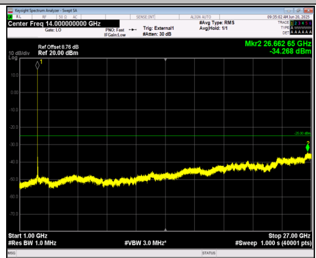
41(2555-2655)-41(2555-2655)-10MHz-20MHz-QPSK-QPS K-40646-40790-1RB#49-0RB#0-1000~27000MHz-PASS
