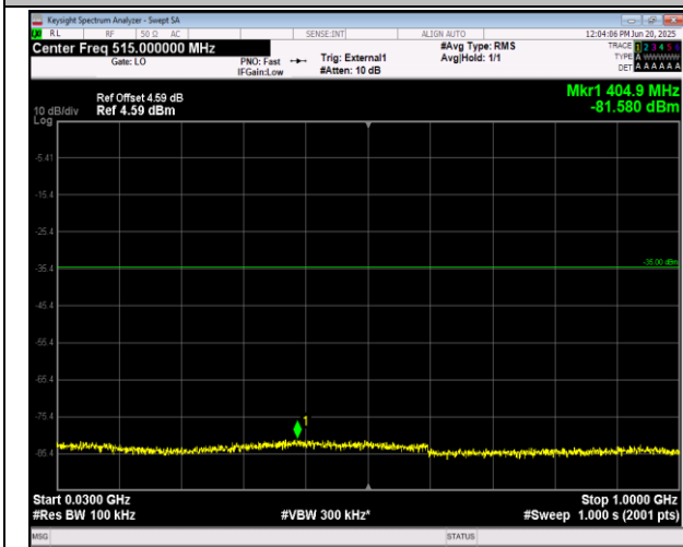
41(2555-2655)-41(2555-2655)-15MHz-10MHz-QPSK-QP SK-40315-40435-1RB#0-1RB#49-30~1000MHz-PASS
