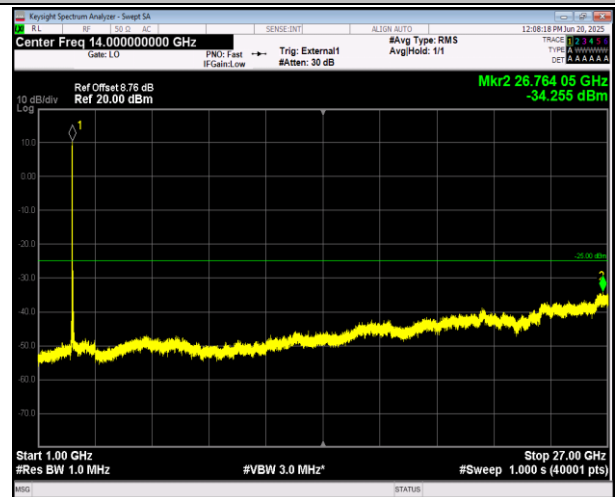
41(2555-2655)-41(2555-2655)-15MHz-10MHz-QPSK-QPS K-40315-40435-1RB#74-ORB#0-1000~27000MHz-PASS
