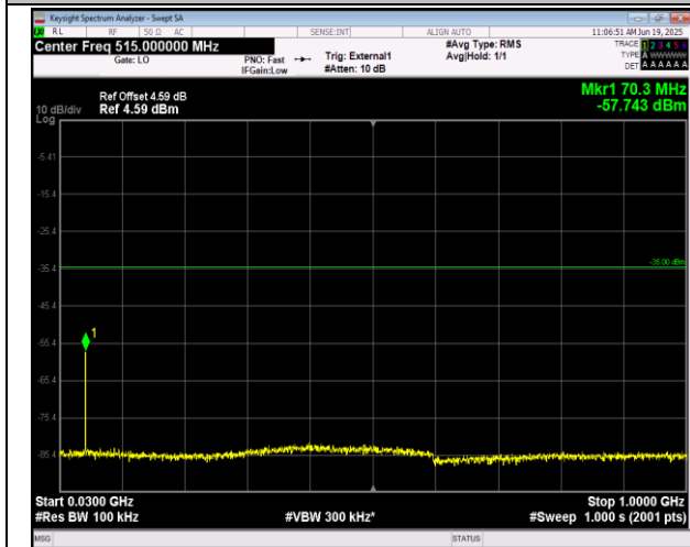
41(2555-2655)-41(2555-2655)-10MHz-15MHz-QPSK-QP SK-41045-41165-1RB#0-1RB#74-30~1000MHz-PASS
