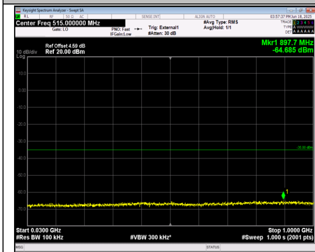
38-38-20MHz-20MHz-QPSK-QPSK-37901-38099-1RB#9-9-0RB#0-30~1000MHz-PASS
