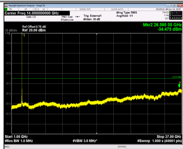
41(2555-2655)-41(2555-2655)-5MHz-20MHz-QPSK-QPSK- 40648-40765-25RB#0-100RB#0-1000~27000MHz-PASS
