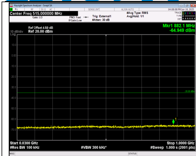
41(2555-2655)-41(2555-2655)-5MHz-20MHz-QPSK-QPS K-40273-40390-1RB#0-0RB#0-30~1000MHz-PASS
