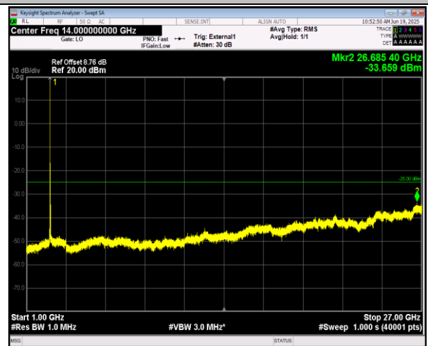
41(2555-2655)-41(2555-2655)-10MHz-15MHz-16QAM-16Q AM-40293-40413-1RB#0-1RB#74-1000~27000MHz-PASS
