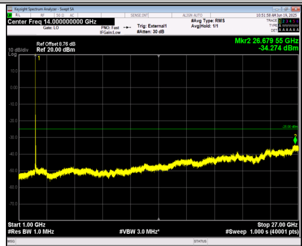
41(2555-2655)-41(2555-2655)-10MHz-15MHz-QPSK-QPS K-40293-40413-1RB#0-1RB#74-1000~27000MHz-PASS
