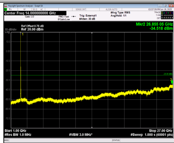
38-38-20MHz-20MHz-QPSK-QPSK-37901-38099-1RB#99-0RB#0-1000~27000MHz-PASS
