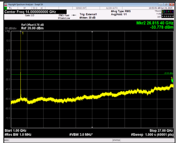
41(2555-2655)-41(2555-2655)-10MHz-15MHz-QPSK-QPS K-40293-40413-50RB#0-75RB#0-1000~27000MHz-PASS
