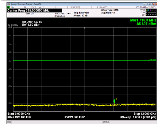
41(2555-2655)-41(2555-2655)-10MHz-15MHz-QPSK-QP SK-40293-40413-1RB#49-ORB#0-30~1000MHz-PASS
