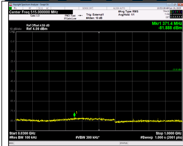
41(2555-2655)-41(2555-2655)-10MHz-15MHz-QPSK-QP SK-40293-40413-50RB#0-75RB#0-30~1000MHz-PASS
