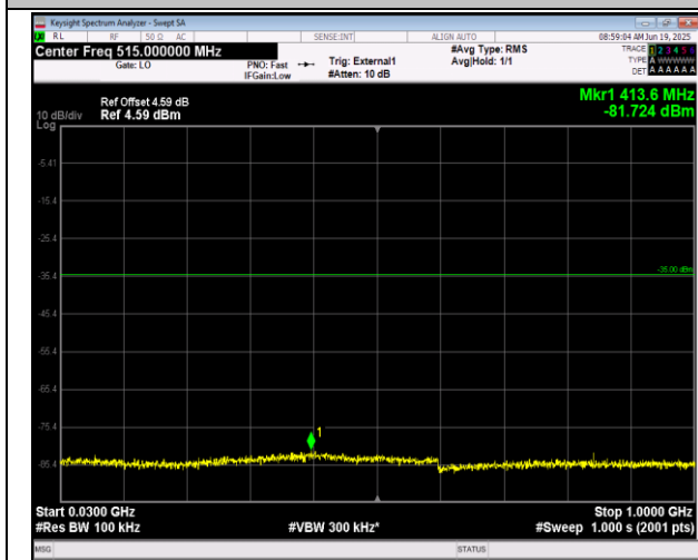
41(2555-2655)-41(2555-2655)-5MHz-20MHz-QPSK-QPS K-40273-40390-1RB#0-1RB#99-30~1000MHz-PASS
