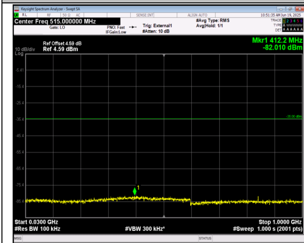
41(2555-2655)-41(2555-2655)-10MHz-15MHz-QPSK-QP SK-40293-40413-1RB#0-1RB#74-30~1000MHz-PASS
