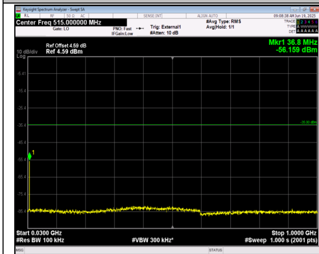
41(2555-2655)-41(2555-2655)-5MHz-20MHz-QPSK-QPS K-40648-40765-25RB#0-100RB#0-30~1000MHz-PASS
