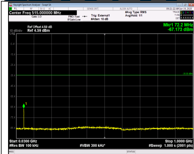
41(2555-2655)-41(2555-2655)-10MHz-15MHz-QPSK-QP SK-40293-40413-1RB#0-ORB#0-30~1000MHz-PASS
