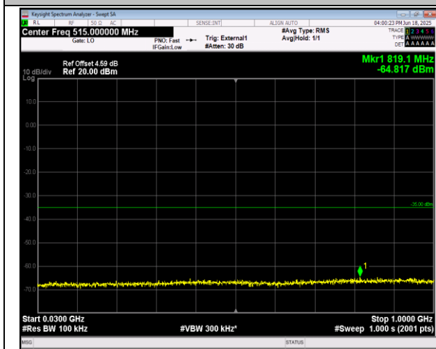
38-38-20MHz-20MHz-QPSK-QPSK-37952-38150-1RB#0- ORB#0-30~1000MHz-PASS
