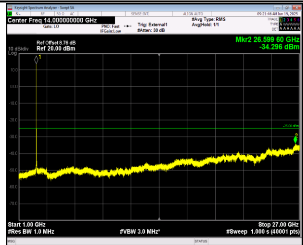
41(2555-2655)-41(2555-2655)-10MHz-15MHz-QPSK-QPS K-40293-40413-1RB#0-ORB#0-1000~27000MHz-PASS
