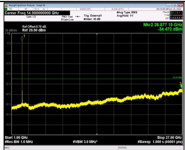
41(2555-2655)-41(2555-2655)-5MHz-20MHz-QPSK-QPSK- 41023-41140-1RB#24-0RB#0-1000~27000MHz-PASS
