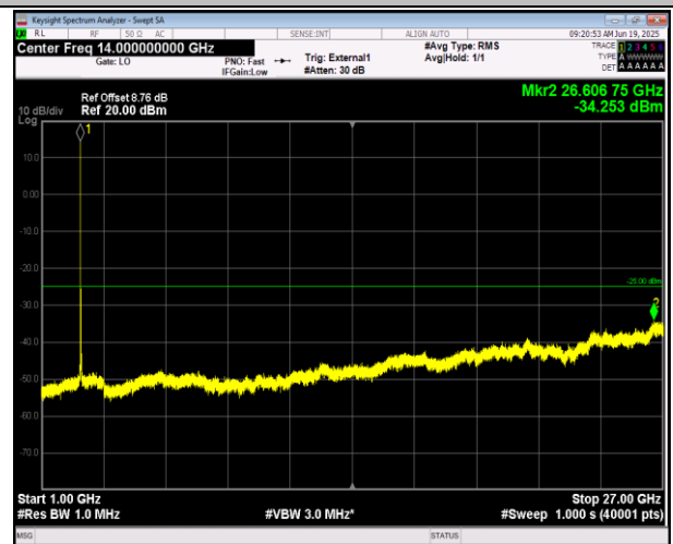
41(2555-2655)-41(2555-2655)-5MHz-20MHz-16QAM-16QA M-41023-41140-1RB#0-0RB#0-1000~27000MHz-PASS
