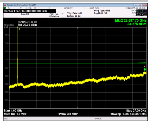
38-38-20MHz-20MHz-QPSK-QPSK-37952-38150-100RB#0 -100RB#0-1000~27000MHz-PASS
