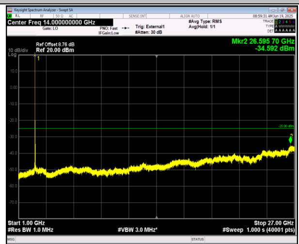
41(2555-2655)-41(2555-2655)-5MHz-20MHz-QPSK-QPSK- 40273-40390-1RB#0-1RB#99-1000~27000MHz-PASS
