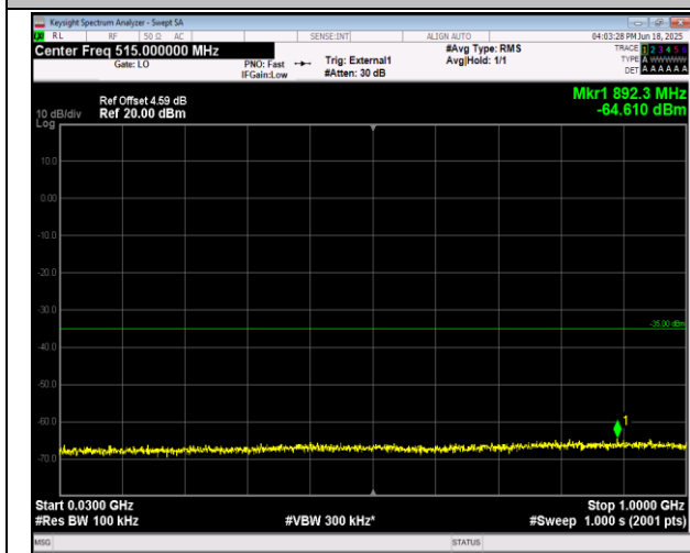
38-38-20MHz-20MHz-QPSK-QPSK-37952-38150-100RB #0-100RB#0-30~1000MHz-PASS
