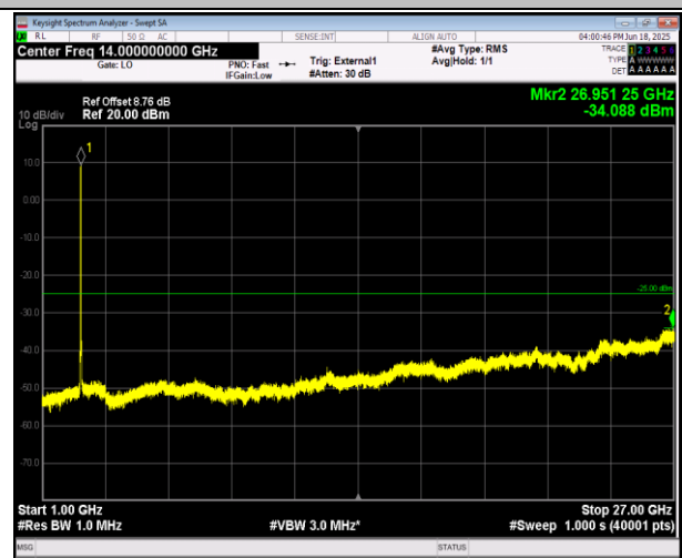
38-38-20MHz-20MHz-QPSK-QPSK-37952-38150-1RB#0-0 RB#0-1000~27000MHz-PASS
