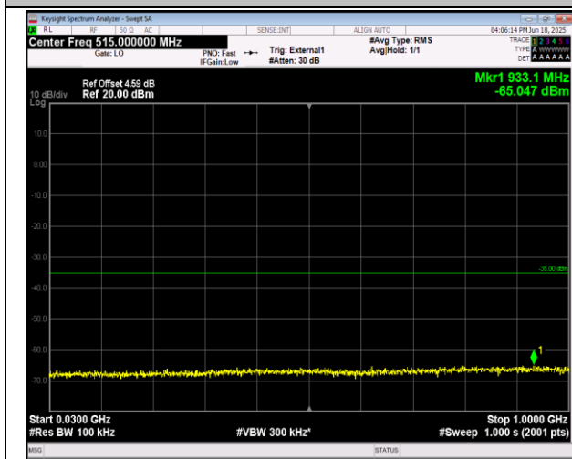
38-38-20MHz-20MHz-16QAM-16QAM-37952-38150-1RB #99-0RB#0-30~1000MHz-PASS
