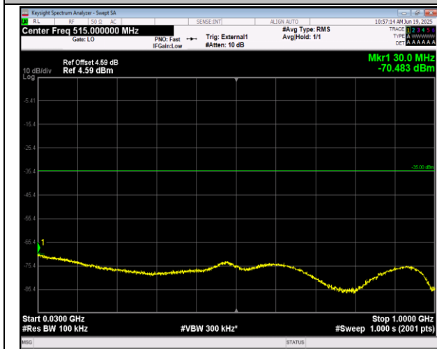
41(2555-2655)-41(2555-2655)-10MHz-15MHz-16QAM-16 QAM-40293-40413-1RB#0-0RB#0-30~1000MHz-PASS
