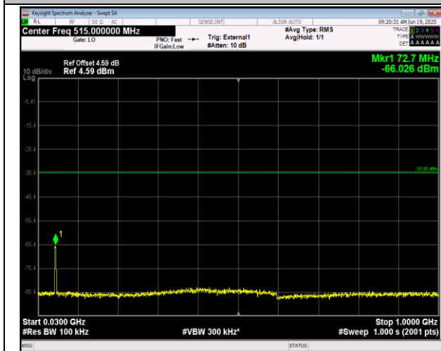
41(2555-2655)-41(2555-2655)-5MHz-20MHz-16QAM-16 QAM-41023-41140-1RB#0-0RB#0-30~1000MHz-PASS
