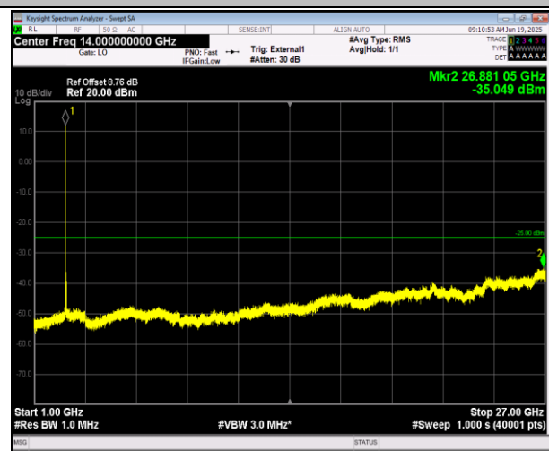
41(2555-2655)-41(2555-2655)-5MHz-20MHz-QPSK-QPSK- 40648-40765-1RB#24-0RB#0-1000~27000MHz-PASS
