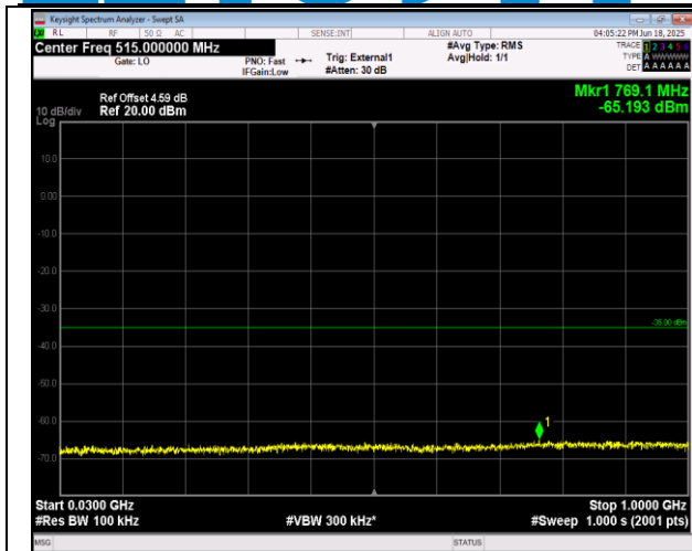
38-38-20MHz-20MHz-QPSK-QPSK-37952-38150-1RB#9 9-0RB#0-30~1000MHz-PASS
