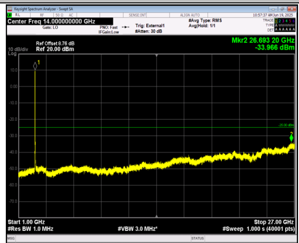
41(2555-2655)-41(2555-2655)-10MHz-15MHz-16QAM-16Q AM-40293-40413-1RB#0-0RB#0-1000~27000MHz-PASS
