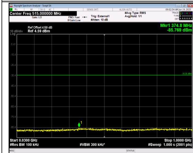
41(2555-2655)-41(2555-2655)-5MHz-20MHz-QPSK-QPS K-40273-40390-1RB#24-0RB#0-30~1000MHz-PASS
