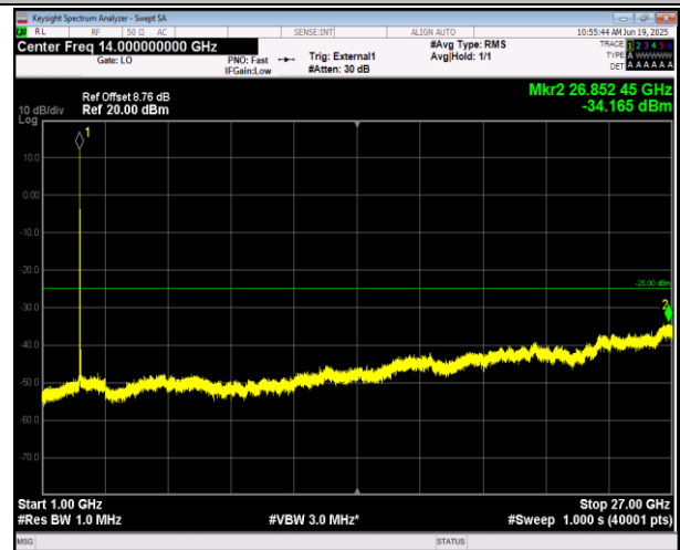
41(2555-2655)-41(2555-2655)-10MHz-15MHz-QPSK-QPS K-40293-40413-1RB#49-ORB#0-1000~27000MHz-PASS
