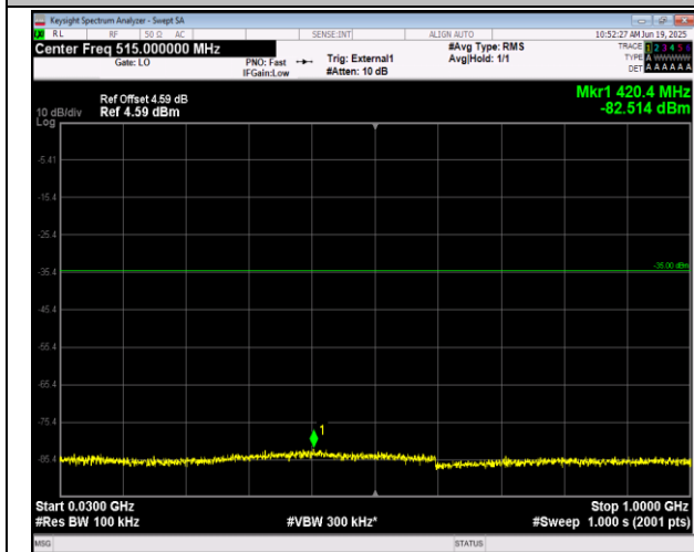
41(2555-2655)-41(2555-2655)-10MHz-15MHz-16QAM-16 QAM-40293-40413-1RB#0-1RB#74-30~1000MHz-PASS
