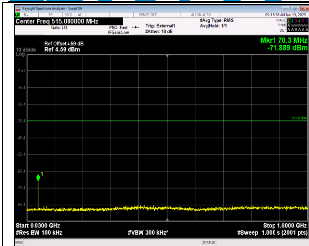
41(2555-2655)-41(2555-2655)-5MHz-20MHz-QPSK-QPS K-41023-41140-1RB#24-0RB#0-30~1000MHz-PASS
