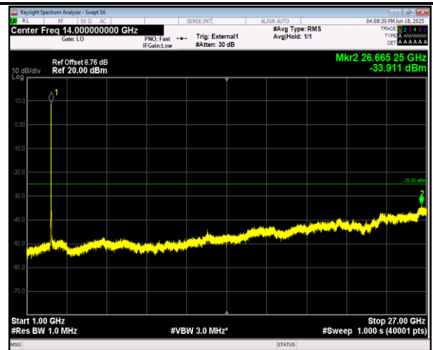
41(2555-2655)-41(2555-2655)-5MHz-20MHz-QPSK-QPSK- 40273-40390-1RB#0-0RB#0-1000~27000MHz-PASS
