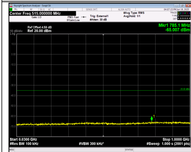
38-38-20MHz-20MHz-16QAM-16QAM-37952-38150-1RB #0-0RB#0-30~1000MHz-PASS
