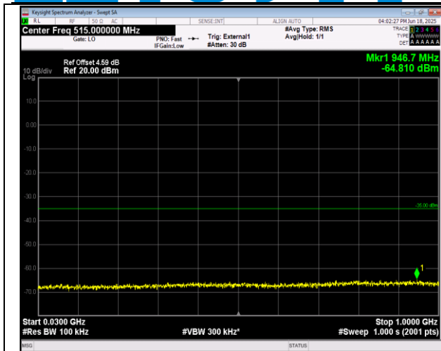
38-38-20MHz-20MHz-16QAM-16QAM-37952-38150-1RB #0-1RB#99-30~1000MHz-PASS
