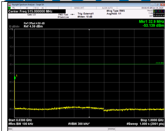
41(2555-2655)-41(2555-2655)-5MHz-20MHz-QPSK-QPS K-40648-40765-1RB#0-1RB#99-30~1000MHz-PASS
