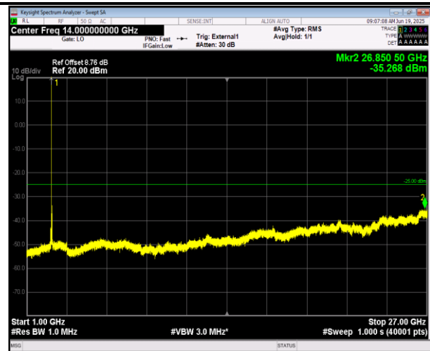
41(2555-2655)-41(2555-2655)-5MHz-20MHz-QPSK-QPSK- 40648-40765-1RB#0-1RB#99-1000~27000MHz-PASS
