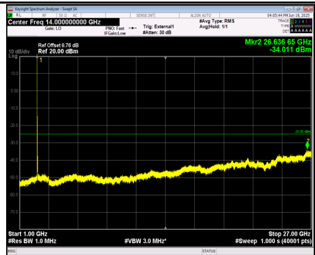
38-38-20MHz-20MHz-QPSK-QPSK-37952-38150-1RB#99- 0RB#0-1000~27000MHz-PASS
