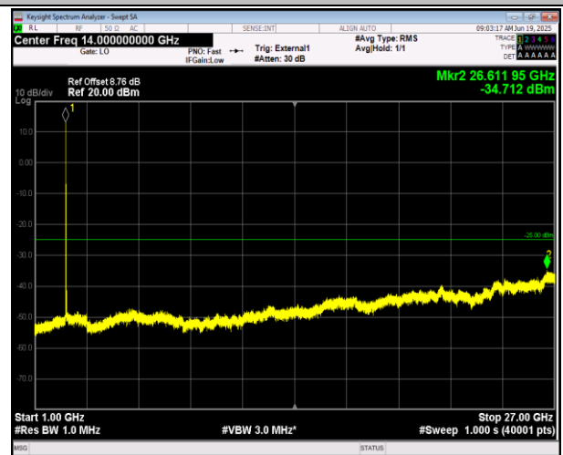
41(2555-2655)-41(2555-2655)-5MHz-20MHz-QPSK-QPSK- 40273-40390-1RB#24-0RB#0-1000~27000MHz-PASS
