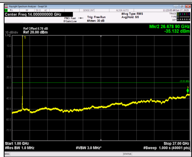
7-7-20MHz-10MHz-QPSK-QPSK-21251-21395-100RB#0-5 ORB#0-1000~27000MHz-PASS
