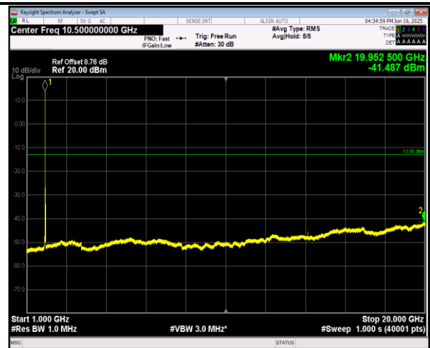
2-2-20MHz-20MHz-QPSK-QPSK-18902-19100-1RB#99-0R B#0-1000~20000MHz-PASS
