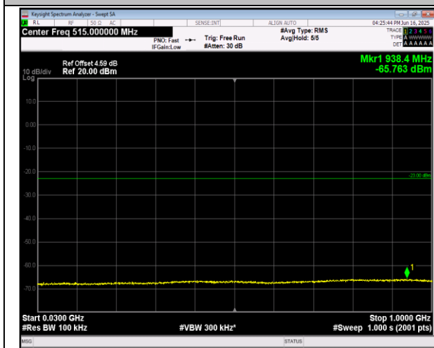
2-2-20MHz-20MHz-16QAM-16QAM-18700-18898-1RB#0-0RB#0-30~1000MHz-PASS
