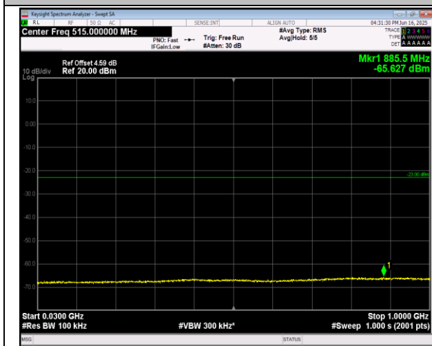
2-2-20MHz-20MHz-QPSK-QPSK-18902-19100-1RB#0-0 RB#0-30~1000MHz-PASS
