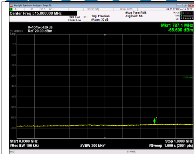
2-2-20MHz-20MHz-16QAM-16QAM-18700-18898-1RB#9 9-0RB#0-30~1000MHz-PASS
