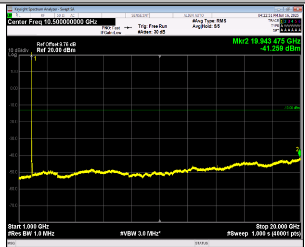
2-2-20MHz-20MHz-16QAM-16QAM-18700-18898-1RB#0-1RB#99-1000~20000MHz-PASS
