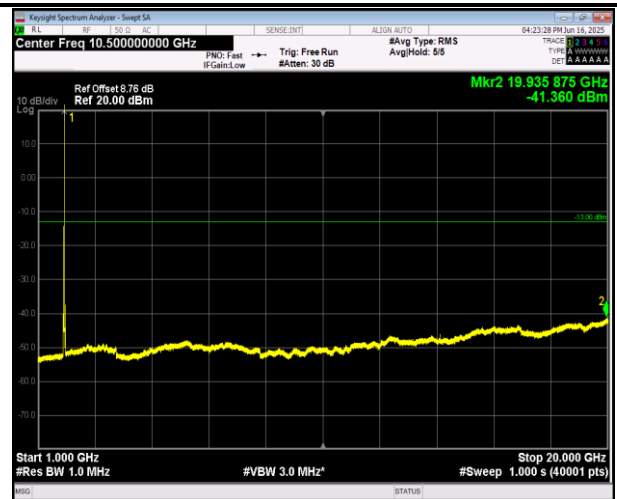
2-2-20MHz-20MHz-QPSK-QPSK-18700-18898-100RB#0-100RB#0-1000~20000MHz-PASS
