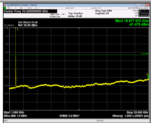
2-2-20MHz-20MHz-16QAM-16QAM-18801-18999-1RB#0-1 RB#99-1000~20000MHz-PASS
