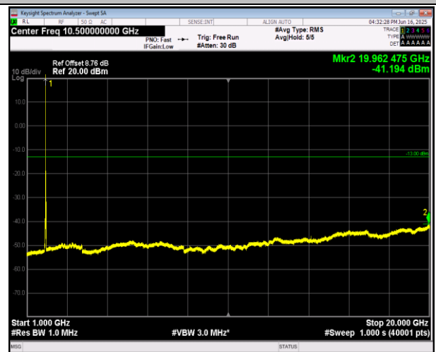
2-2-20MHz-20MHz-QPSK-QPSK-18902-19100-1RB#0-1RB #99-1000~20000MHz-PASS
