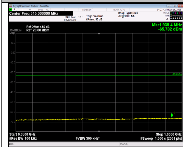
2-2-20MHz-20MHz-16QAM-16QAM-18801-18999-1RB#0 -1RB#99-30~1000MHz-PASS
