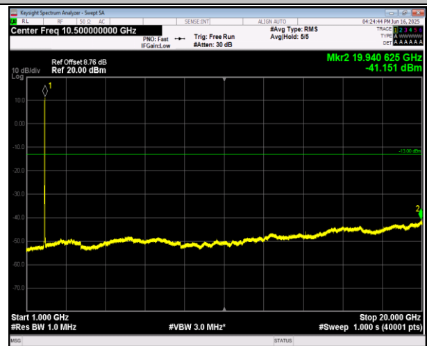
2-2-20MHz-20MHz-QPSK-QPSK-18700-18898-1RB#99-0RB B#0-1000~20000MHz-PASS
