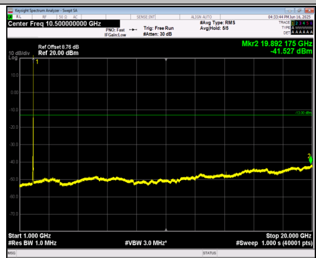
2-2-20MHz-20MHz-QPSK-QPSK-18902-19100-100RB#0-1 00RB#0-1000~20000MHz-PASS
