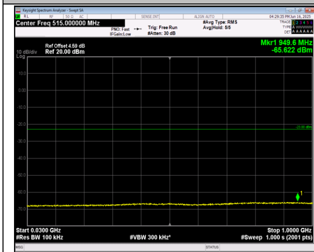
2-2-20MHz-20MHz-QPSK-QPSK-18801-18999-1RB#99-0 RB#0-30~1000MHz-PASS
