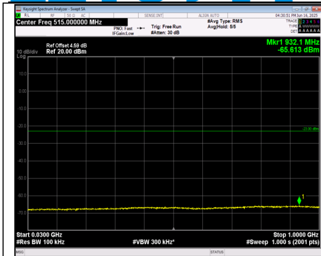
2-2-20MHz-20MHz-16QAM-16QAM-18801-18999-1RB#0 -0RB#0-30~1000MHz-PASS
