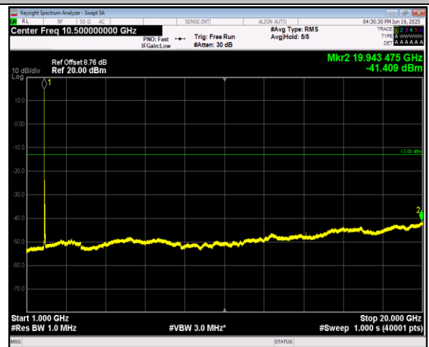
2-2-20MHz-20MHz-16QAM-16QAM-18801-18999-1RB#99- 0RB#0-1000~20000MHz-PASS
