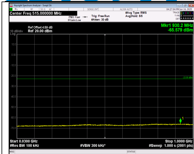
2-2-20MHz-20MHz-QPSK-QPSK-18801-18999-1RB#0-1 RB#99-30~1000MHz-PASS
