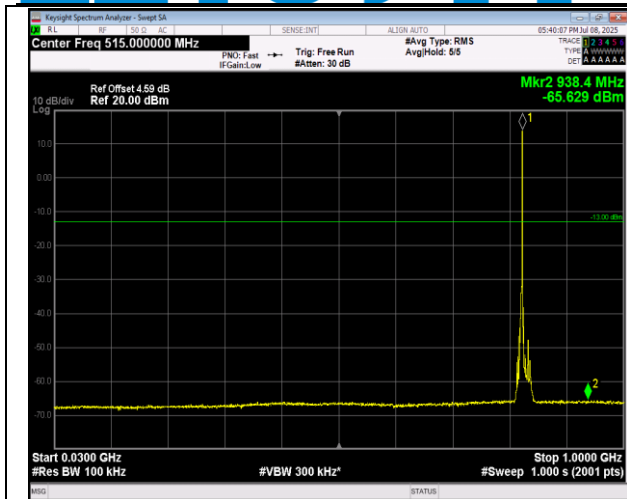
5-5-3MHz-5MHz-QPSK-QPSK-20416-20455-15RB#0-25 RB#0-30~1000MHz-PASS
