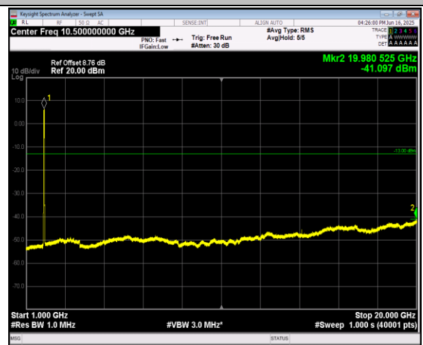
2-2-20MHz-20MHz-16QAM-16QAM-18700-18898-1RB#0-0RB#0-1000~20000MHz-PASS
