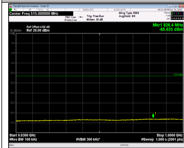
2-2-20MHz-20MHz-QPSK-QPSK-18700-18898-1RB#0-1 RB#99-30~1000MHz-PASS
