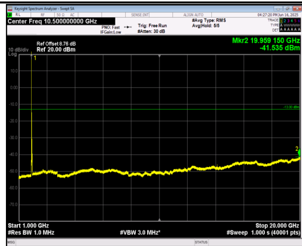
2-2-20MHz-20MHz-QPSK-QPSK-18801-18999-1RB#0-1RB #99-1000~20000MHz-PASS
