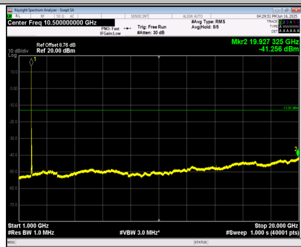
2-2-20MHz-20MHz-QPSK-QPSK-18801-18999-1RB#99-0R B#0-1000~20000MHz-PASS
