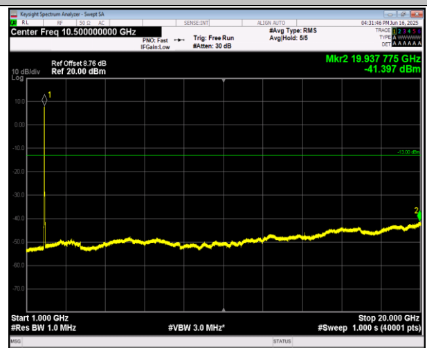
2-2-20MHz-20MHz-QPSK-QPSK-18902-19100-1RB#0-0RB #0-1000~20000MHz-PASS
