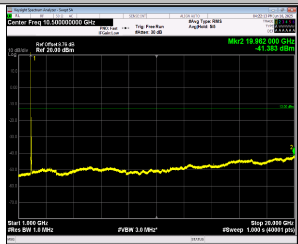
2-2-20MHz-20MHz-QPSK-QPSK-18700-18898-1RB#0-1RB #99-1000~20000MHz-PASS
