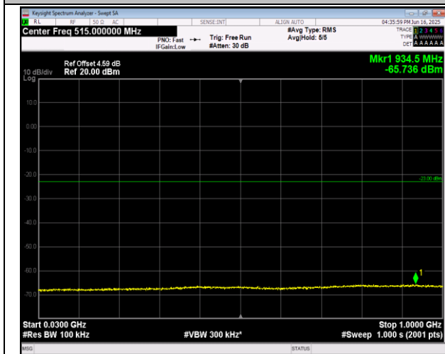
2-2-20MHz-20MHz-16QAM-16QAM-18902-19100-1RB#0- -0RB#0-30~1000MHz-PASS
