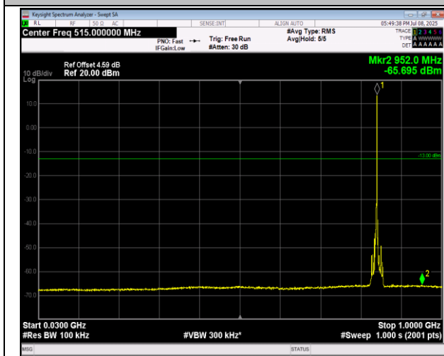
5-5-3MHz-5MHz-QPSK-QPSK-20586-20625-15RB#0-25 RB#0-30~1000MHz-PASS
