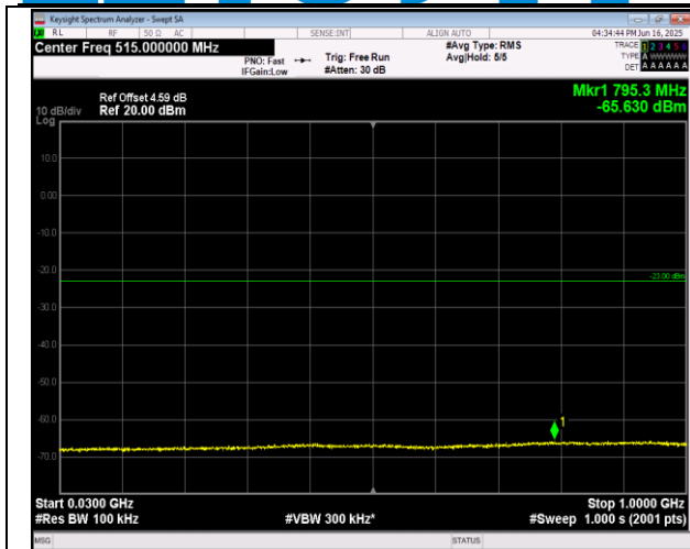
2-2-20MHz-20MHz-QPSK-QPSK-18902-19100-1RB#99-0 RB#0-30~1000MHz-PASS
