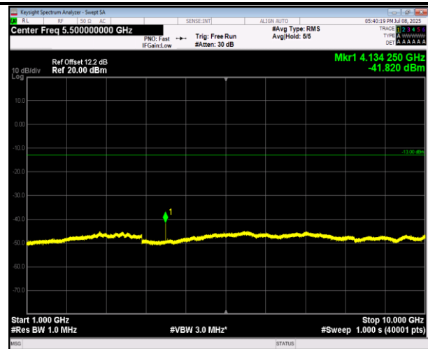
5-5-3MHz-5MHz-QPSK-QPSK-20416-20455-15RB#0-25RB #0-1000~10000MHz-PASS
