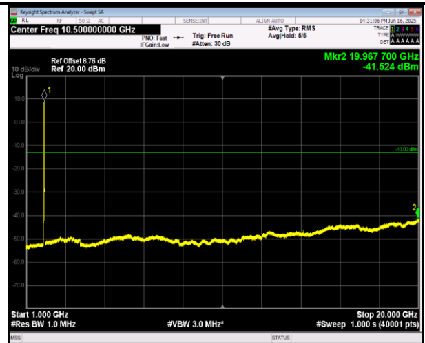
2-2-20MHz-20MHz-16QAM-16QAM-18801-18999-1RB#0-0 RB#0-1000~20000MHz-PASS
