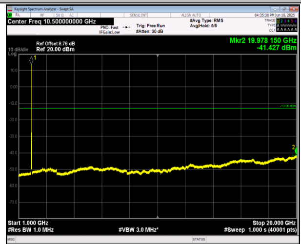
2-2-20MHz-20MHz-16QAM-16QAM-18902-19100-1RB#99- 0RB#0-1000~20000MHz-PASS
