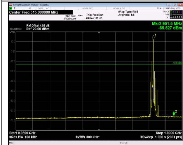
5-5-3MHz-5MHz-QPSK-QPSK-20416-20455-1RB#14-0R B#0-30~1000MHz-PASS
