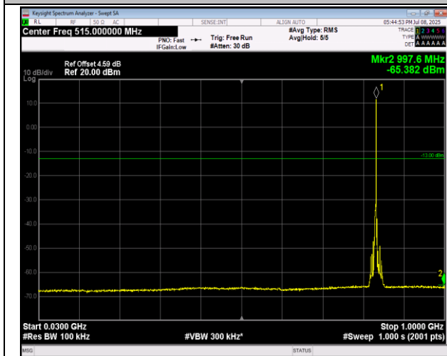
5-5-3MHz-5MHz-QPSK-QPSK-20501-20540-15RB#0-25 RB#0-30~1000MHz-PASS
