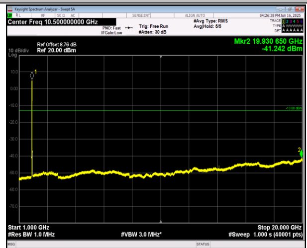
2-2-20MHz-20MHz-QPSK-QPSK-18801-18999-1RB#0-0RB #0-1000~20000MHz-PASS
