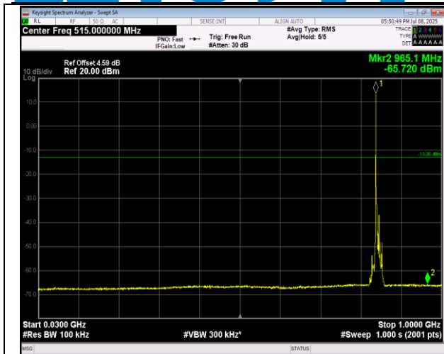
5-5-3MHz-5MHz-QPSK-QPSK-20586-20625-1RB#14-0R B#0-30~1000MHz-PASS
