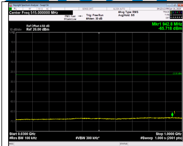
2-2-20MHz-20MHz-QPSK-QPSK-18700-18898-100RB#0-100RB#0-30~1000MHz-PASS
