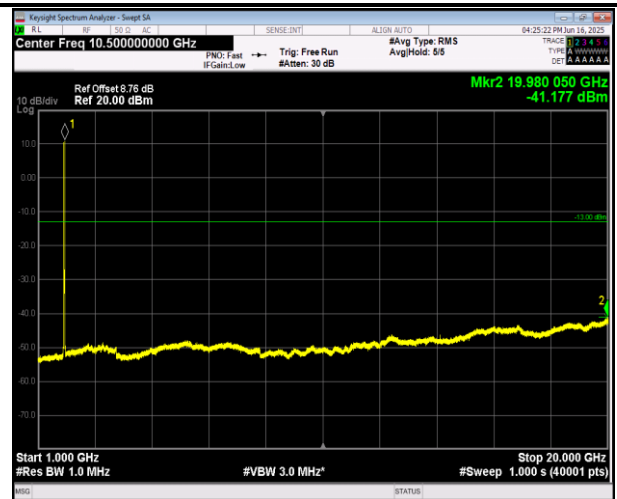
2-2-20MHz-20MHz-16QAM-16QAM-18700-18898-1RB#99- 0RB#0-1000~20000MHz-PASS
