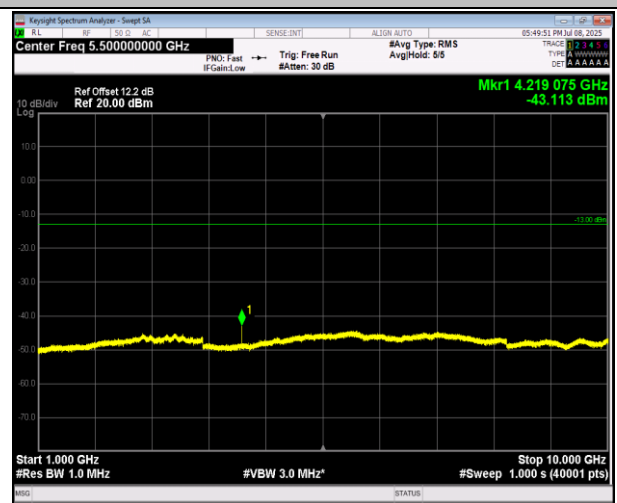
5-5-3MHz-5MHz-QPSK-QPSK-20586-20625-15RB#0-25RB #0-1000~10000MHz-PASS
