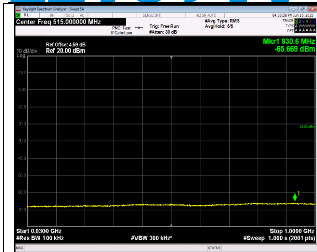
5-5-3MHz-5MHz-QPSK-QPSK-20416-20455-1RB#0-0RB #0-30~1000MHz-PASS
