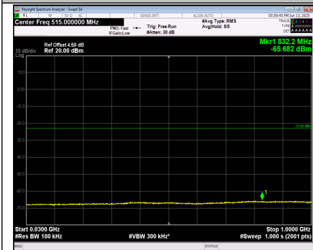
2-2-5MHz-20MHz-QPSK-QPSK-18808-18925-1RB#0-0R B#0-30~1000MHz-PASS
