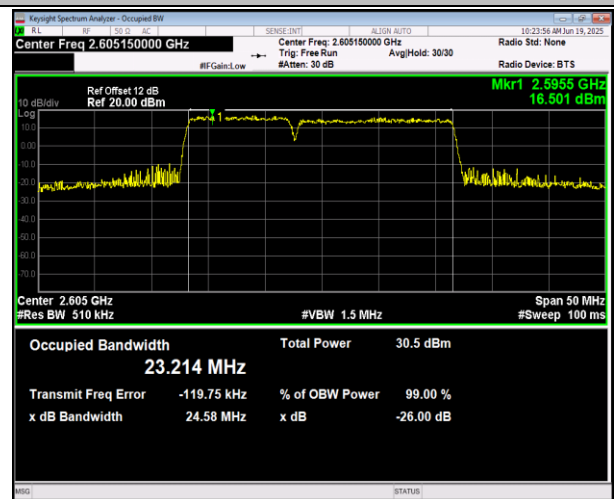
41(2555-2655)-41(2555-2655)-10MHz-15MHz-16QAM-16Q AM-41045-41165-50RB#0-75RB#0-PASS
