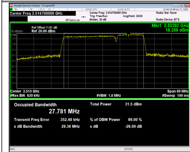
7-7-20MHz-10MHz-QPSK-QPSK-21051-21195-100RB#0-50RB#0-PASS
