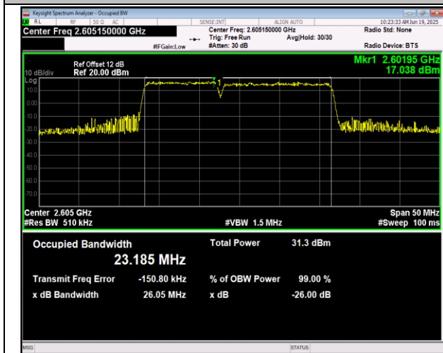
41(2555-2655)-41(2555-2655)-10MHz-15MHz-QPSK-QP SK-41045-41165-50RB#0-75RB#0-PASS
