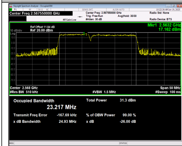
41(2555-2655)-41(2555-2655)-10MHz-15MHz-QPSK-QP SK-40669-40789-50RB#0-75RB#0-PASS
