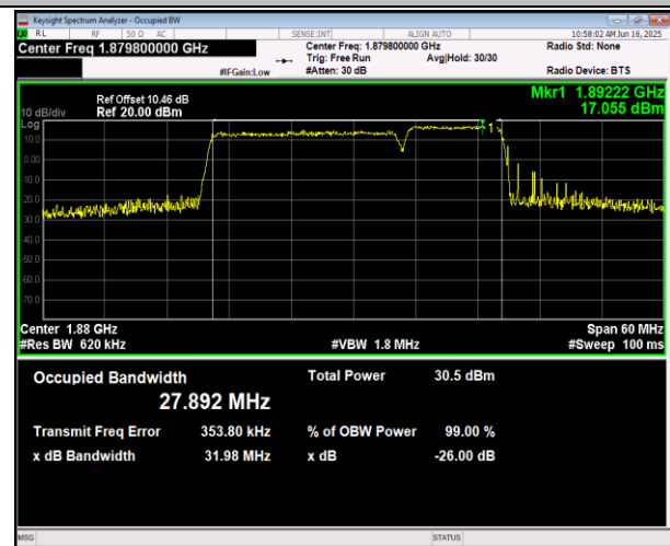
2-2-20MHz-10MHz-16QAM-16QAM-19001-19145-100RB#0-50RB#0-PASS
