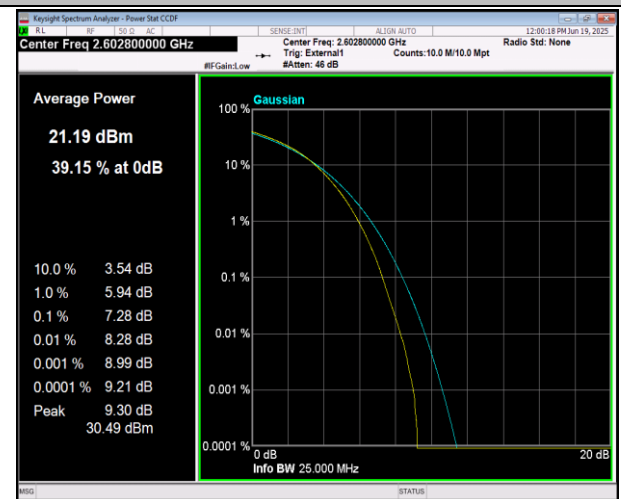
41(2555-2655)-41(2555-2655)-10MHz-20MHz-16QAM-16 QAM-40996-41140-50RB#0-100RB#0-PASS
