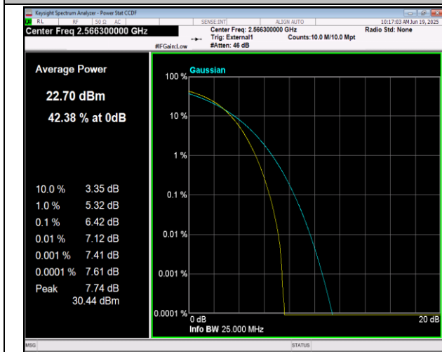
41(2555-2655)-41(2555-2655)-10MHz-15MHz-QPSK-QPS K-40669-40789-50RB#0-75RB#0-PASS
