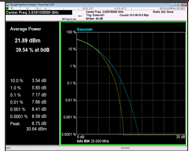
41(2555-2655)-41(2555-2655)-10MHz-15MHz-16QAM-16 QAM-40293-40413-50RB#0-75RB#0-PASS
