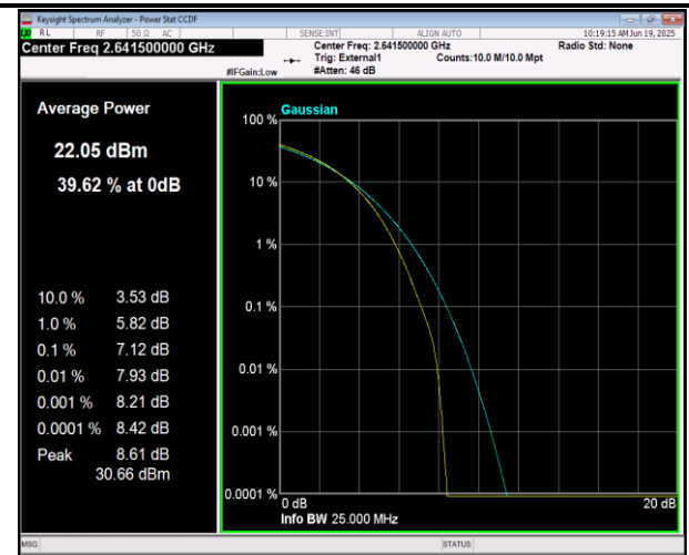
41(2555-2655)-41(2555-2655)-10MHz-20MHz-16QAM-16 QAM-40295-40439-50RB#0-100RB#0-PASS
