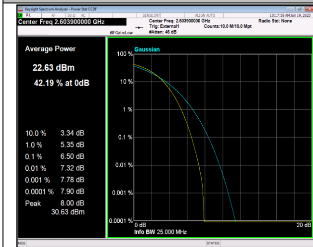
41(2555-2655)-41(2555-2655)-10MHz-15MHz-QPSK-QPS K-41045-41165-50RB#0-75RB#0-PASS
