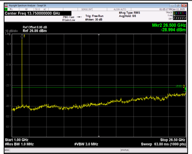
Band7-5MHz-QPSK-20775-1RB#0-Range2:1000~26500MHz
