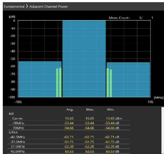
70MHz_30kHz_3665MHz-OFDM QPSK_RB90@45 -53.44,-54.66dB
