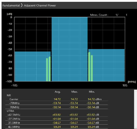
70MHz_30kHz_3665MHz-OFDM QPSK_RB1@188 -53.74,-50.14dB
