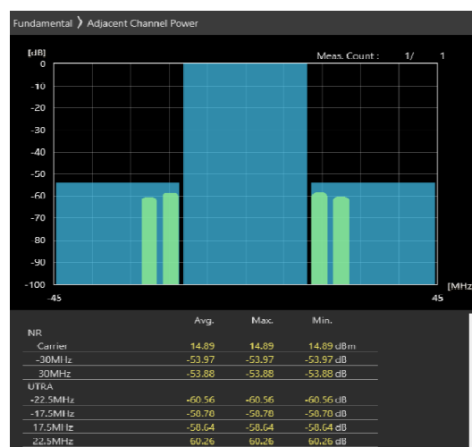
30MHz_30kHz_3685MHz-OFDM QPSK_RB75@0 -53.97,-53.88dB
