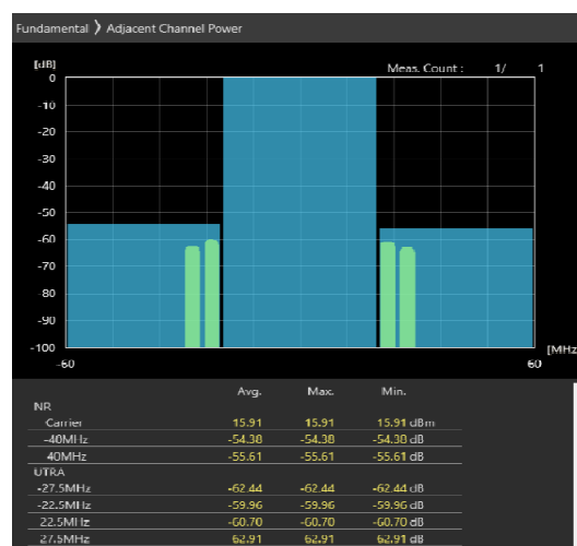
40MHz_30kHz_3680MHz-OFDM QPSK_RB50@25 -54.38,-55.61dB
