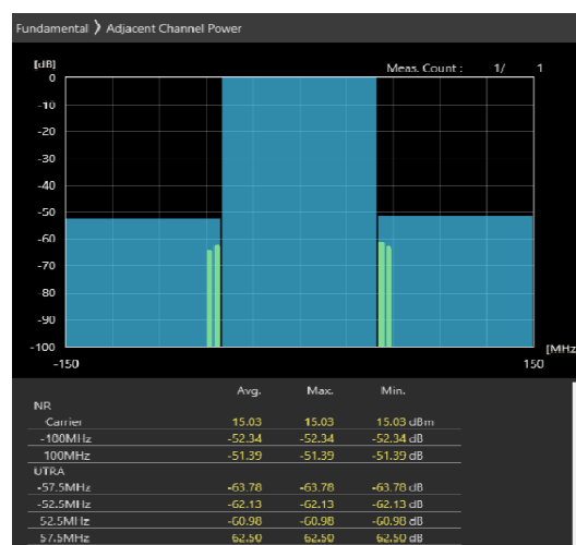
100MHz_30kHz_3650MHz-OFDM QPSK_RB270@0 -52.34,-51.39dB
