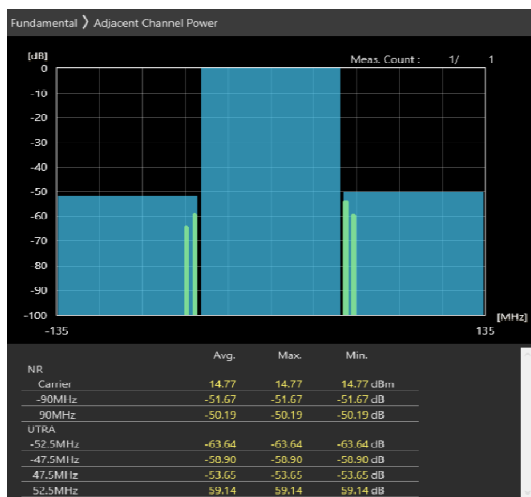
90MHz_30kHz_3655MHz-OFDM QPSK_RB1@244 -51.67,-50.19dB
