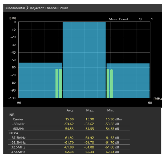
60MHz_30kHz_3670MHz-OFDM QPSK_RB81@40 -53.62,-54.53dB
