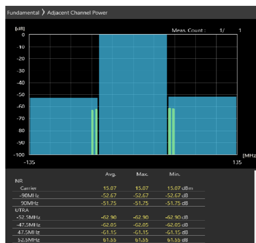
90MHz_30kHz_3655MHz-OFDM QPSK_RB243@0 -52.67,-51.75dB
