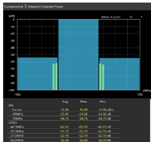
70MHz_30kHz_3665MHz-OFDM QPSK_RB90@45 -53.92,-54.75dB
