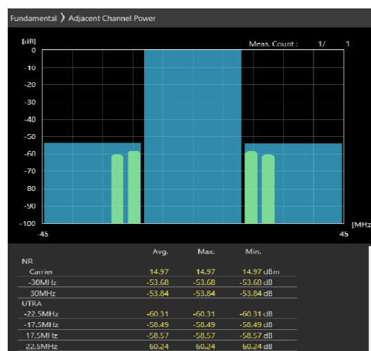
30MHz_30kHz_3685MHz-OFDM QPSK_RB75@0 -53.68,-53.84dB
