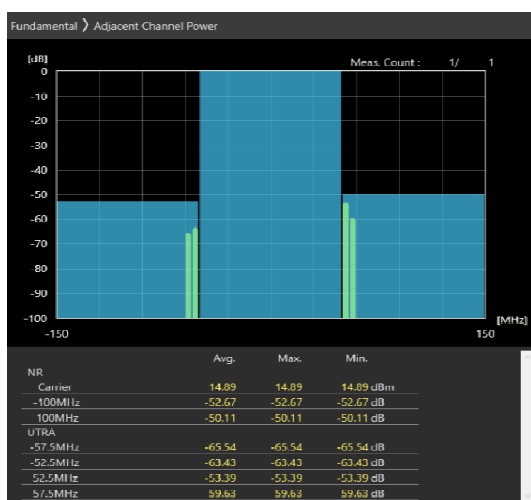
100MHz_30kHz_3650MHz-OFDM QPSK_RB1@272 -52.67,-50.11dB
