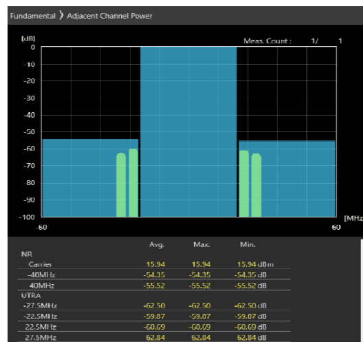
40MHz_30kHz_3680MHz-OFDM QPSK_RB50@25 -54.35,-55.52dB
