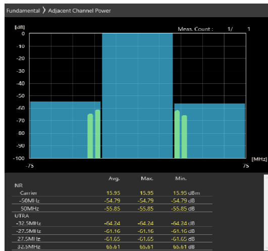
50MHz_30kHz_3675MHz-OFDM QPSK_RB64@32 -54.79,-55.85dB
