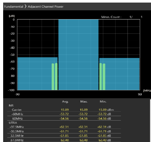
60MHz_30kHz_3670MHz-OFDM QPSK_RB81@40 -53.72,-54.56dB
