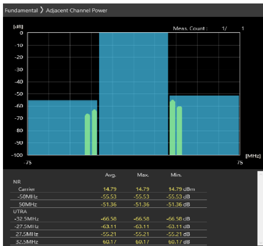
50MHz_30kHz_3675MHz-OFDM QPSK_RB1@132 -55.53,-51.36dB
