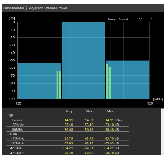
80MHz_30kHz_3660MHz-OFDM QPSK_RB1@216 -53.1,-50.48dB
