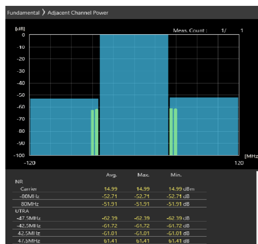
80MHz_30kHz_3660MHz-OFDM QPSK_RB216@0 -52.71,-51.91dB
