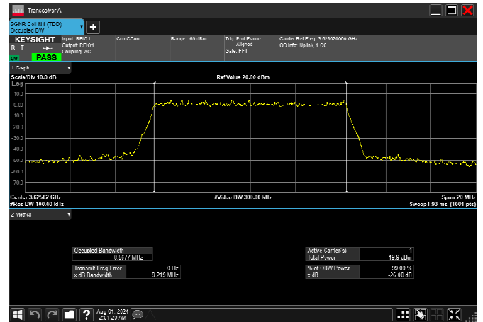
n77_2_15MHz_30kHz_3625MHz_DFT-s-OFDM \pi/2 BPSK_RB36@0 13.463MHz
