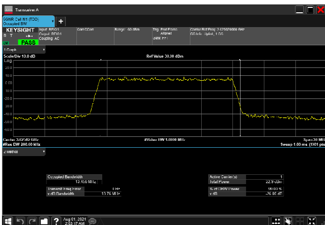
n77_2_15MHz_30kHz_3625MHz_DFT-s-OFDM QPSK_RB36@0 13.456MHz
