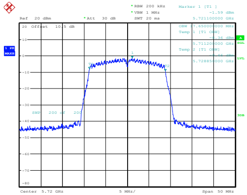
n20_5720MHz_Chain 0 17.650MHz
