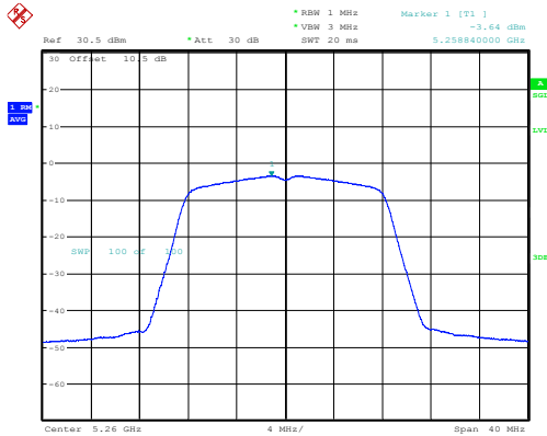
a_5260MHz_Chain 0 -3.64dBm/MHz
