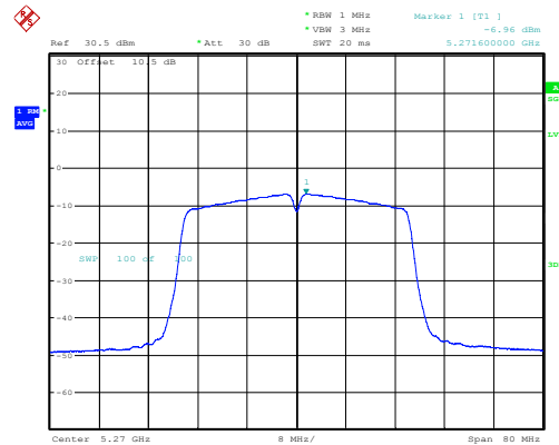
n40_5270MHz_Chain 0 -6.96dBm/MHz
