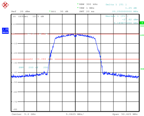
a_5200MHz_Chain 0 20.250MHz
