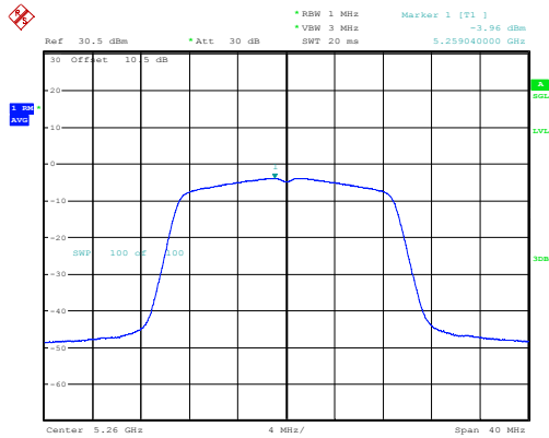
n20_5260MHz_Chain 0 -3.96dBm/MHz
