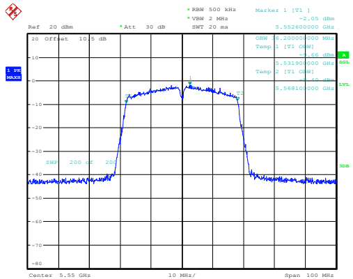
n40_5550MHz_Chain 0 36.200MHz
