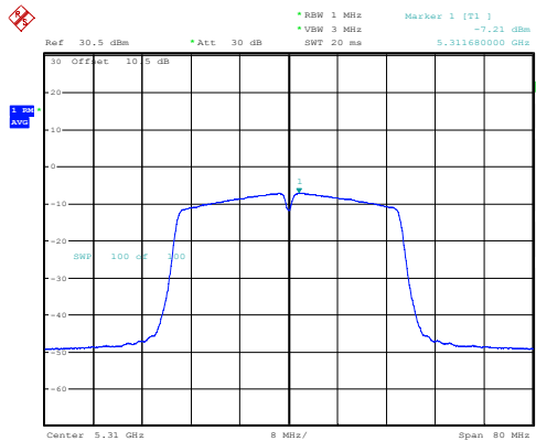
n40_5310MHz_Chain 0 -7.21dBm/MHz
