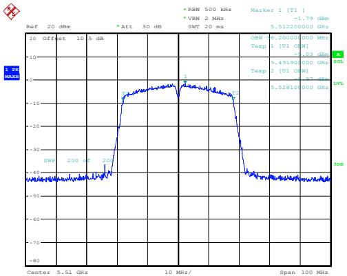
n40_5510MHz_Chain 0 36.200MHz
