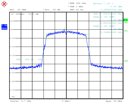
n20_5700MHz_Chain 0 17.650MHz
