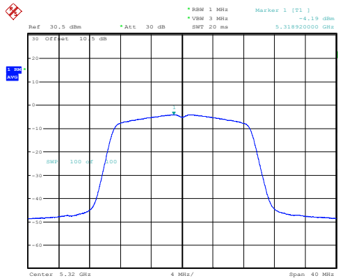
n20_5320MHz_Chain 0 -4.19dBm/MHz
