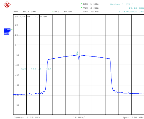
ac80_5290MHz_Chain 0 -10.12dBm/MHz
