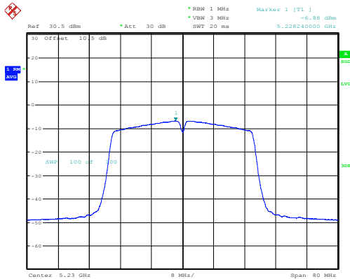
n40_5230MHz_Chain 0 -6.88dBm/MHz
