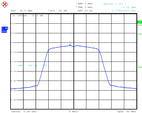
a_5280MHz_Chain 0 -3.24dBm/MHz
