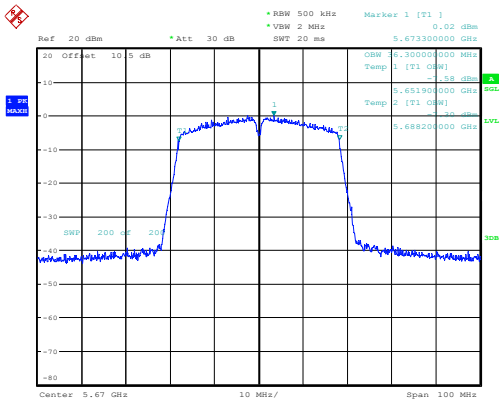
n40_5670MHz_Chain 0 36.300MHz
