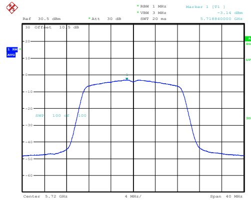
n20_5720MHz_Chain 0 -3.14dBm/MHz
