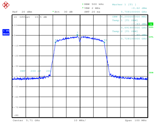
n40_5710MHz_Chain 0 36.200MHz
