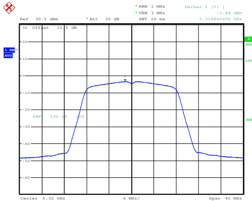
a_5320MHz_Chain 0 -3.48dBm/MHz
