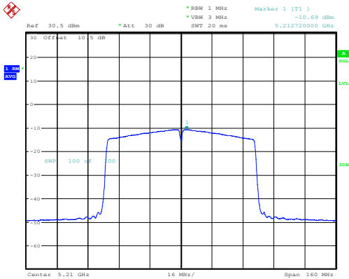
ac80_5210MHz_Chain 0 -10.69dBm/MHz
