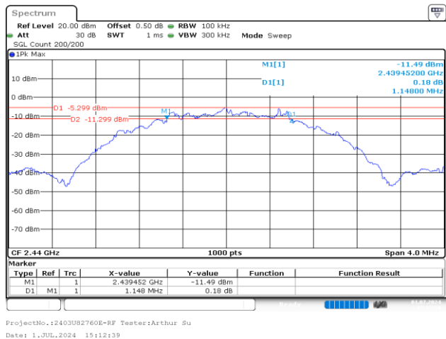
Middle 1.148MHz
