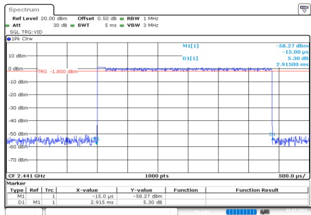
8DPSK_Hopping_3DH5 2.915ms
