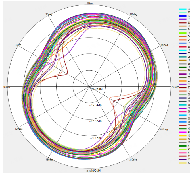
LTE B42 NR n77/n78 Phi=0deg
