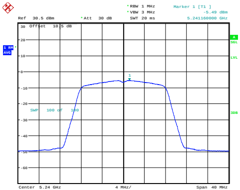
a_5240MHz -5.49dBm/MHz
