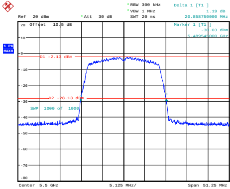
n20_5500MHz 20.859MHz
