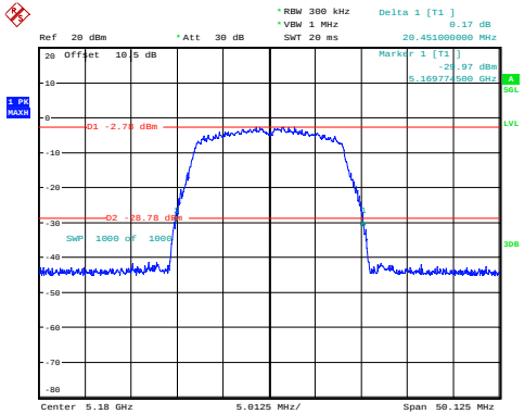
a_5180MHz 20.451MHz
