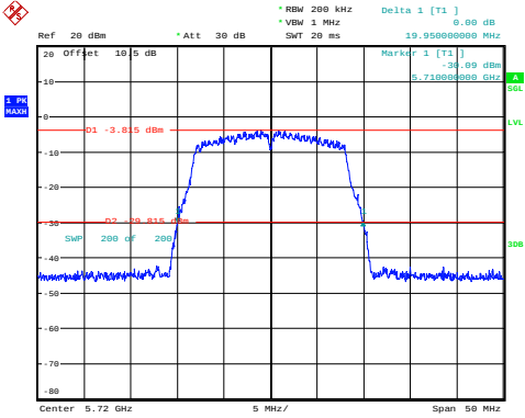
a_5720MHz 19.950MHz
