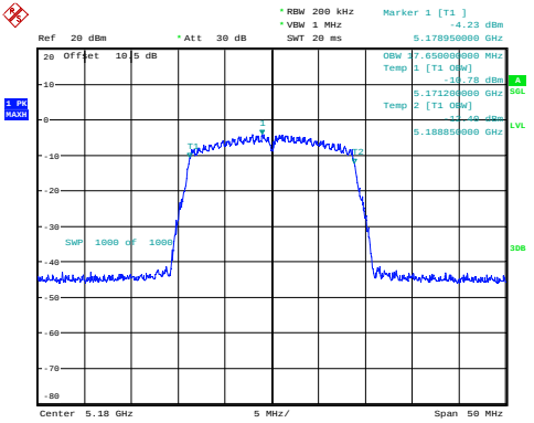
n20_5180MHz 17.650MHz
