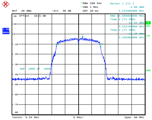
a_5240MHz 16.600MHz
