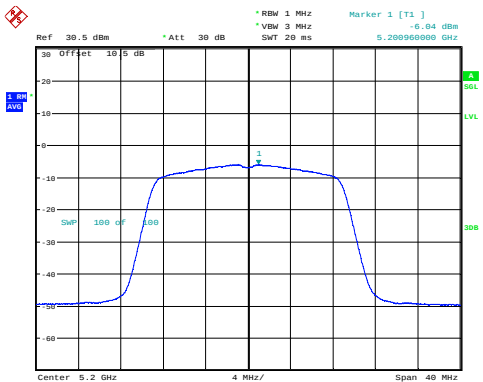
n20_5200MHz -6.04dBm/MHz
