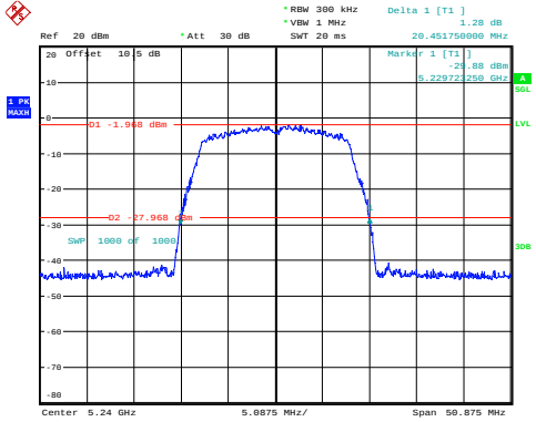
a_5240MHz 20.452MHz
