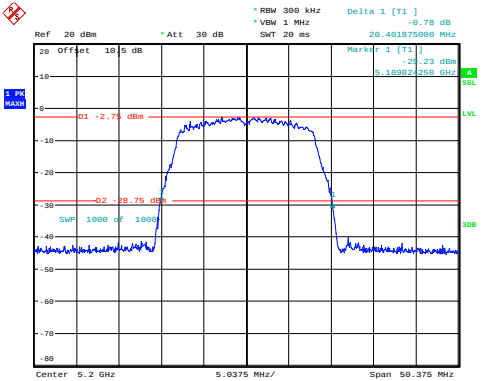
a_5200MHz 20.402MHz
