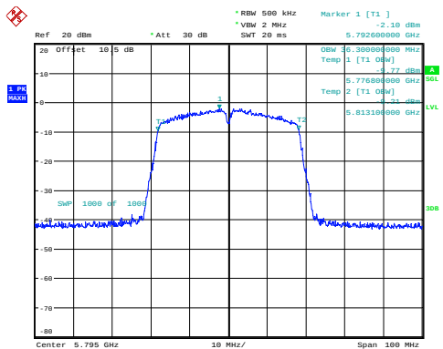
n40_5795MHz 36.300MHz
