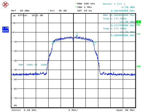
a_5180MHz 16.600MHz
