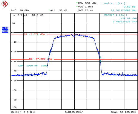
a_5500MHz 20.501MHz
