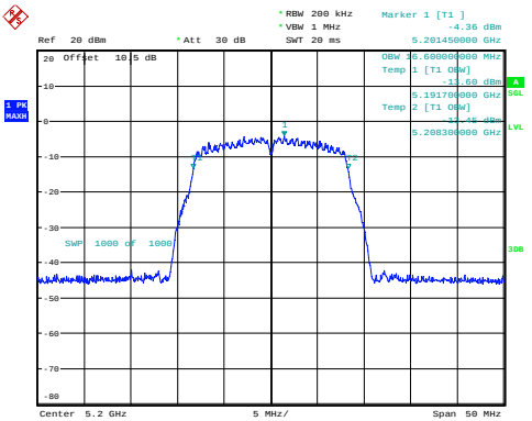
a_5200MHz 16.600MHz
