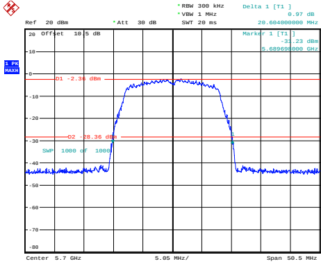
a_5700MHz 20.604MHz
