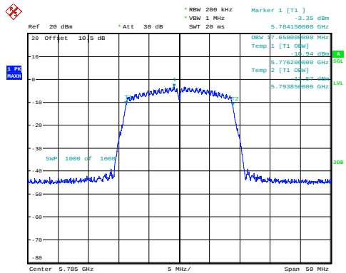
n20_5785MHz 17.650MHz
