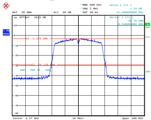
n40_5270MHz 41.400MHz
