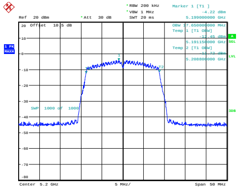
n20_5200MHz 17.650MHz
