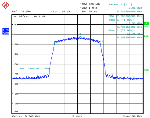
n20_5745MHz 17.700MHz
