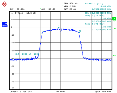
n40_5755MHz 36.300MHz
