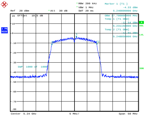
n20_5240MHz 17.700MHz
