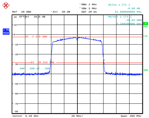
ac80_5290MHz 81.800MHz
