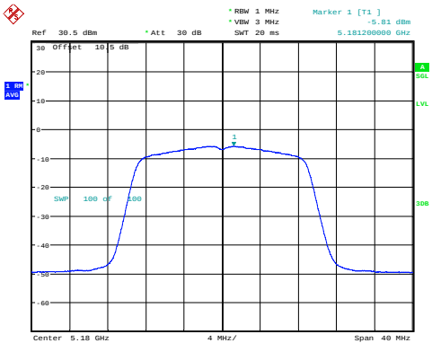
n20_5180MHz -5.81dBm/MHz
