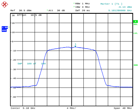
a_5180MHz -6.13dBm/MHz
