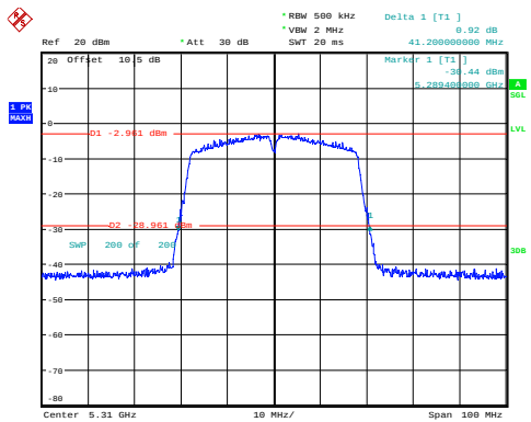
n40_5310MHz 41.200MHz
