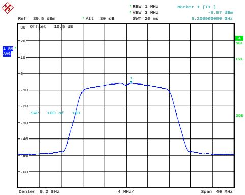
a_5200MHz -6.07dBm/MHz
