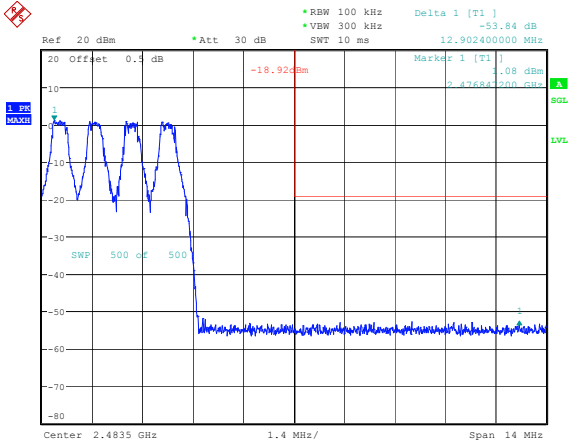
GFSK_Hopping_Upper 53.84dB
