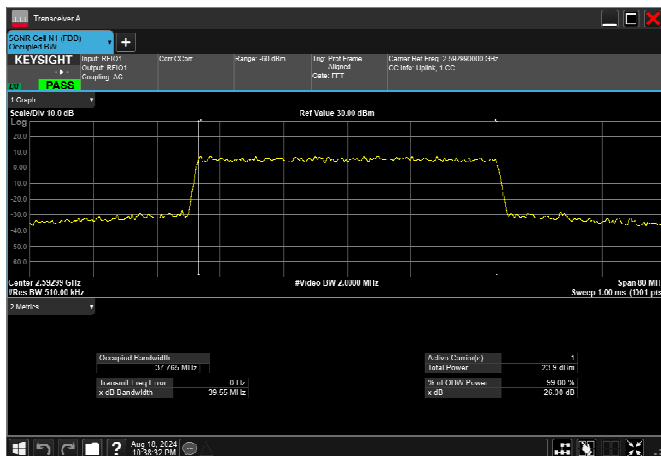
n41_50MHz_30kHz_2592.99MHz_DFT-s-OFDM QPSK_RB128@0 46.889MHz
