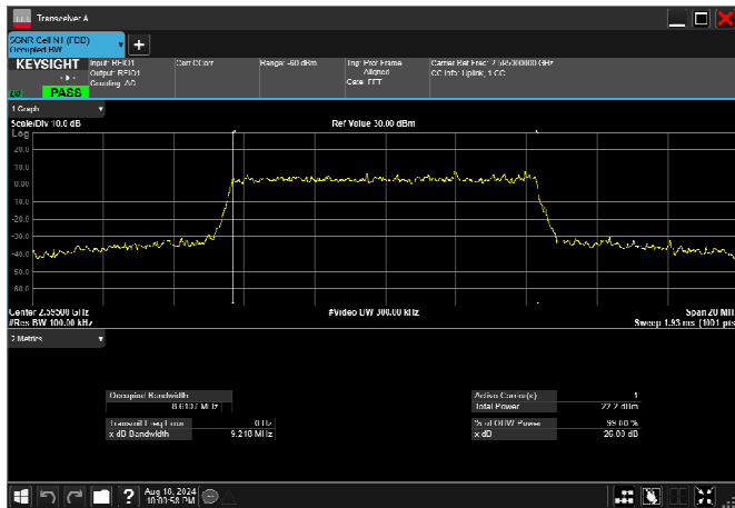
n38_15MHz_30kHz_2595MHz_DFT-s-OFDM QPSK_RB36@0 13.449MHz
