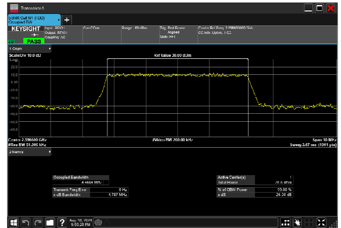
n38_5MHz_15kHz_2595MHz_DFT-s-OFDM 16 QAM_RB25@0 4.466MHz
