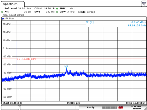
1_15MHz_Middle_QPSK_75@0
