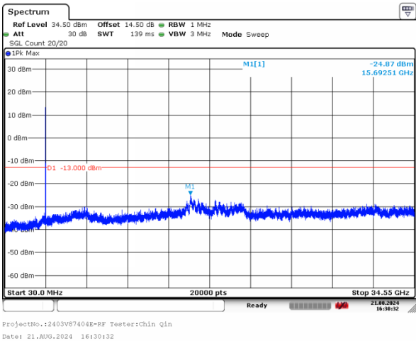
1_10MHz_Middle_QPSK_50@0
