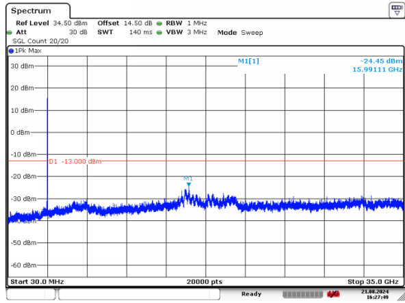
1_5MHz_Middle_QPSK_25@0
