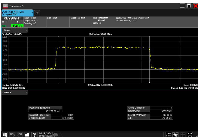
n78_2_90MHz_30kHz_3625MHz_DFT-s-OFDM 256 QAM_RB243@0 86.767MHz
