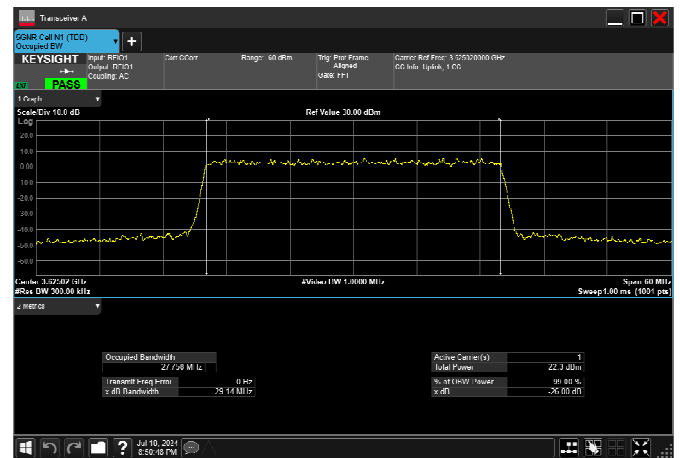
n77_2_30MHz_30kHz_3625MHz_CP-OFDM 256 QAM_RB78@0 27.758MHz
