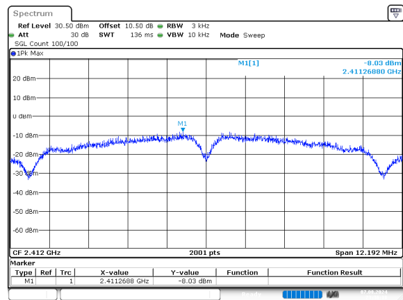
b_2412MHz_Chain 0
