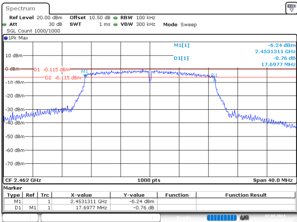
n20_2462MHz_Chain 0
