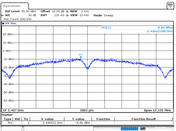
b_2437MHz_Chain 0
