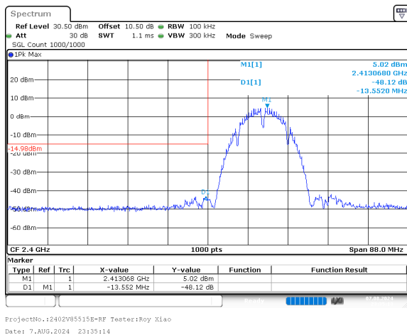
b_2412MHz_Chain 0
