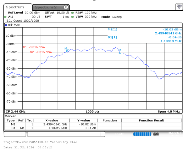
BLE 2Mbps Middle
