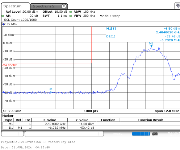
BLE 2Mbps Low
