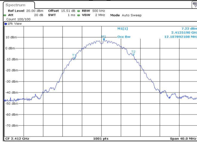
11B_Ant1_2412
