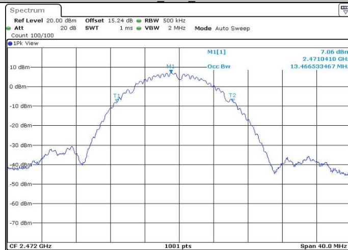
11B_Ant1_2472
