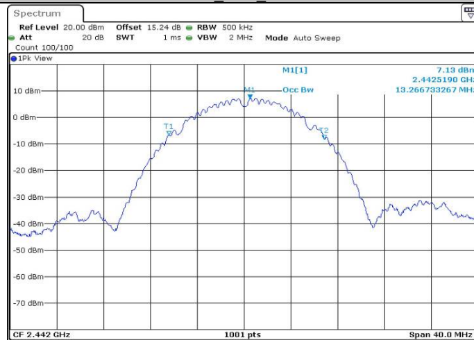
11B_Ant1_2442
