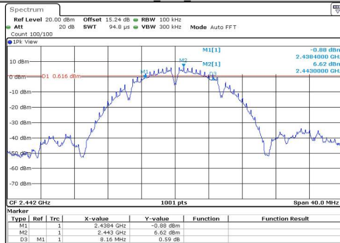
11B_Ant1_2442
