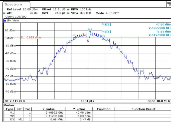
11B_Ant1_2412
