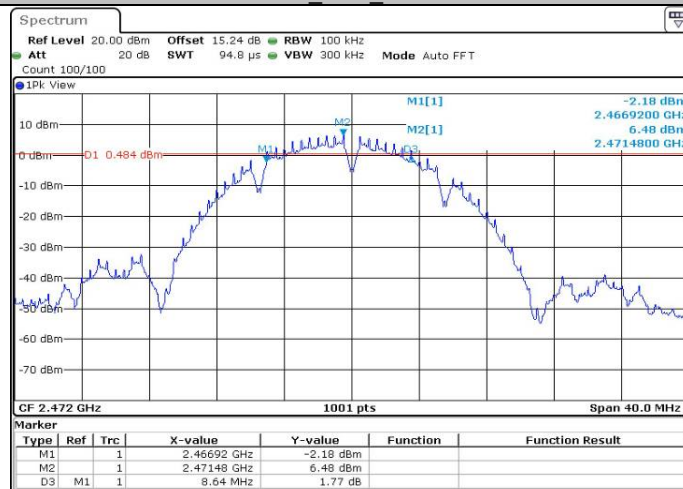
11B_Ant1_2472
