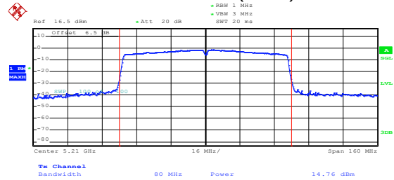
802.11ac(HT80)
