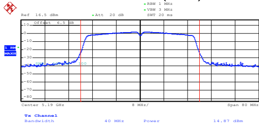
802.11ac(HT40)
