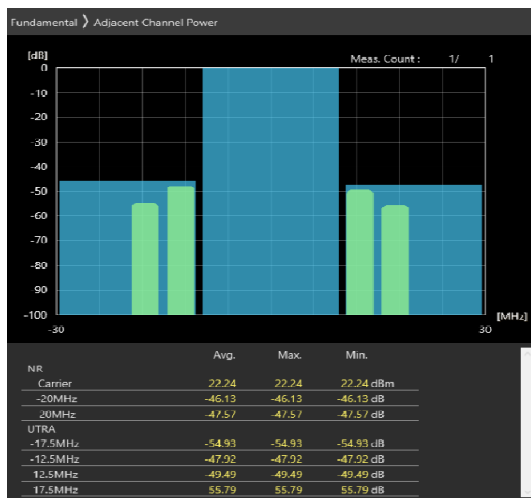
20MHz_30kHz_3690MHz-OFDM QPSK_RB25@12 -46.13,-47.57dB
