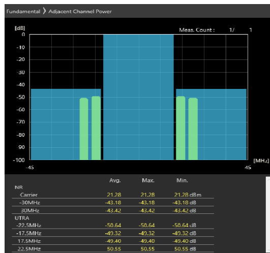
30MHz_30kHz_3685MHz-OFDM QPSK_RB75@0 -43.18,-43.42dB
