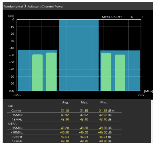
15MHz_30kHz_3692.5MHz-OFDM QPSK_RB36@0 -42.92,-43.4dB
