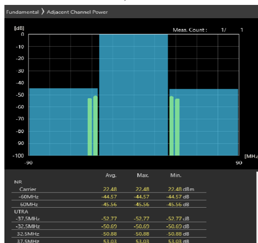
60MHz_30kHz_3670MHz-OFDM QPSK_RB81@40 -44.57,-45.56dB
