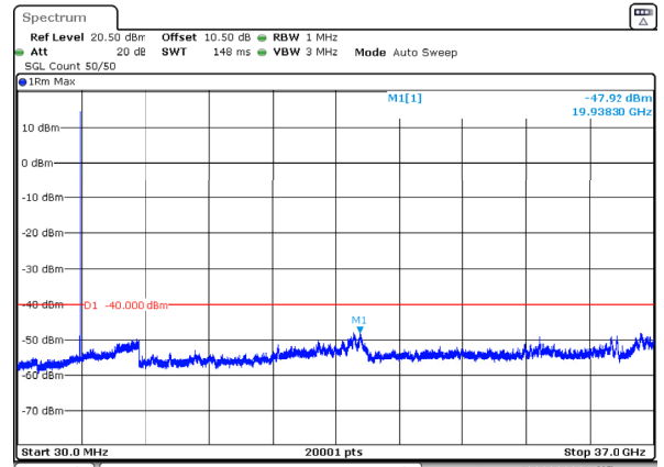
n77_2_15MHz_30kHz_3625MHz_DFT-s-OFDM QPSK_RB1@37 -47.92dBm
