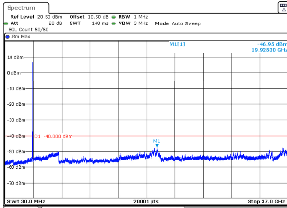
n77_2_15MHz_30kHz_3625MHz_DFT-s-OFDM QPSK_RB36@0 -46.95dBm
