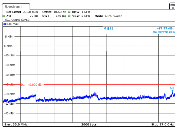
n77_2_15MHz_30kHz_3692.5MHz_DFT-s-OFDM QPSK_RB1@37 -47.77dBm
