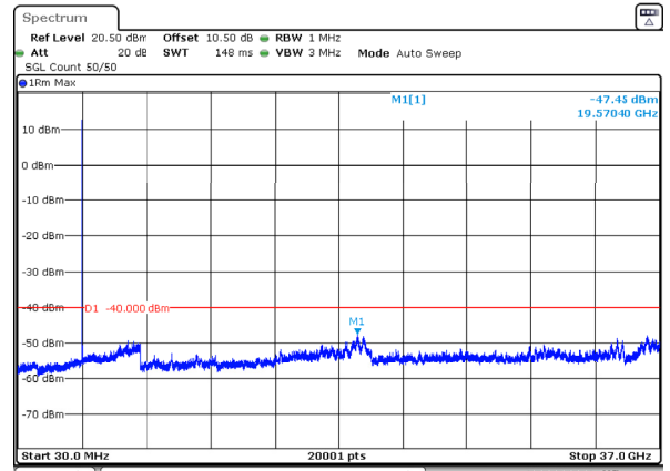
n77_2_15MHz_30kHz_3692.5MHz_DFT-s-OFDM QPSK_RB1@0 -47.45dBm
