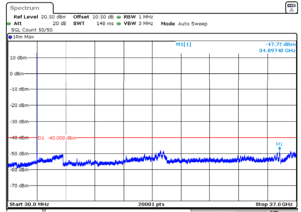
n77_2_10MHz_30kHz_3695MHz_DFT-s-OFDM QPSK_RB1@23 -47.72dBm
