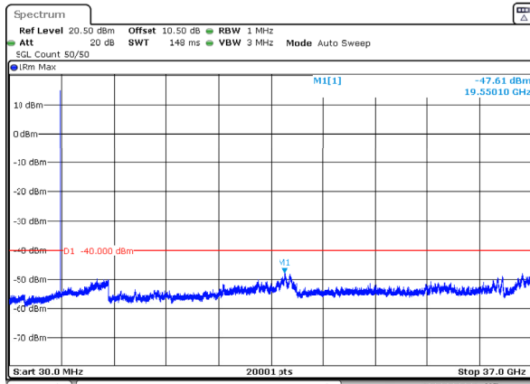
n77_2_15MHz_30kHz_3625MHz_DFT-s-OFDM QPSK_RB1@0 -47.61dBm
