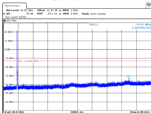
n71_10MHz_15kHz_668MHz_DFT-s-OFDM QPSK_RB50@0 -34.57dBm
