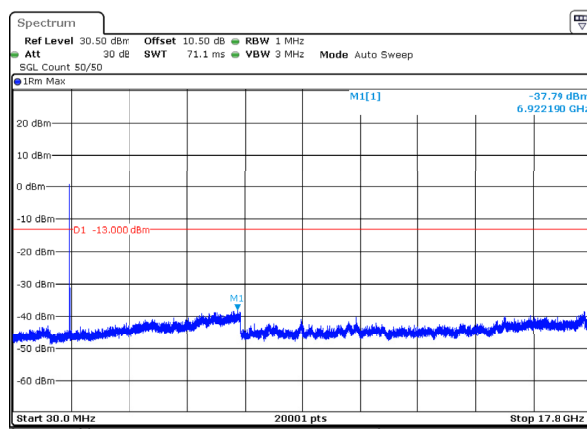
n66_40MHz_15kHz_1730MHz_DFT-s-OFDM QPSK_RB1@215 -37.79dBm
