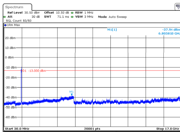
n66_40MHz_15kHz_1745MHz_DFT-s-OFDM QPSK_RB216@0 -37.94dBm
