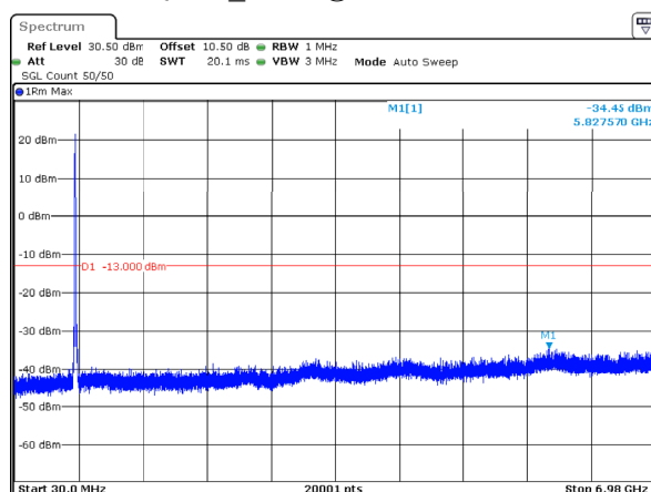
n71_10MHz_15kHz_680.5MHz_DFT-s-OFDM QPSK_RB50@0 -34.45dBm
