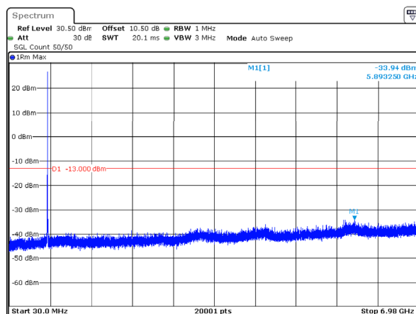
n71_10MHz_15kHz_668MHz_DFT-s-OFDM QPSK_RB1@51 -33.94dBm
