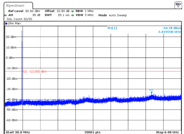
n71_5MHz_15kHz_695.5MHz_DFT-s-OFDM QPSK_RB1@0 -34.28dBm
