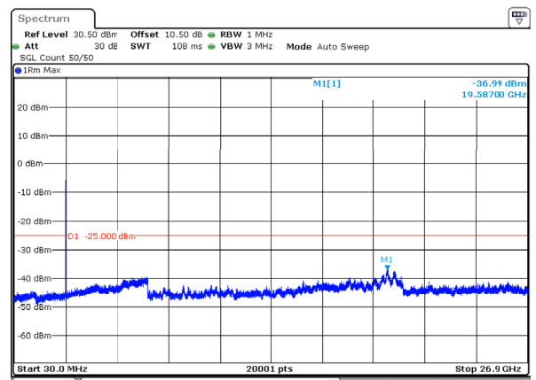
n41_15MHz_30kHz_2682.48MHz_DFT-s-OFDM QPSK_RB36@0 -36.99dBm
