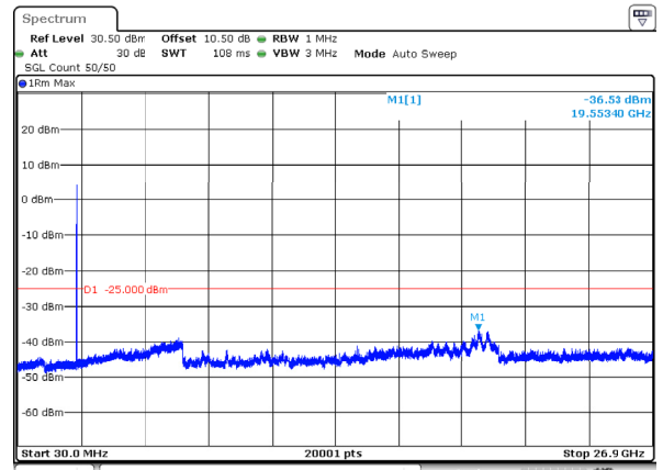
n41_30MHz_30kHz_2511MHz_DFT-s-OFDM QPSK_RB1@0 -36.53dBm
