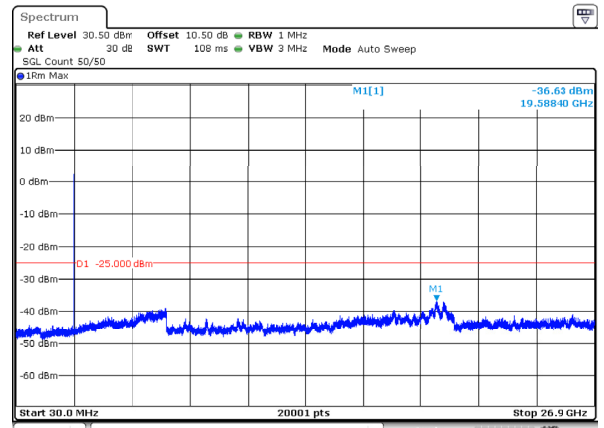
n41_15MHz_30kHz_2682.48MHz_DFT-s-OFDM QPSK_RB1@0 -36.63dBm
