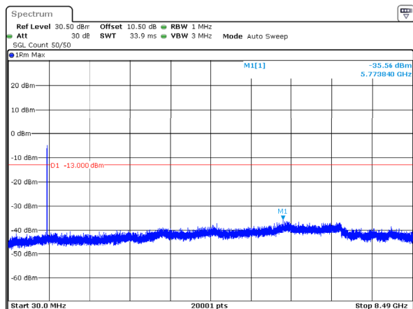
n5_10MHz_15kHz_829MHz_DFT-s-OFDM QPSK_RB50@0 -35.56dBm
