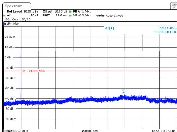
n5_10MHz_15kHz_829MHz_DFT-s-OFDM QPSK_RB1@0 -35.18dBm
