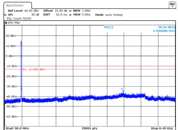
n5_20MHz_15kHz_834MHz_DFT-s-OFDM QPSK_RB100@0 -36.04dBm
