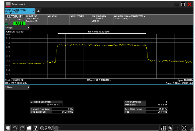
n77_3_100MHz_30kHz_3840MHz_DFT-s-OFDM QPSK_RB270@0
