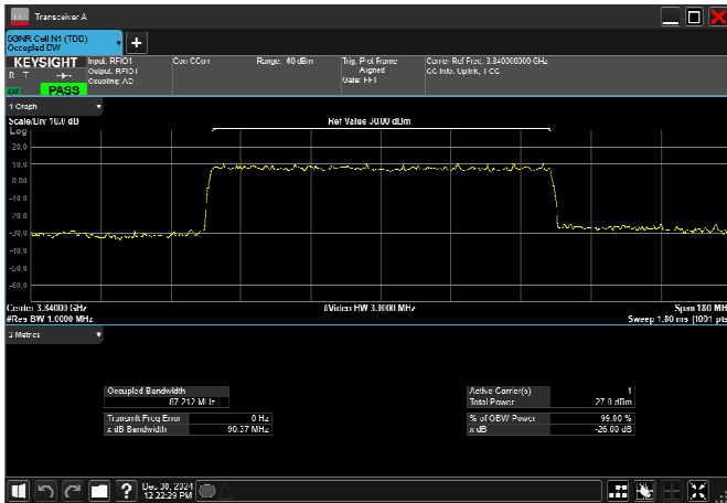
n77_3_100MHz_30kHz_3840MHz_DFT-s-OFDM \pi/2 BPSK_RB270@0
