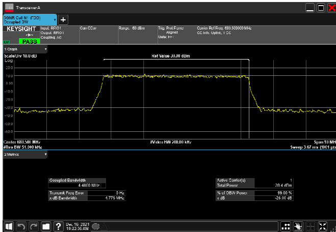
n71_5MHz_15kHz_680.5MHz_CP-OFDM QPSK_RB25@0
