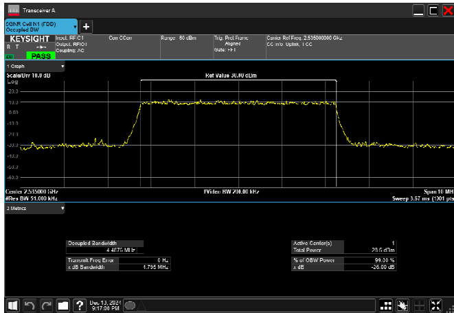
n7_5MHz_15kHz_2535MHz_CP-OFDM QPSK_RB25@0
