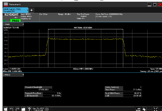
n41_80MHz_30kHz_2592.99MHz_DFT-s-OFDM \pi/2 BPSK RB216@0
