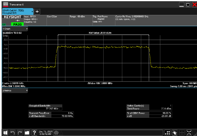
n41_80MHz_30kHz_2592.99MHz_CP-OFDM QPSK_RB217@0
