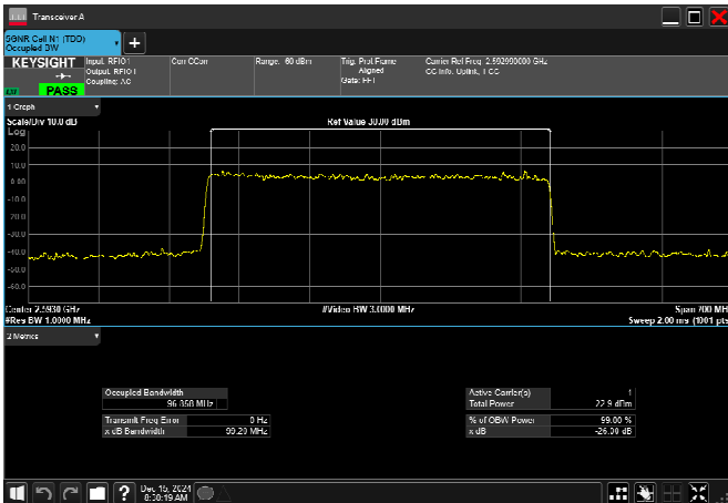
n41_100MHz_30kHz_2592.99MHz_CP-OFDM QPSK_RB273@0
