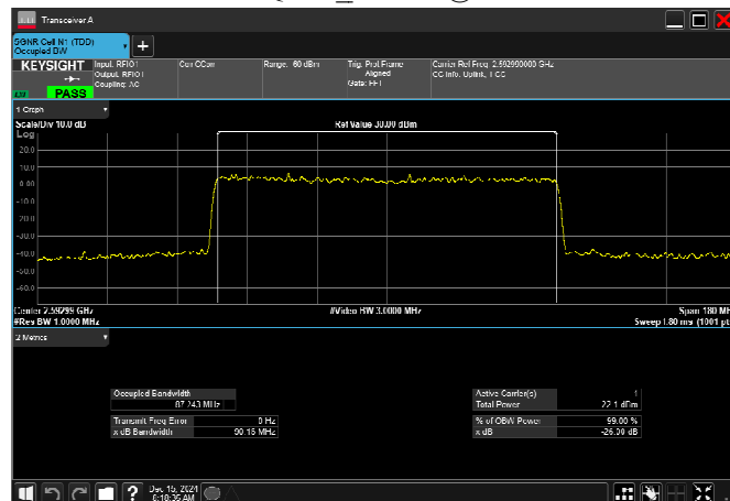
n41_100MHz_30kHz_2592.99MHz_DFT-s-OFDM \pi/2 BPSK RB270@0
